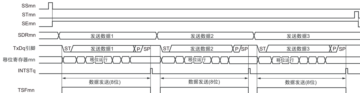
图 12-79 UART 发送（单次发送模式）的时序图
