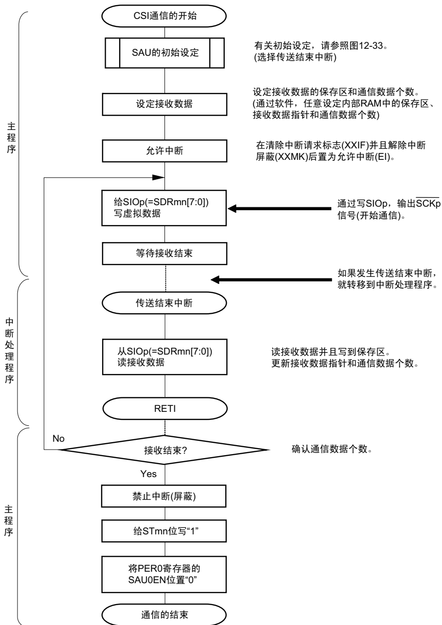
图 12-37 主控接收（单次接收模式）的流程图
