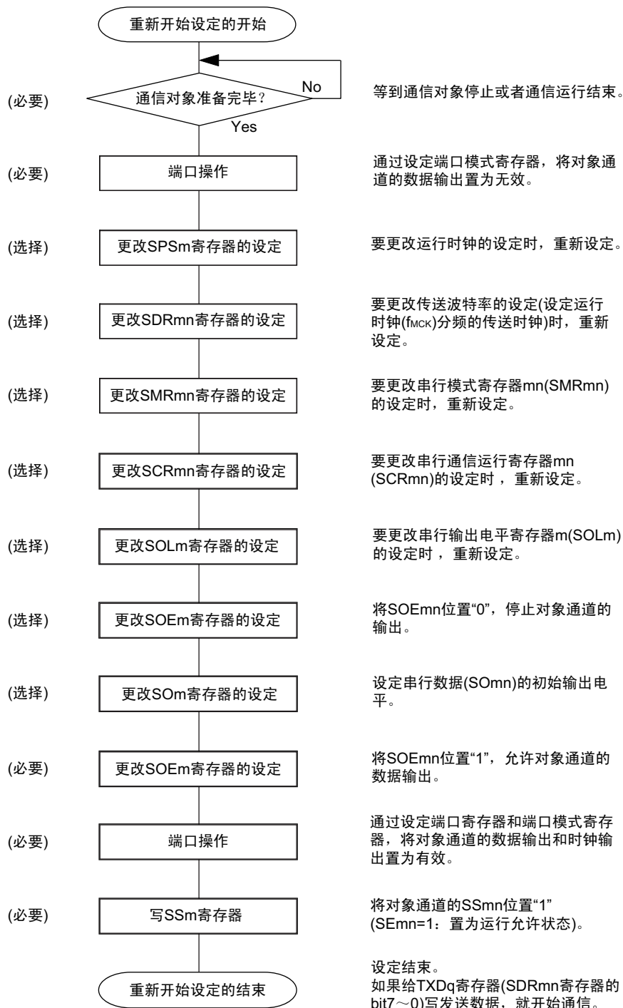
图 12-78 UART 发送的重新开始设定步骤
