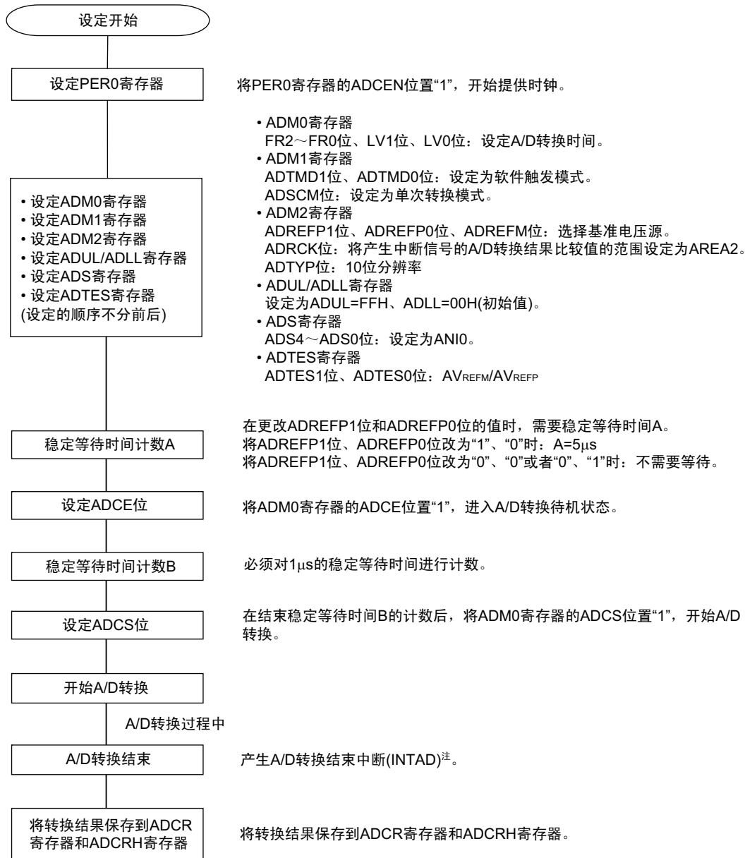
图 11-30 测试触发模式的设定
