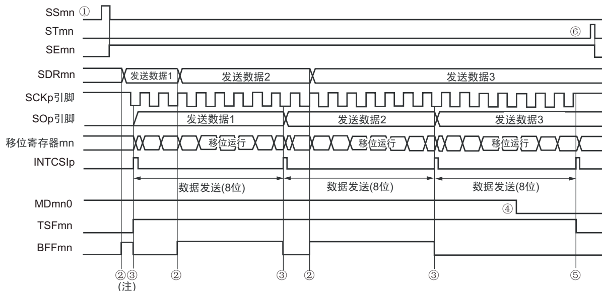
图 12-54 从属发送（连续发送模式）的时序图（类型 1：DAPmn=0、CKPmn=0）
