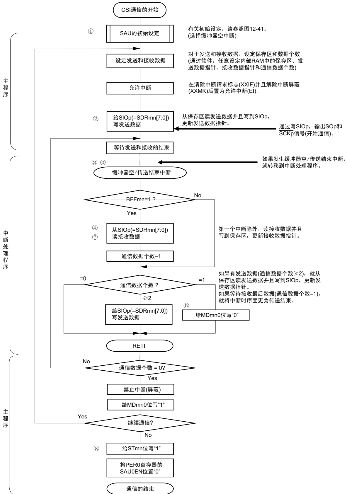
图 12-47 主控发送和接收（连续发送和接收模式）的流程图
