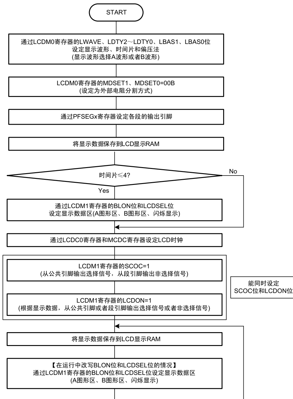
图 14-19 通常液晶波形时的外部电阻分割方式的设定步骤
