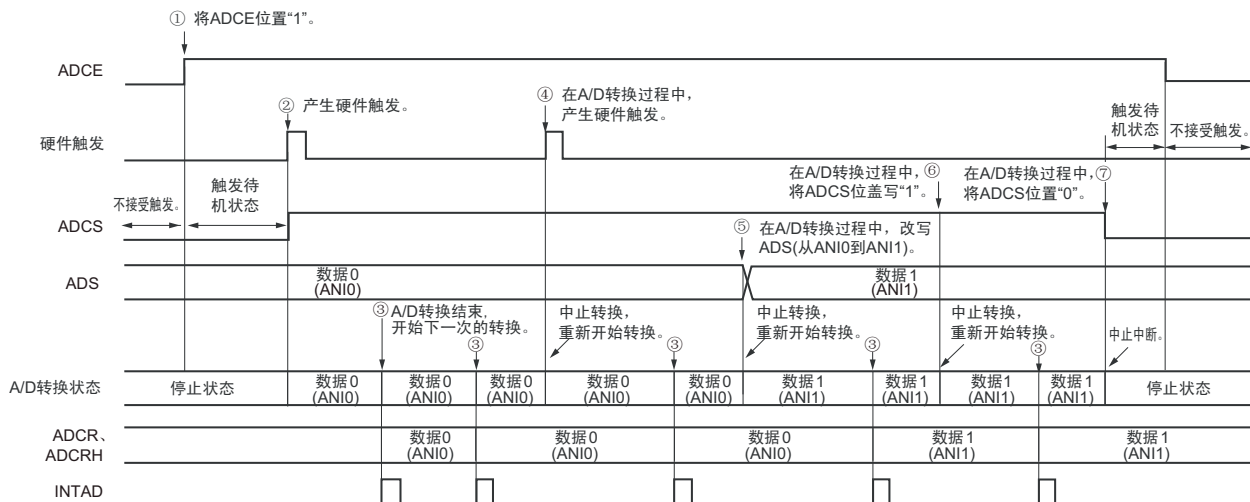
图 11-24 硬件触发等待模式（连续转换模式）的运行时序例子
