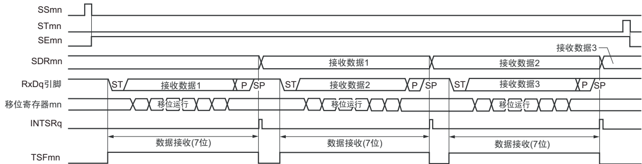
图 12-87 UART 接收的时序图
