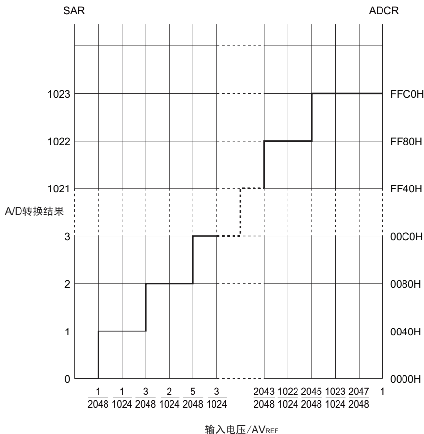
图 11-19 模拟输入电压和 A/D 转换结果的关系
