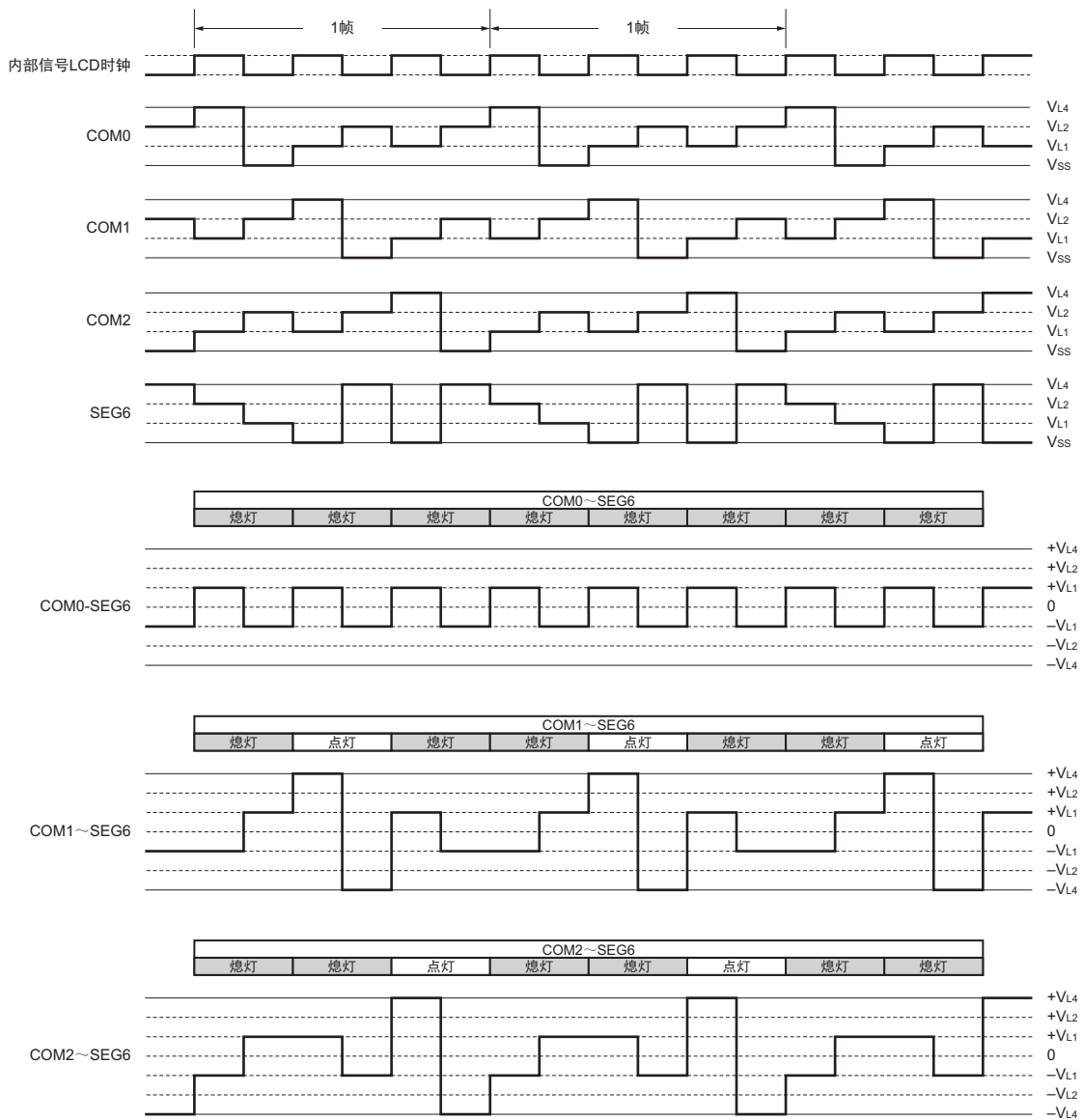
图 14-38 SEG6 和各公共信号之间的 3 个时间片的 LCD 驱动波形例子 (1/3 偏压法)
