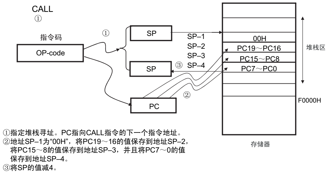
图 3-38 CALL、CALLT 的例子
