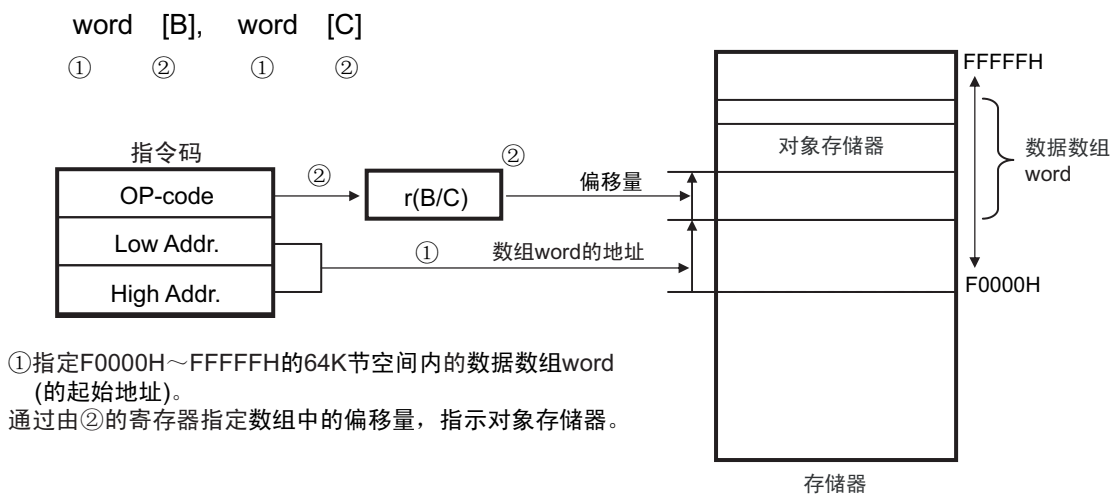
图 3-30 word[BC] 的例子
