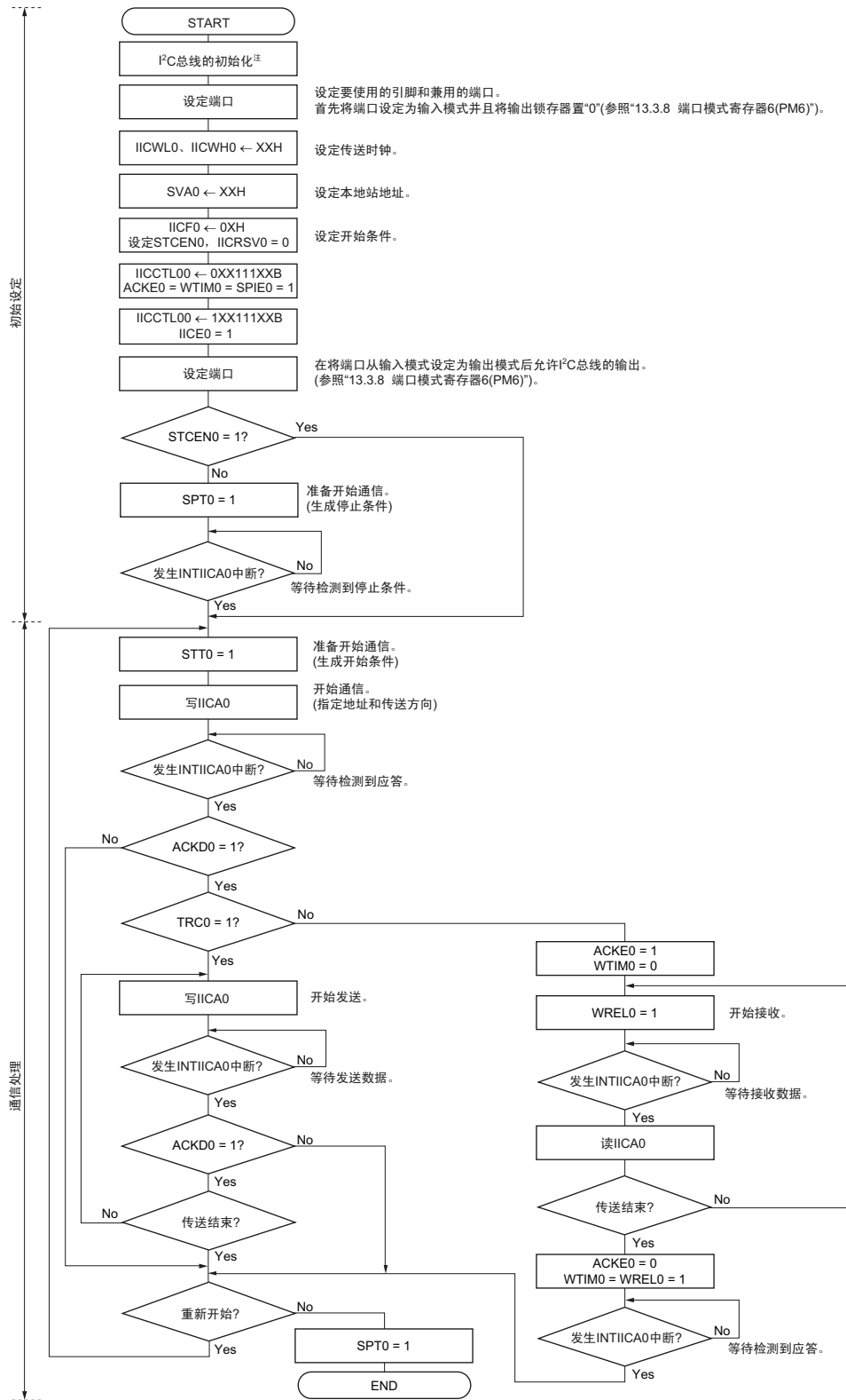
图 13-28 单主控系统的主控运行
