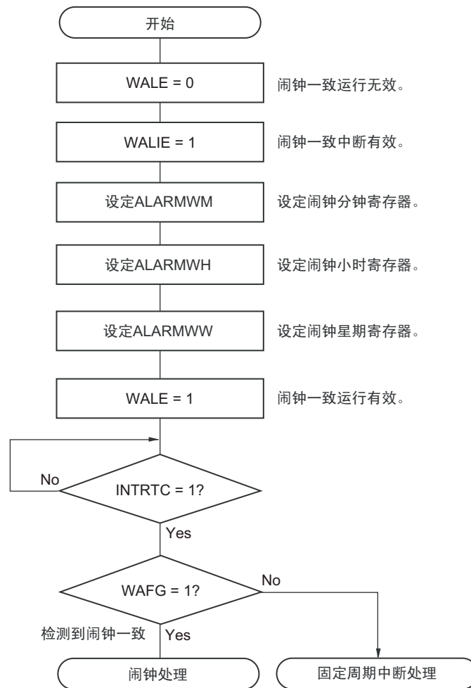
图 7-21 闹钟设定步骤
