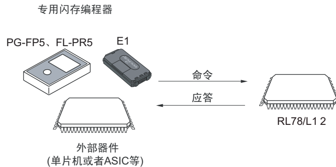
图 26-9 通信命令
