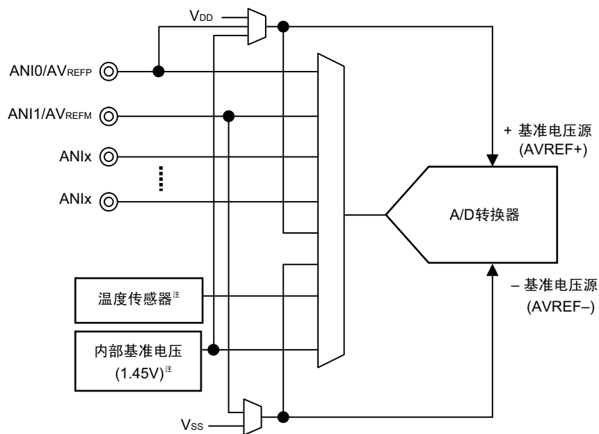
图 23-14 A/D 测试功能的结构
