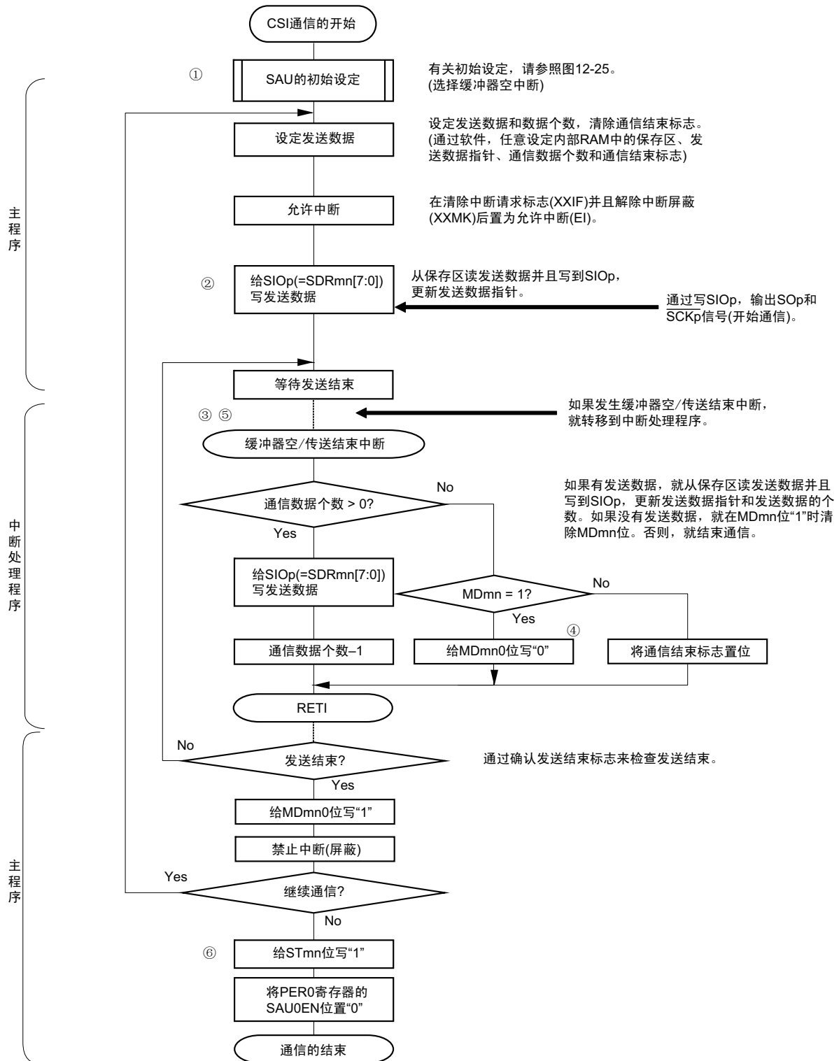
图 12-31 主控发送（连续发送模式）的流程图
