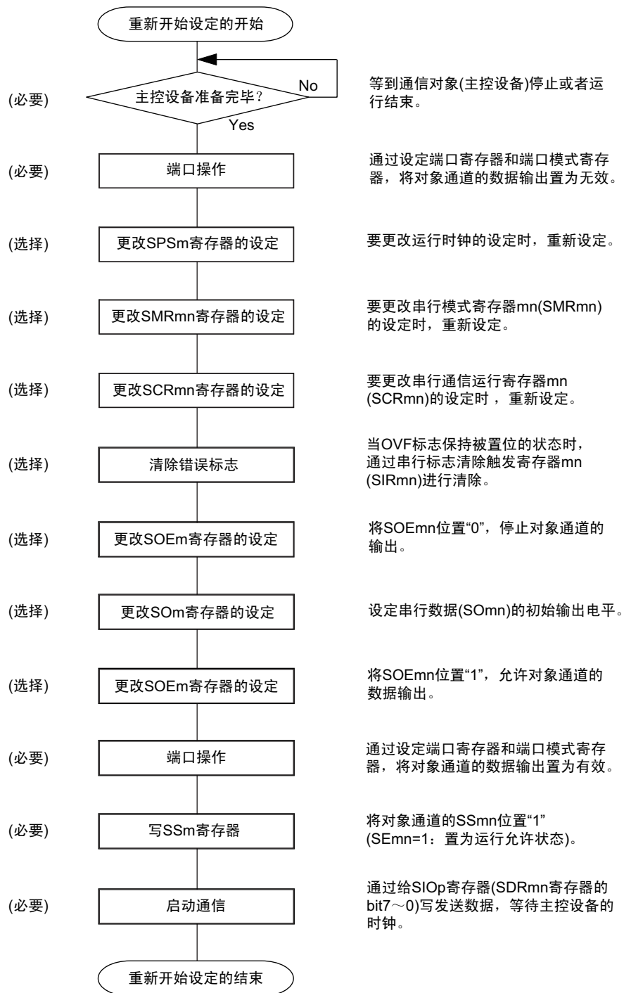
图 12-65 从属发送和接收的重新开始设定步骤
