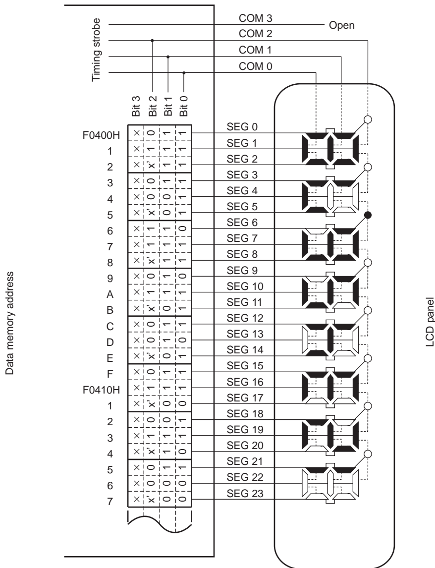
图 14-36 3 个时间片的 LCD 显示屏的连线例子
