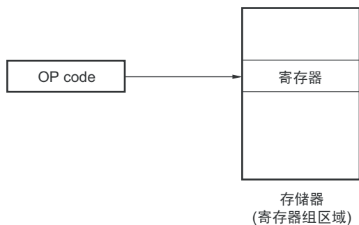
图 3-20 寄存器寻址的概要
