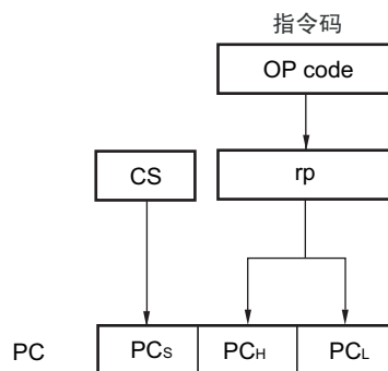
图 3-18 寄存器直接寻址的概要
