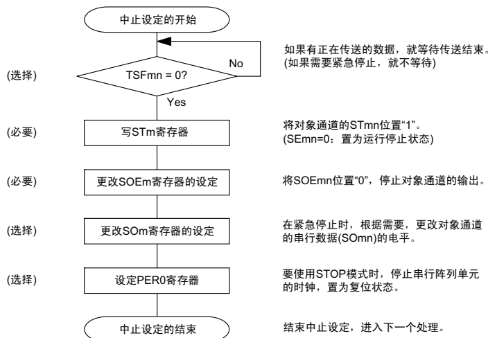
图 12-77 UART 发送的中止步骤
