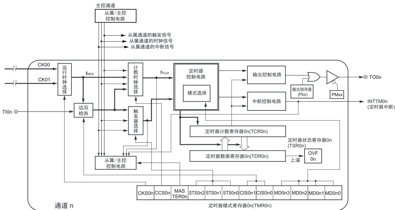
图 6-2 定时器阵列单元 0 的通道 0、2、4、6 的内部框图
