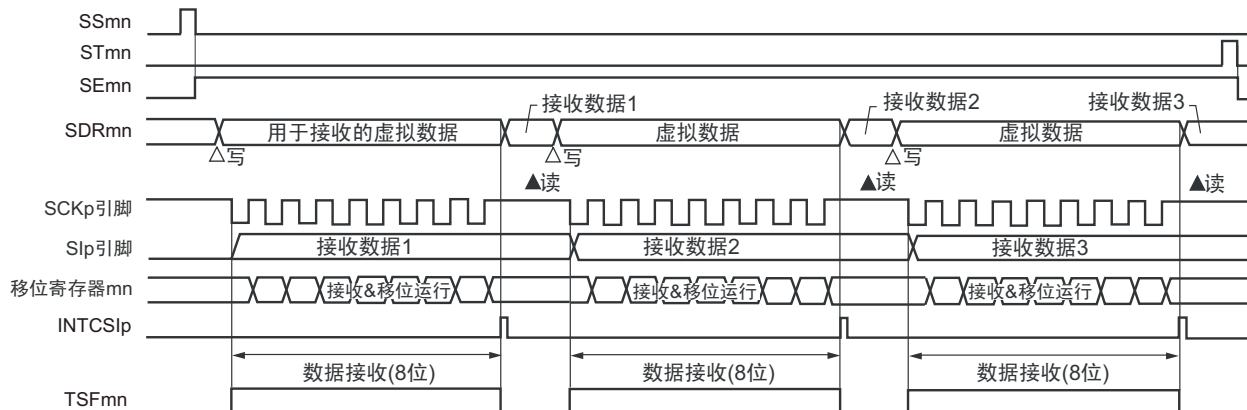
图 12-36 主控接收（单次接收模式）的时序图（类型 1：DAPmn=0、CKPmn=0）
