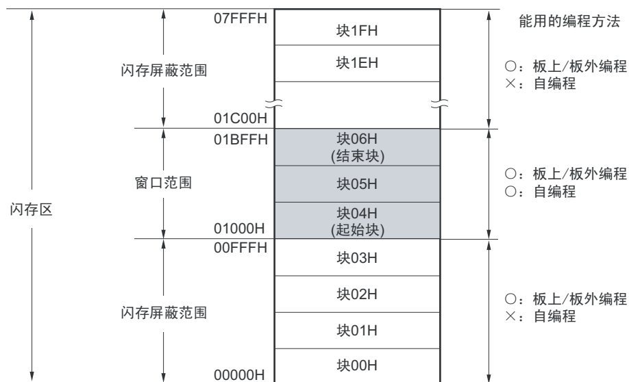
图 26-11 闪存屏蔽窗口的设定例子 (对象器件: R5F10RxC, 起始块: 04H, 结束块: 06H)
