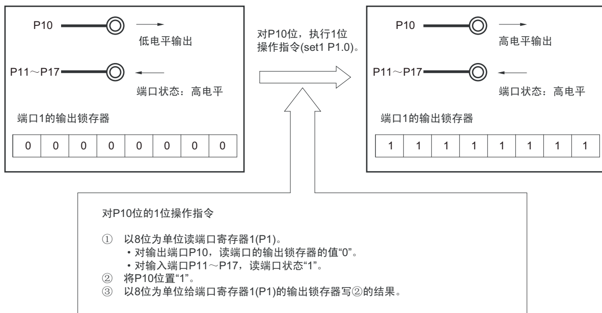
图 4-15 1 位操作指令（P10 的情况）
