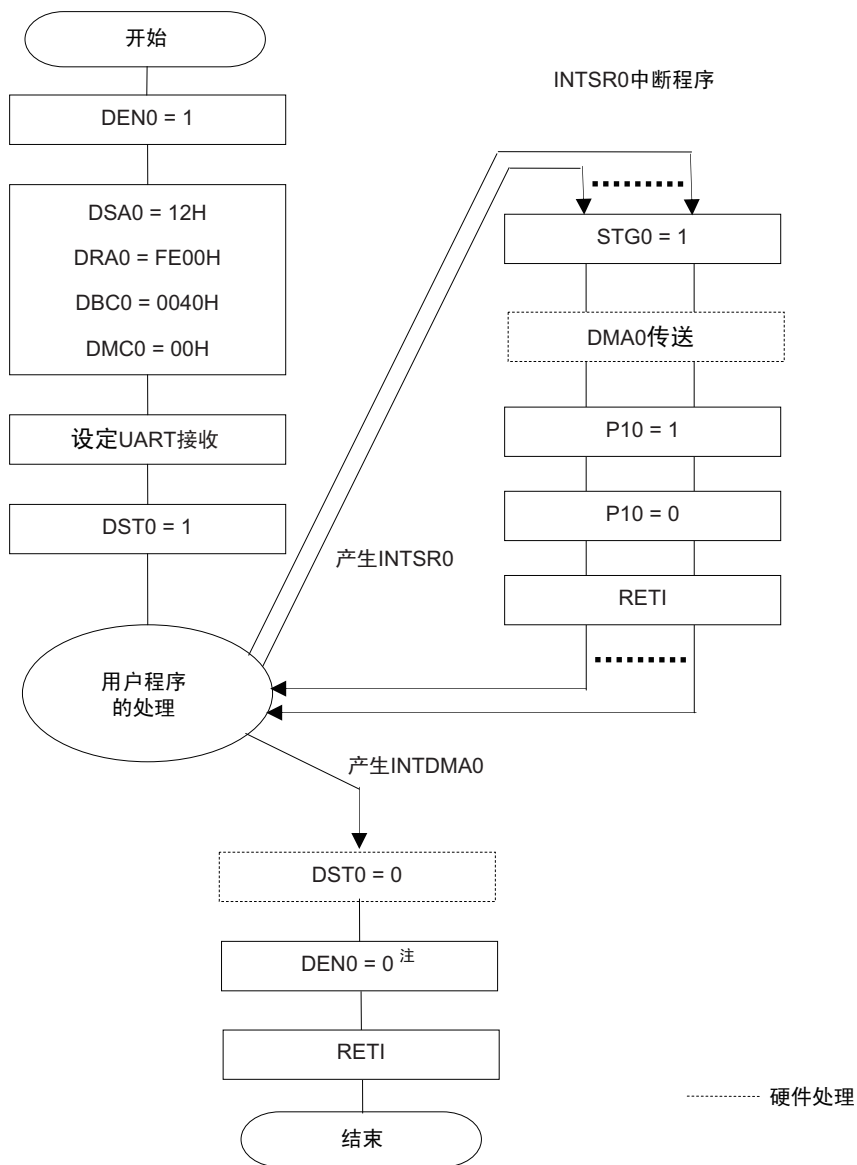
图 16-9 UART 连续接收 +ACK 发送的设定例子
