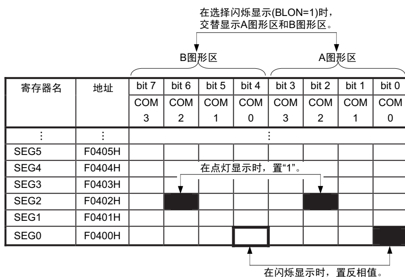
图 14-16 图形切换显示时的 LCD 显示寄存器的设定例子
