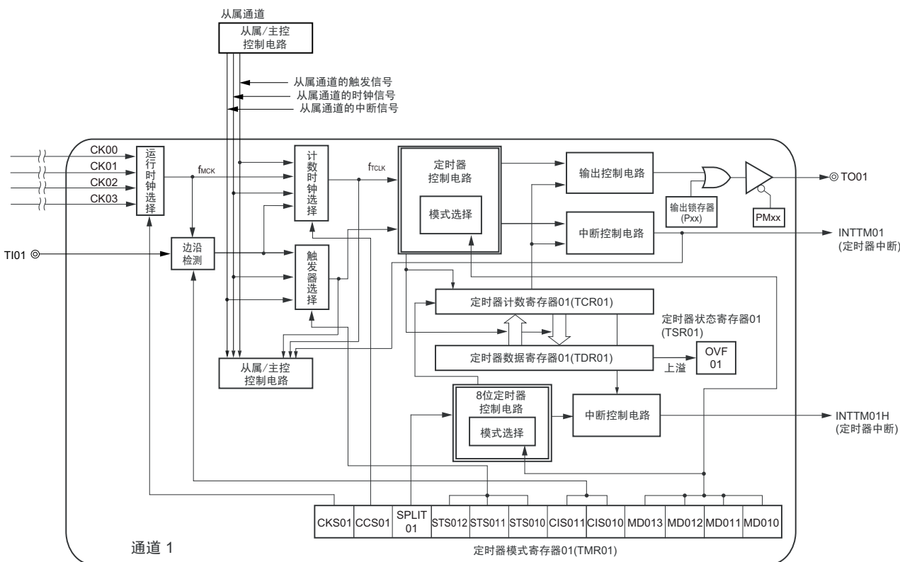
图 6-3 定时器阵列单元 0 的通道 1 的内部框图
