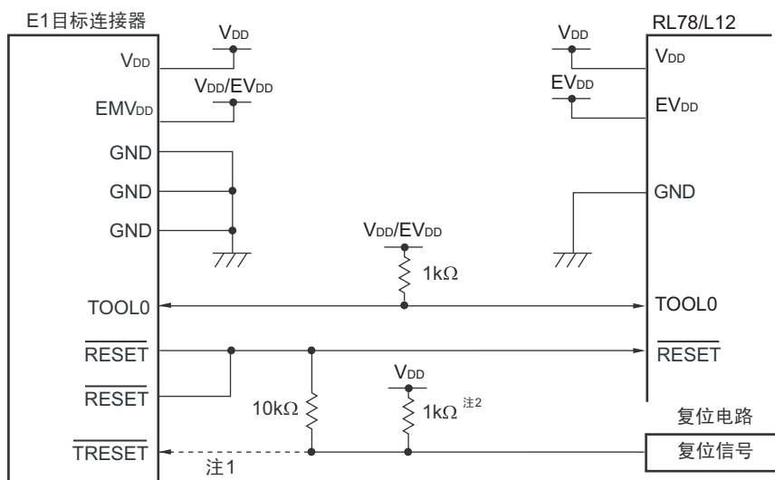
图 27-1 E1 on-chip 调试仿真器和 RL78/L12 的连接例子
