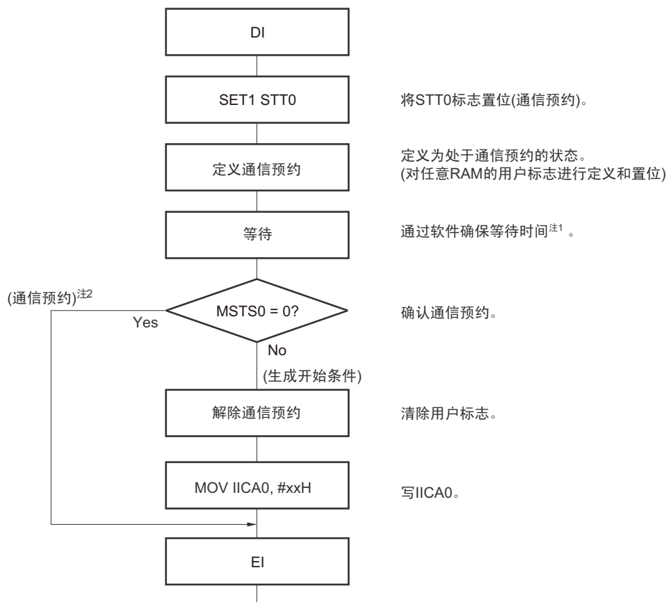
图 13-27 通信预约步骤
