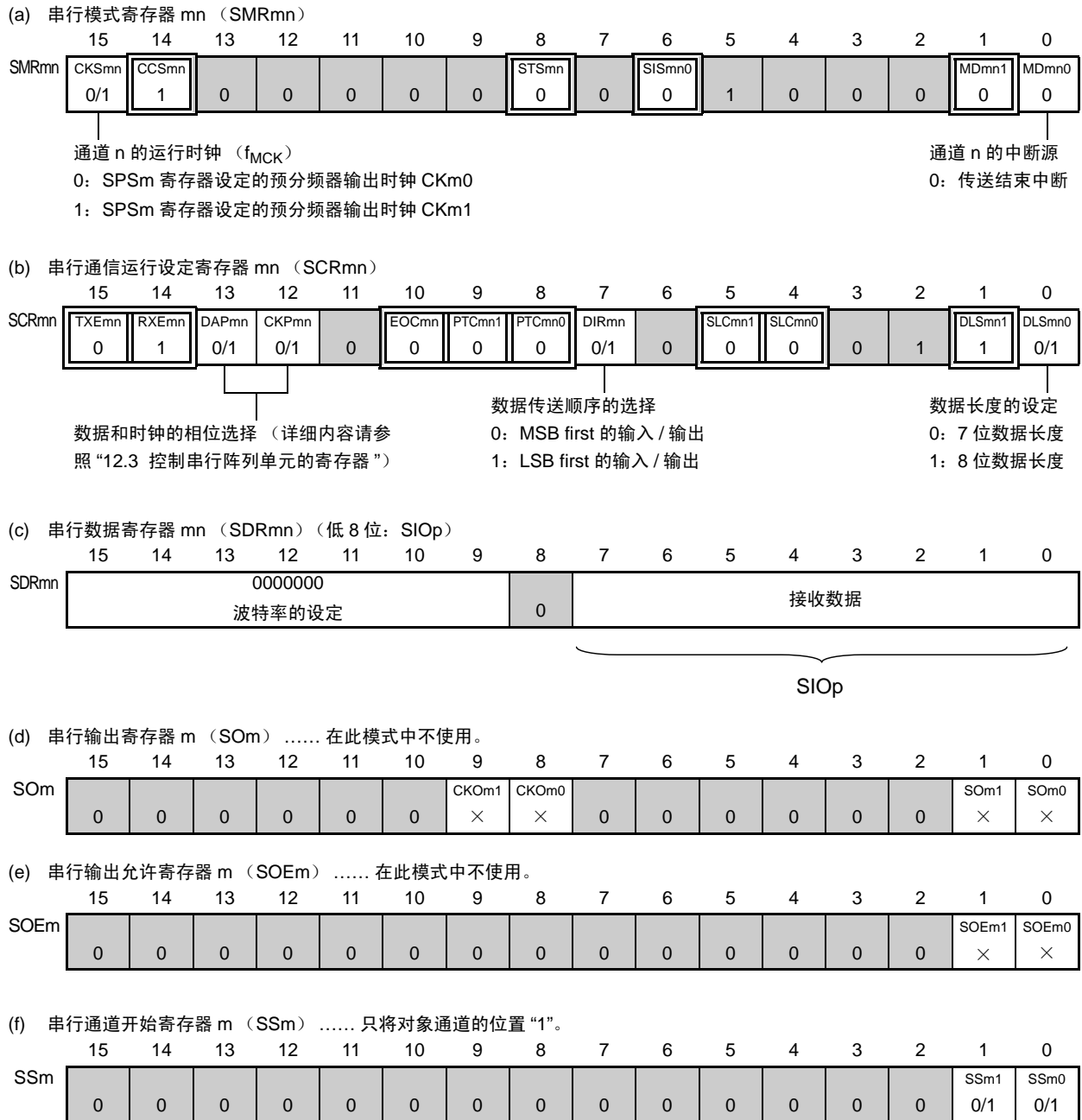
图 12-56 3 线串行 I/O (CSI00、CSI01) 从属接收时的寄存器设定内容例子
