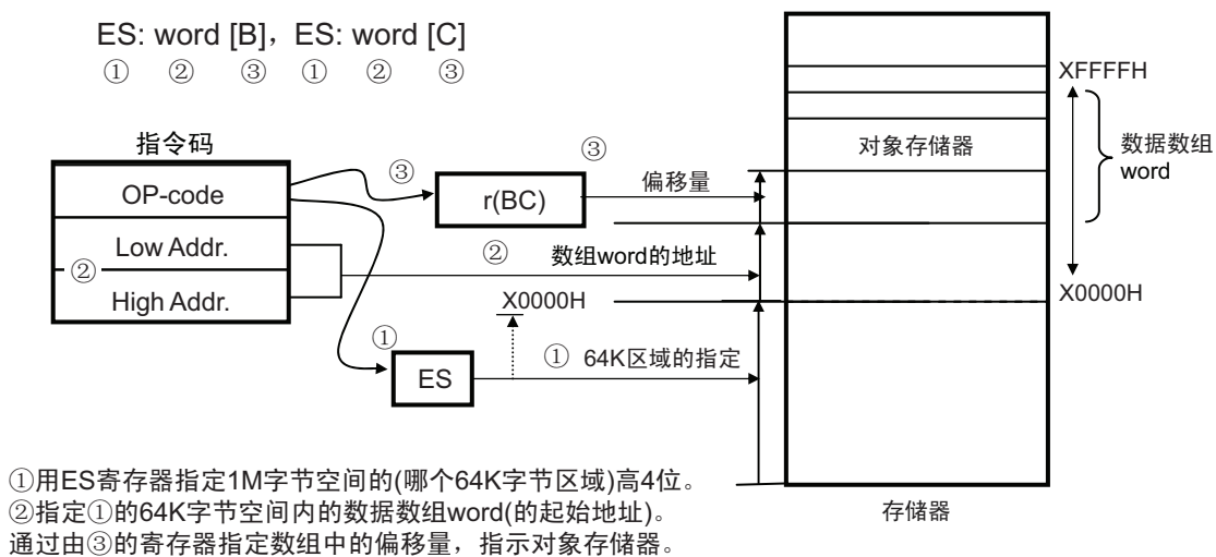
图 3-33 ES:word[BC] 的例子
