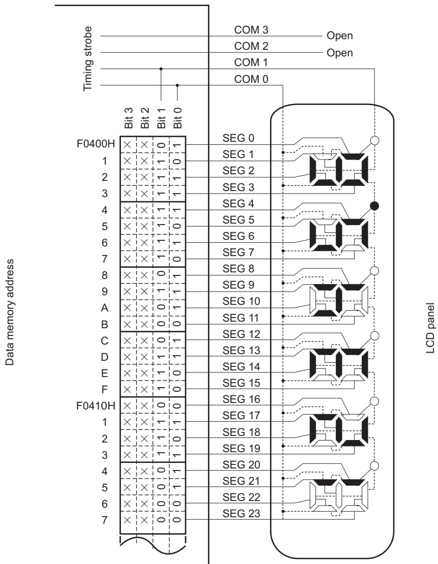
图 14-33 2 个时间片的 LCD 显示屏的连线例子
