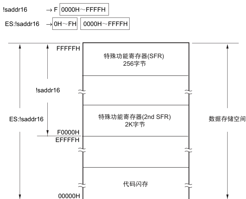
图 3-13 数据存取区的扩充
