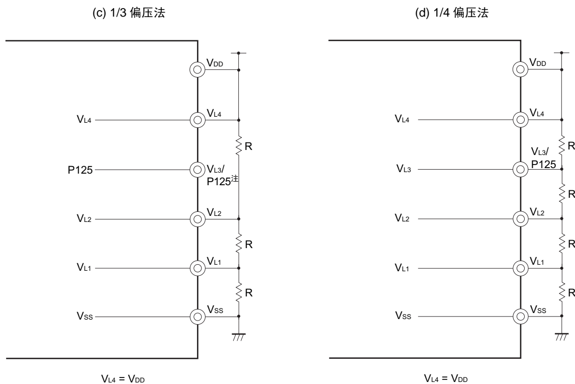
图 14-24 LCD 驱动电源的连接例子（外部电阻分割方式）(2/2)
