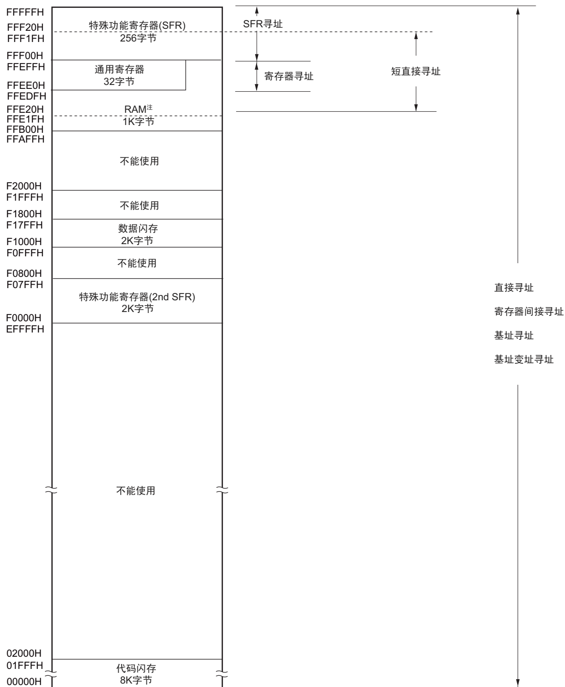
图 3-5 数据存储器和寻址的对应 (R5F10Rx8 (x=B、F、G、J))
