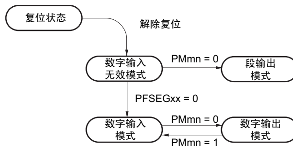
图 4-11 SEGxx/ 端口引脚功能的状态转移图
