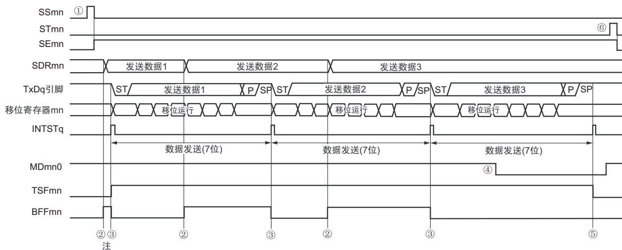
图 12-81 UART 发送（连续发送模式）的时序图
