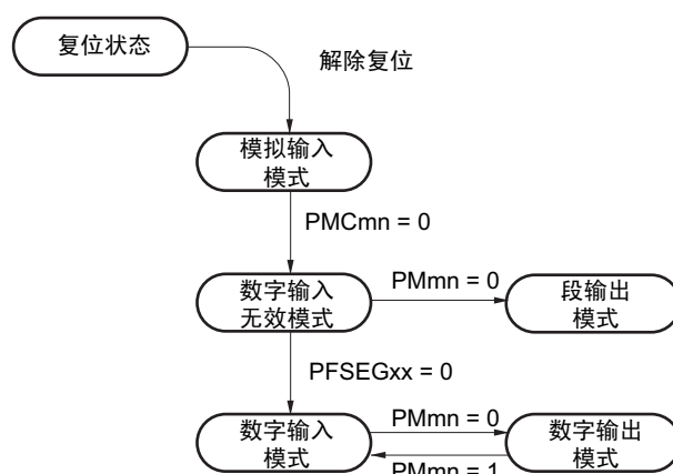
图 4-12 ANIXx/SEGxx/ 端口引脚功能的状态转移图
