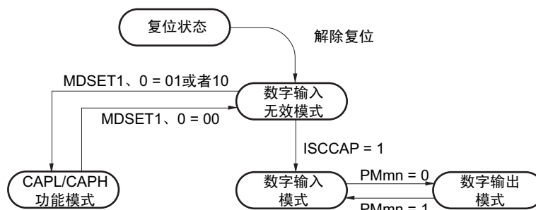
图 4-14 CAPL/P126、CAPH/P127 引脚功能的状态转移图
