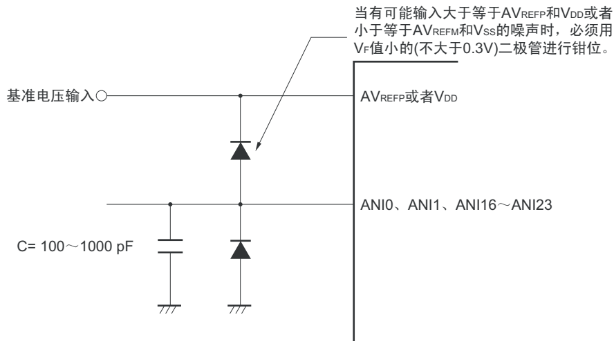
图 11-41 模拟输入引脚的处理
