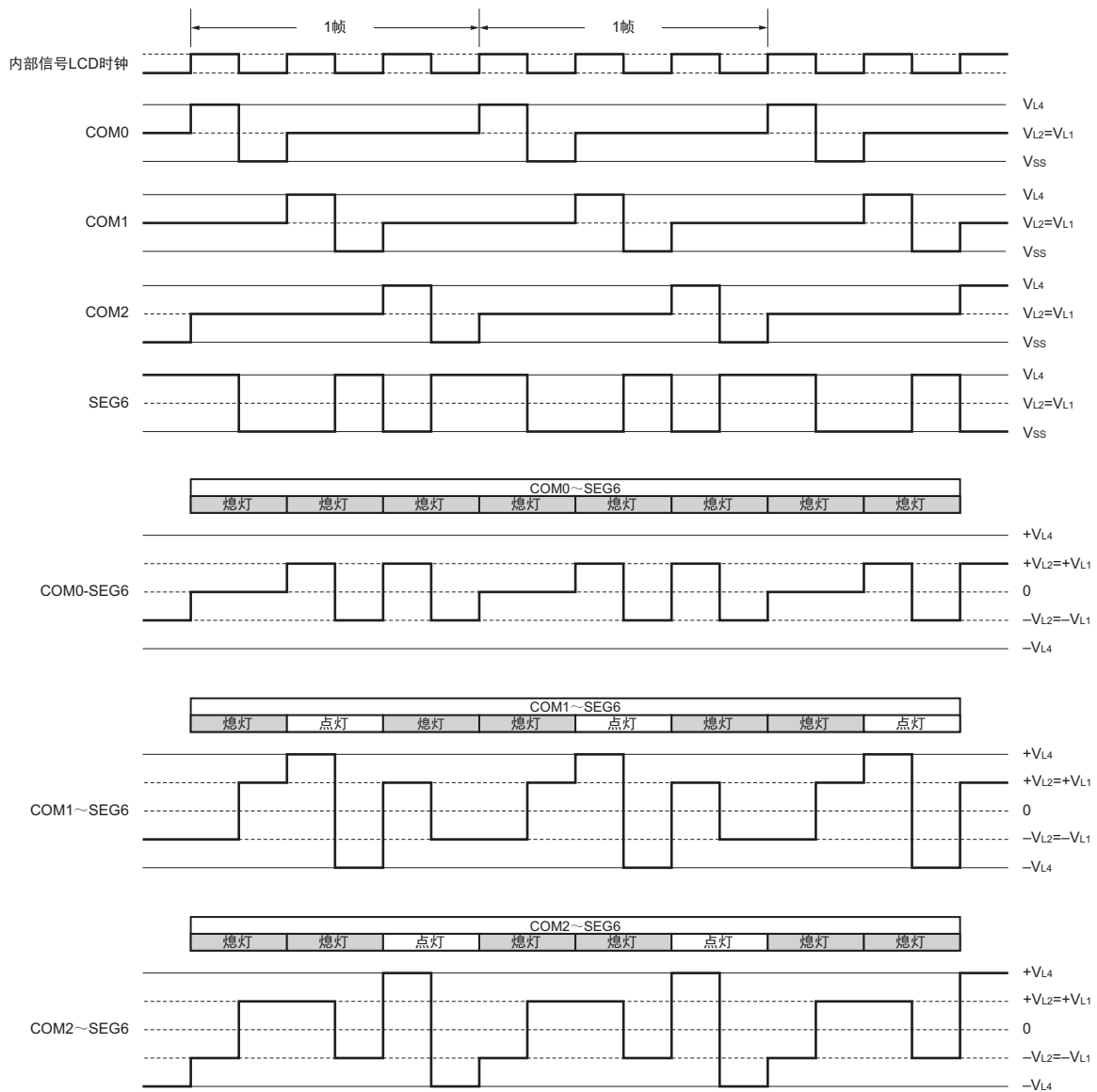
图 14-37 SEG6 和各公共信号之间的 3 个时间片的 LCD 驱动波形例子 (1/2 偏压法)
