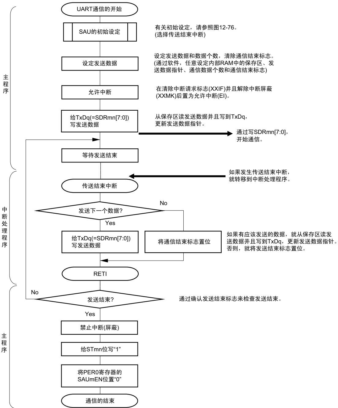
图 12-80 UART 发送（单次发送模式）的流程图
