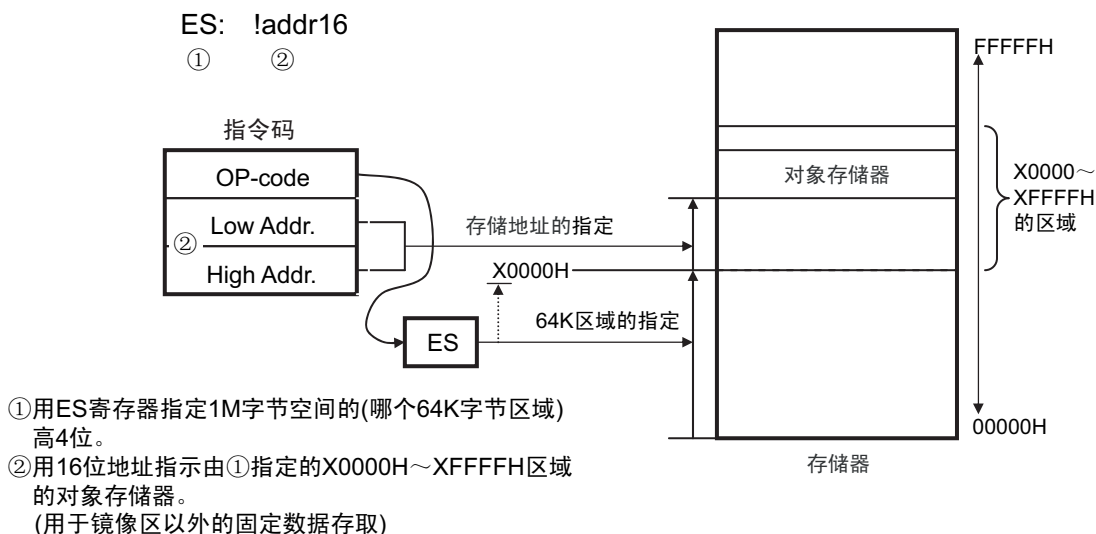
图 3-22 ES:ADDR16 的例子
