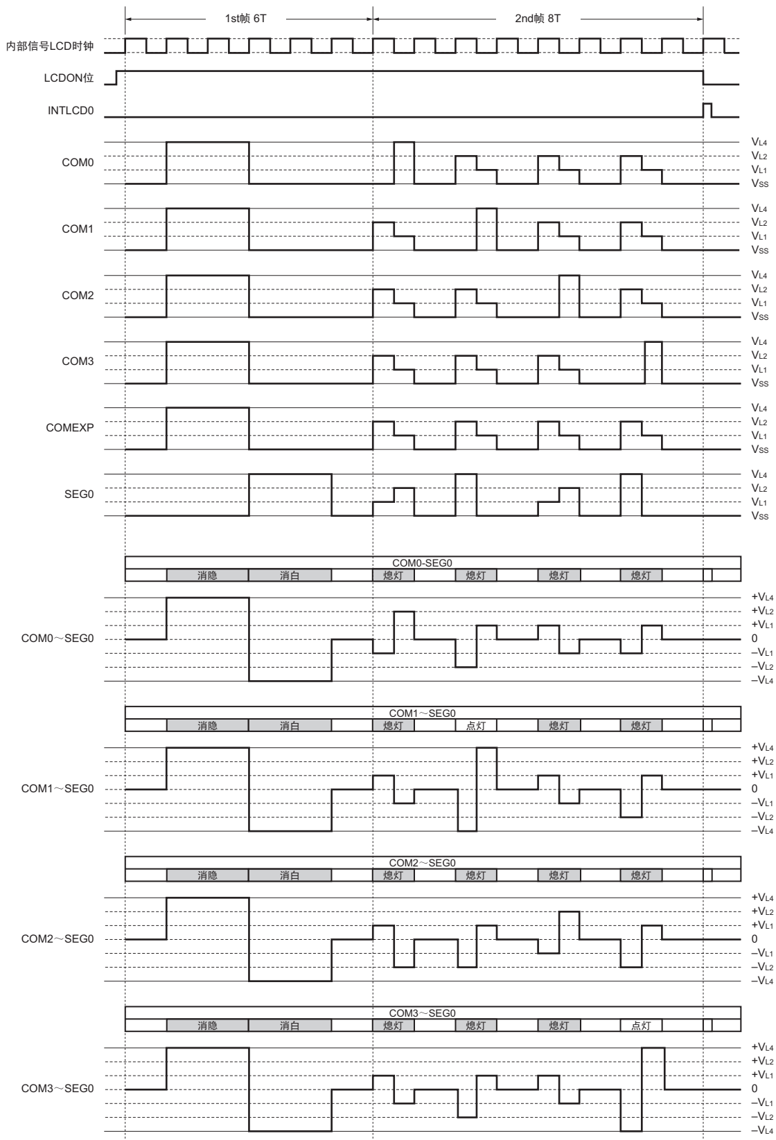
图 14-46 记忆性液晶波形的 LCD 驱动波形例子（4 个时间片、1/3 偏压法）
