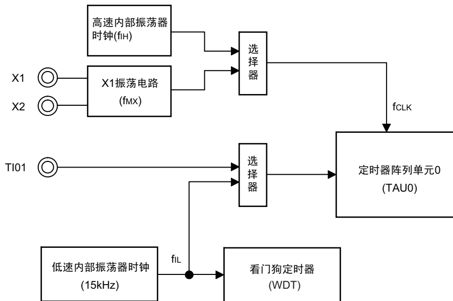
图 23-12 频率检测功能的结构
