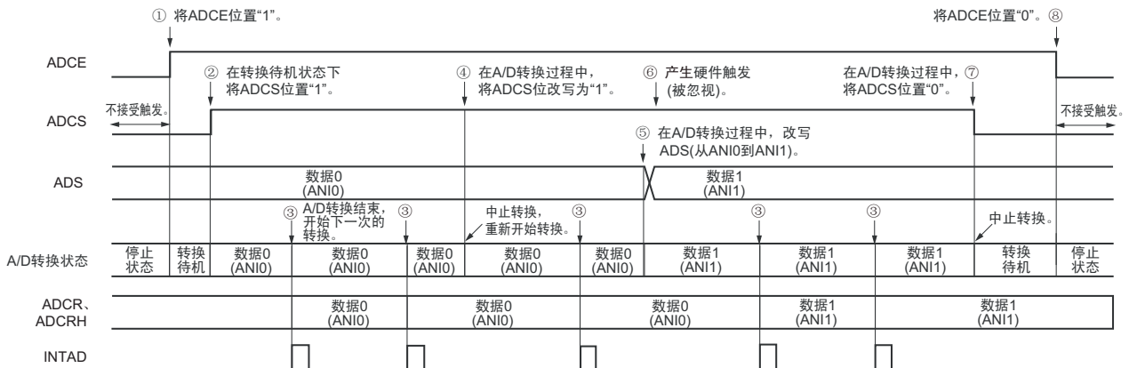
图 11-20 软件触发模式（连续转换模式）的运行时序例子
