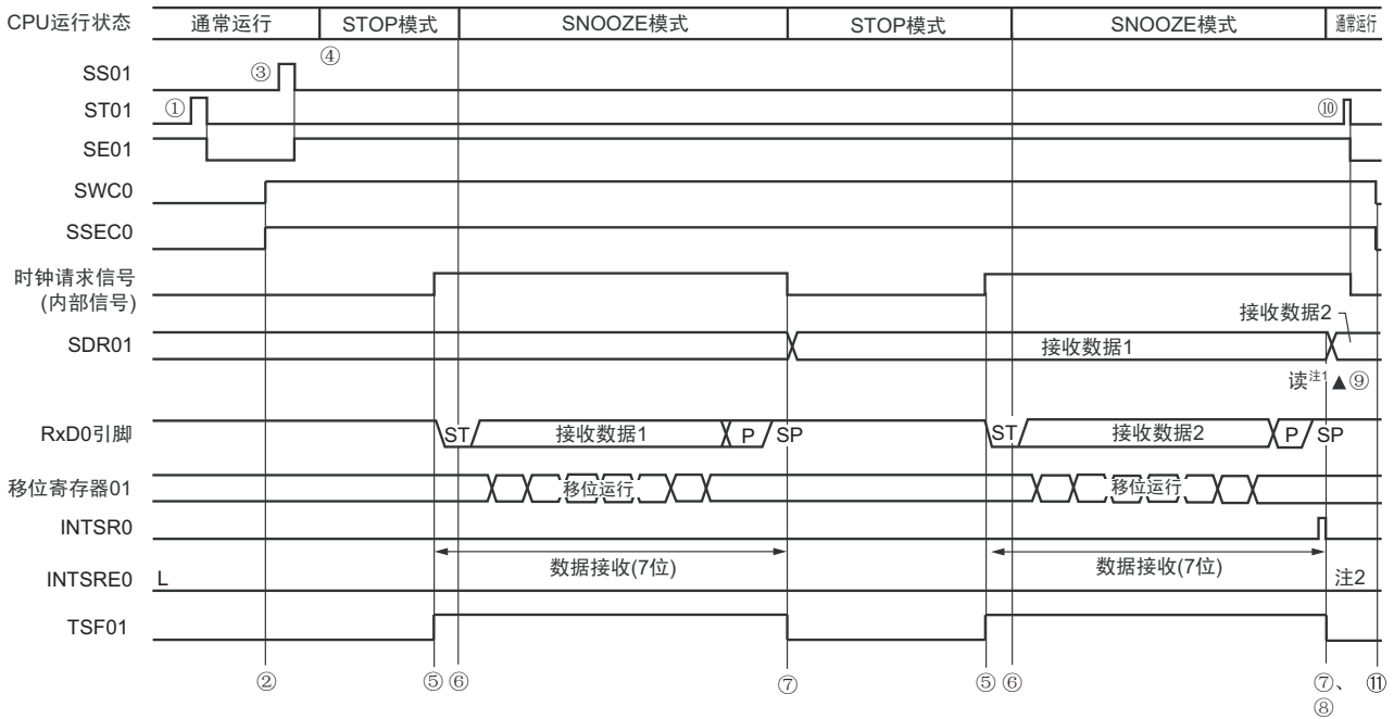
图 12-92 SNOOZE 模式运行（异常运行②）的时序图
