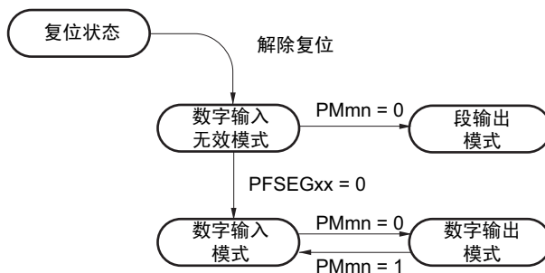
图 14-13 SEGxx/ 端口引脚功能的状态转移图
