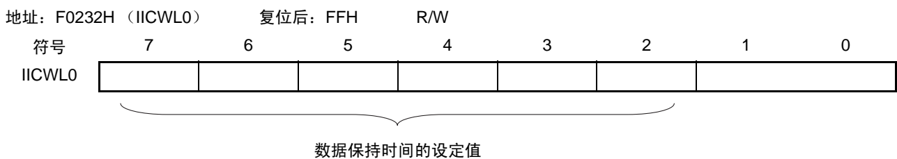
图 13-10 IICA 低电平宽度设定寄存器 0 (IICWL0) 的格式
