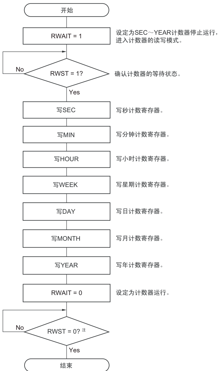
图 7-20 实时时钟计数器的写操作步骤
