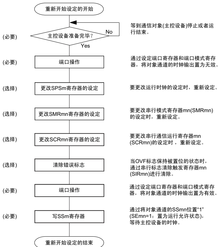
图 12-59 从属接收的重新开始设定步骤
