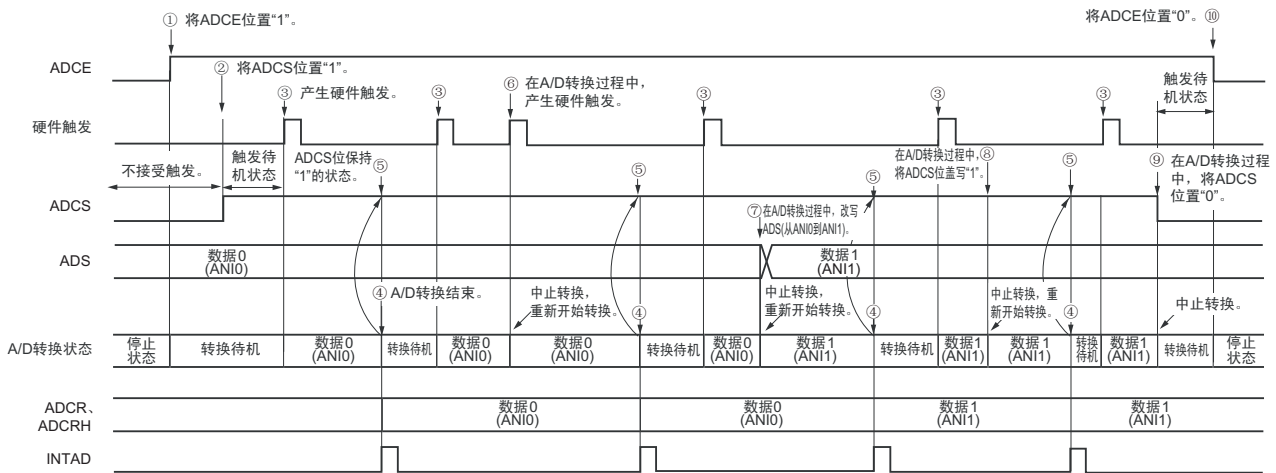
图 11-23 硬件触发无等待模式（单次转换模式）的运行时序例子
