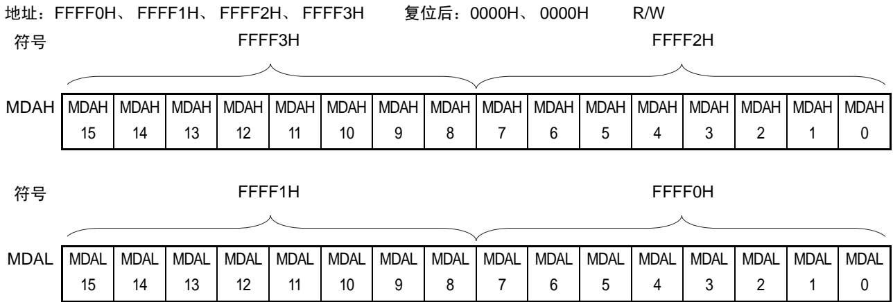
图 15-2 乘除数据寄存器 A (MDAH、MDAL) 的格式
