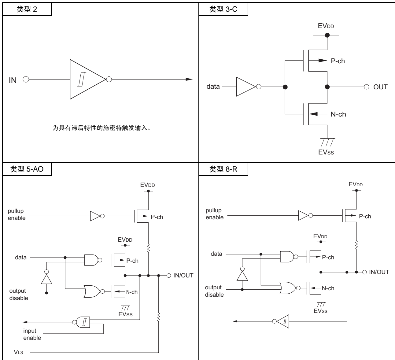
图 2-1 引脚的输入 / 输出电路一览表 (1/4)
