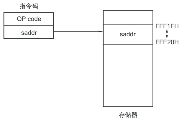
图 3-23 短直接寻址的概要
