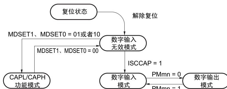
图 14-11 CAPL/P126、CAPH/P127 引脚功能的状态转移图
