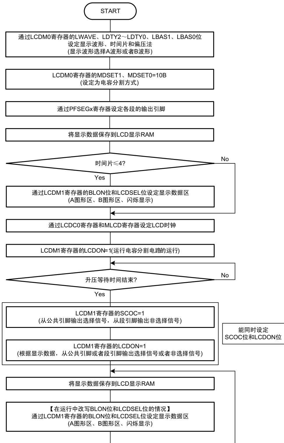
图 14-21 通常液晶波形时的电容分割方式的设定步骤
