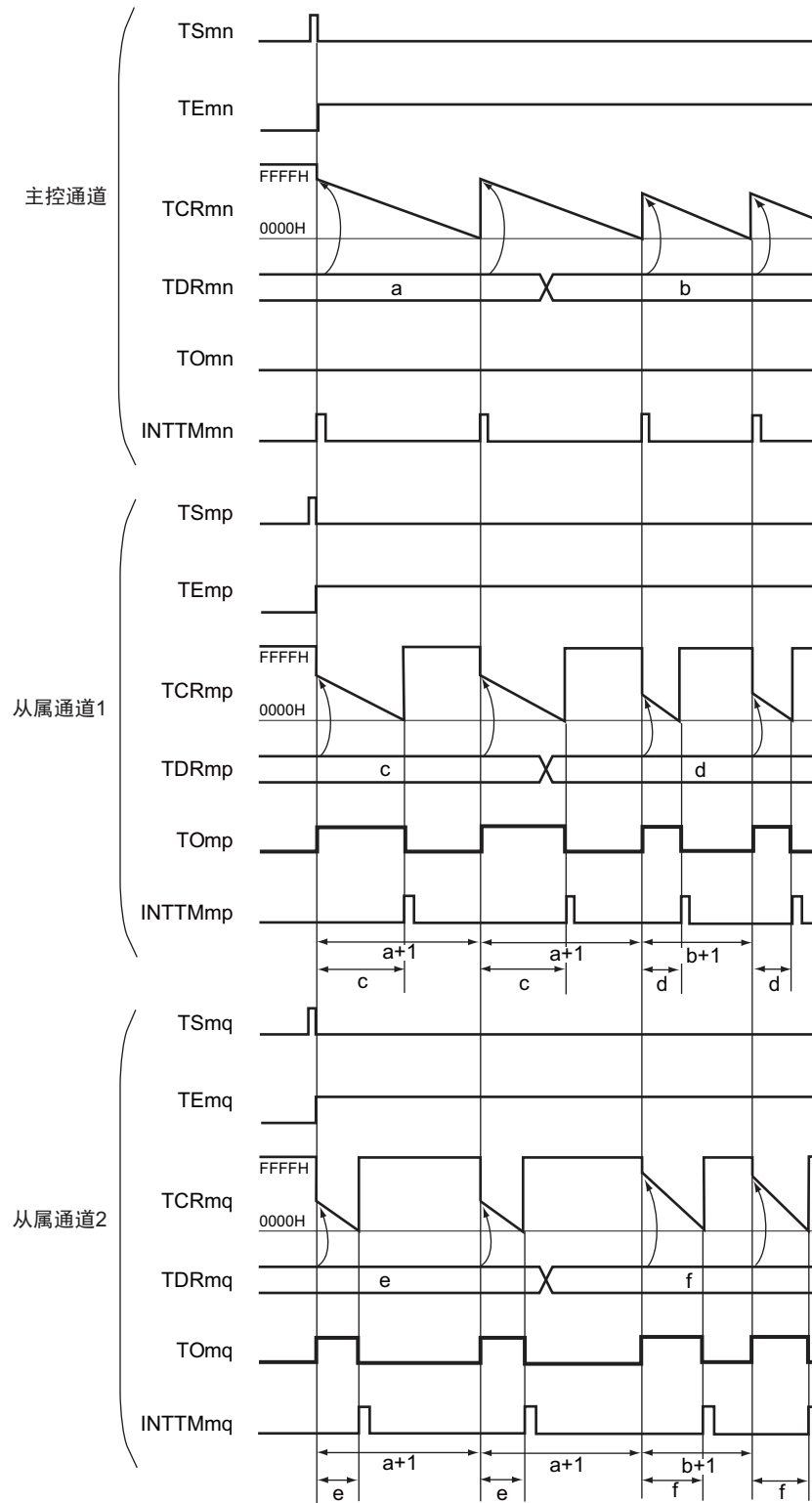
图 6-78 作为多重 PWM 输出功能的运行基本时序例子（输出 2 种 PWM 的情况）(1/2)
