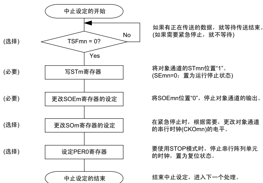
图 12-34 主控接收的中止步骤
