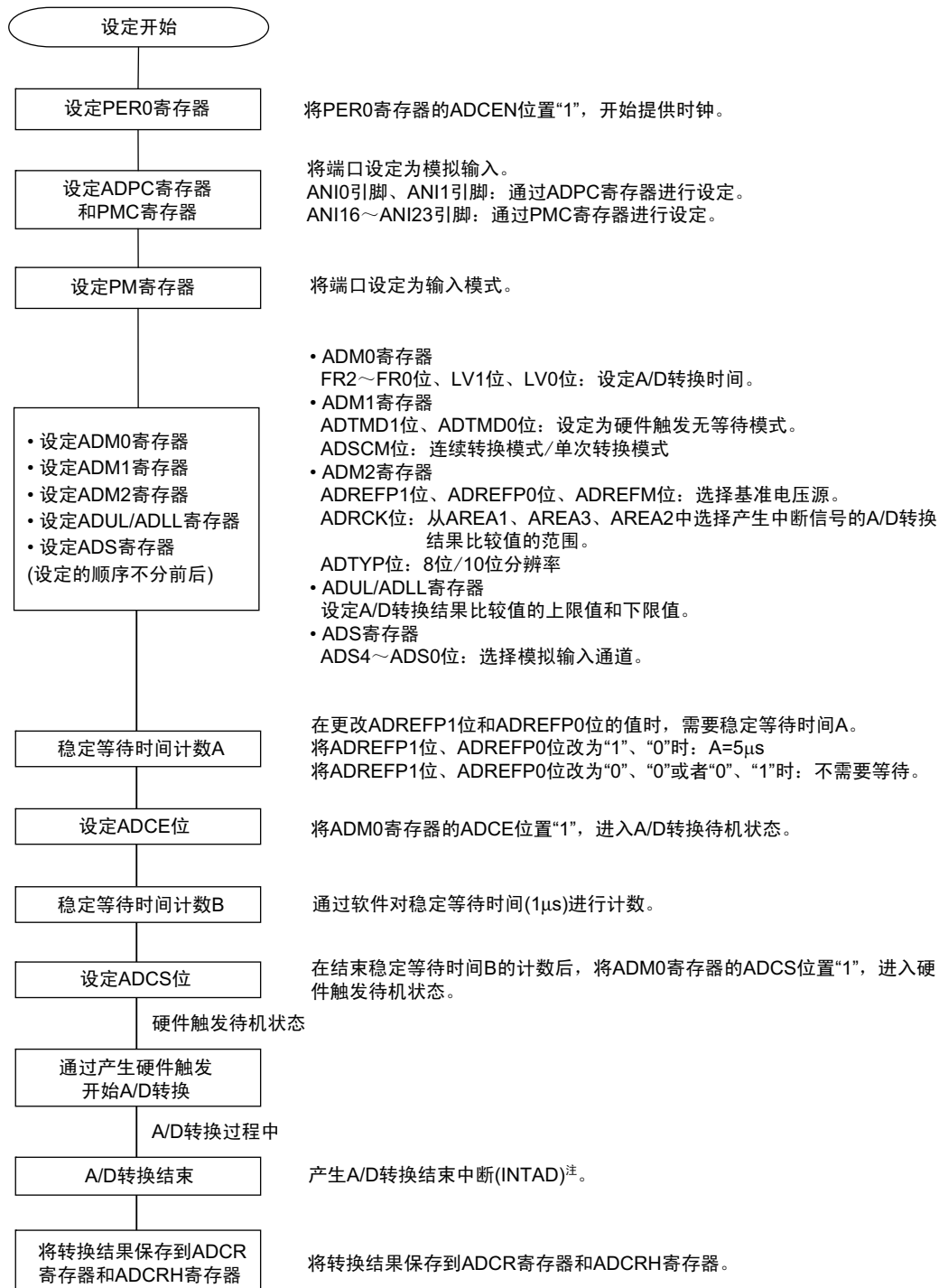
图 11-27 硬件触发无等待模式的设定
