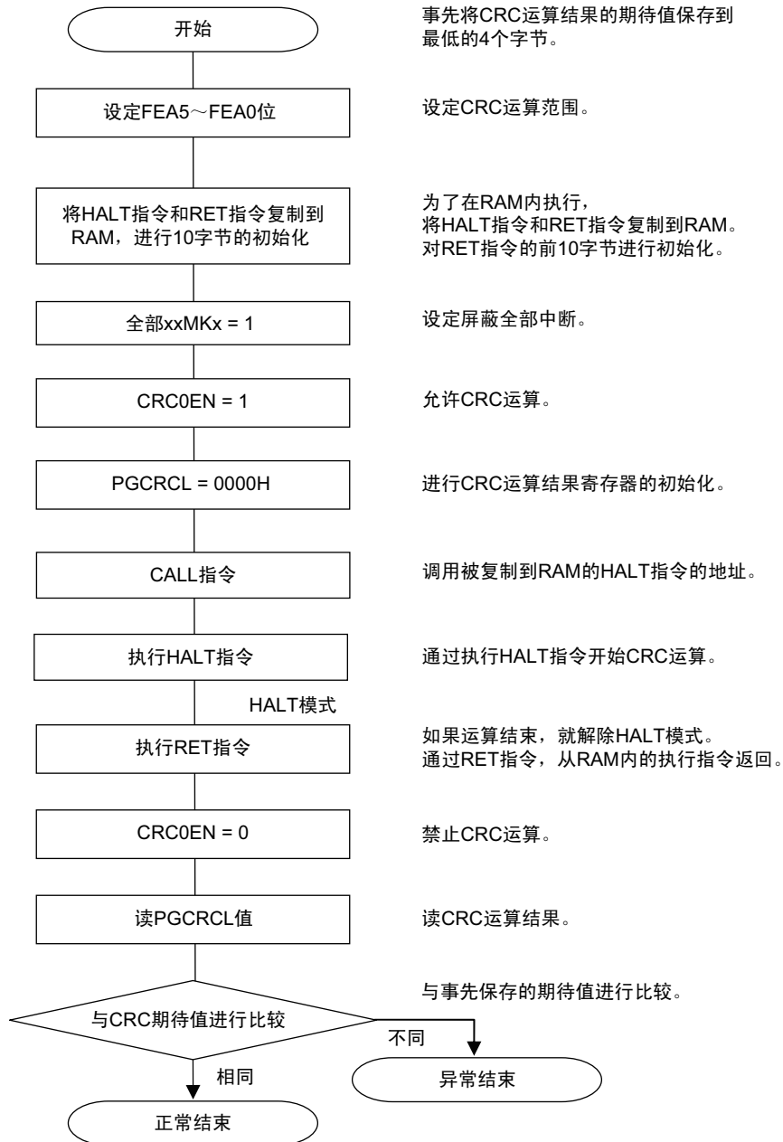
图 23-3 闪存 CRC 运算功能（高速 CRC）的流程图
