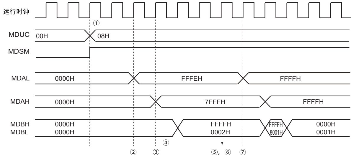
图 15-7 乘法运算（带符号）的时序图（ -2 \times 32767 = -65534 ）
