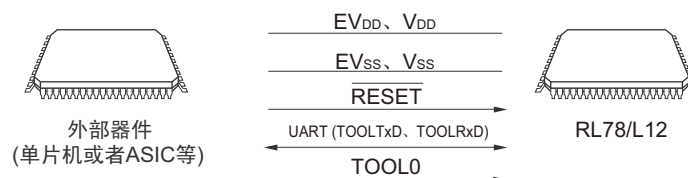
图 26-3 闪存的编程环境
