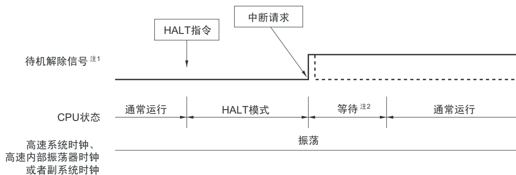
图 19-3 通过中断请求解除 HALT 模式
