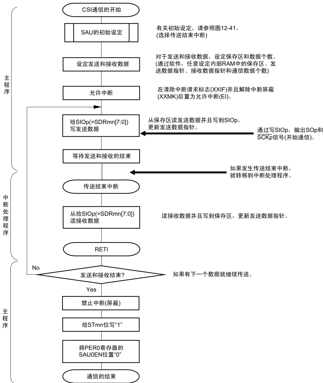
图 12-45 主控发送和接收（单次发送和接收模式）的流程图
