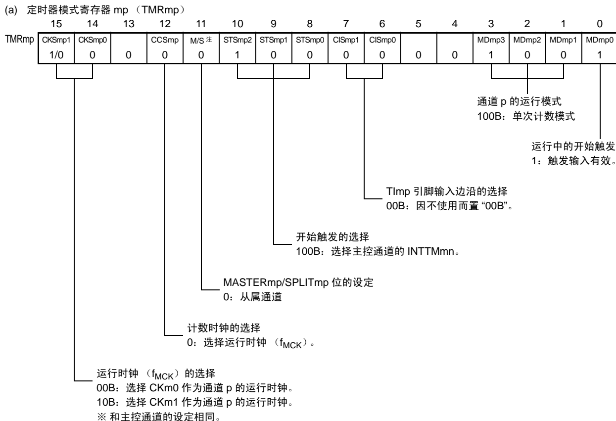
图 6-75 PWM 功能时（从属通道）的寄存器设定内容例子
