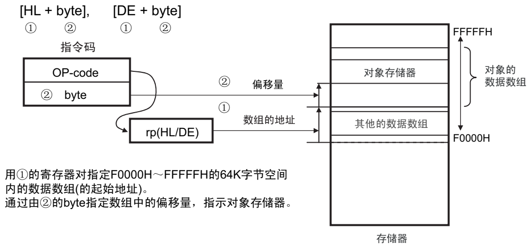
图 3-29 word[B]、word[C] 的例子
