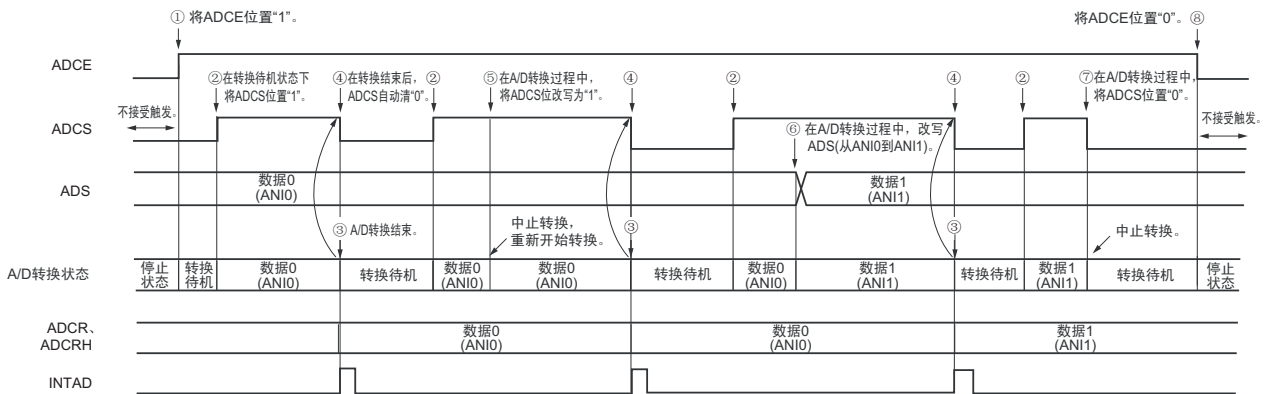
图 11-21 软件触发模式（单次转换模式）的运行时序例子
