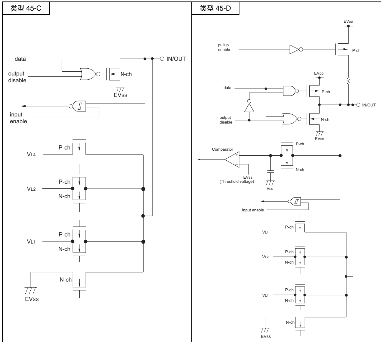
图 2-1 引脚的输入 / 输出电路一览表 (4/4)
