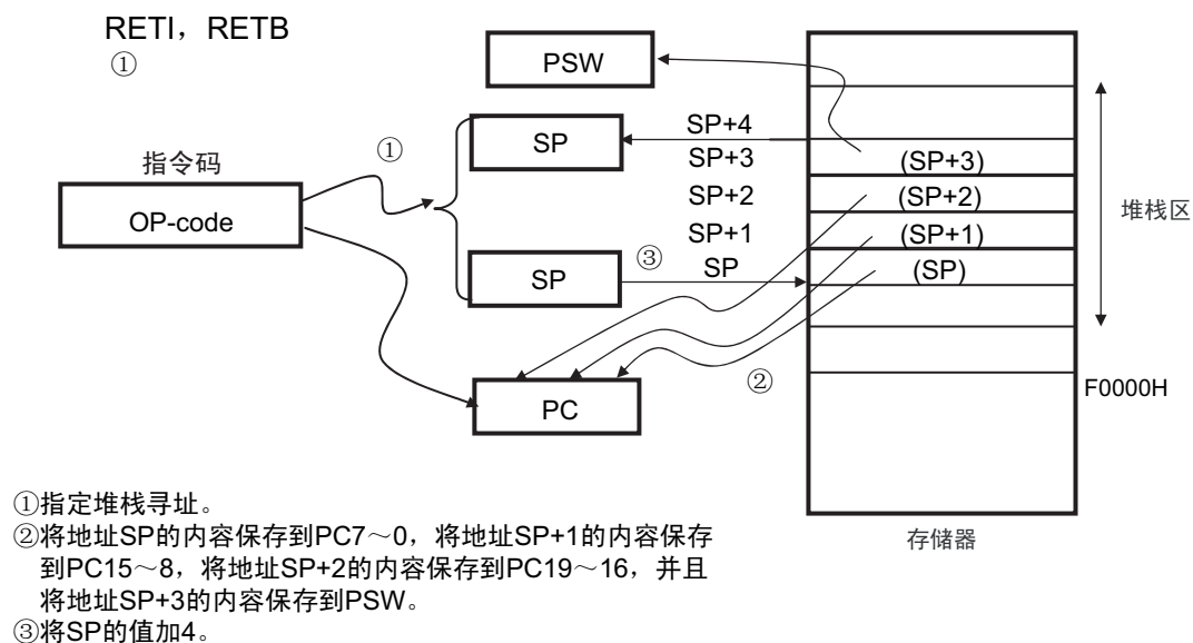
图 3-41 RETI、RETB 的例子
