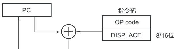
图 3-14 相对寻址的概要
