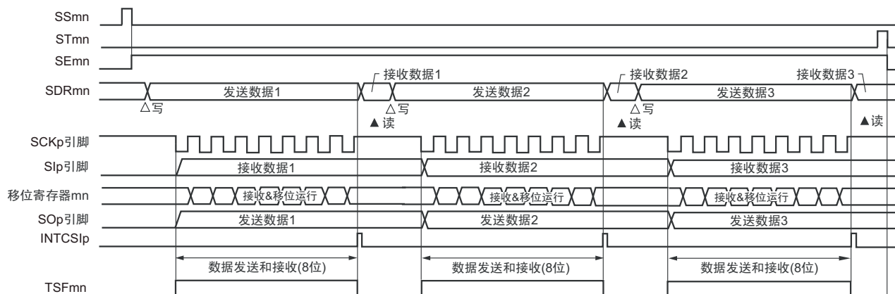
图 12-66 从属发送和接收（单次发送和接收模式）的时序图（类型 1：DAPmn=0、CKPmn=0）
