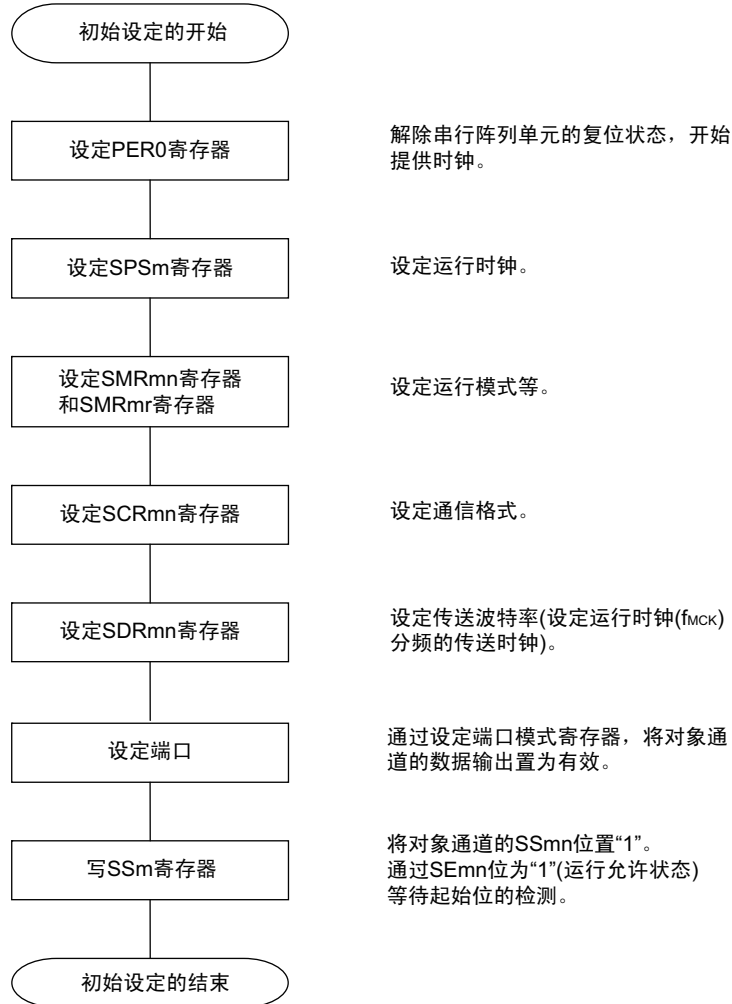
图 12-84 UART 接收的初始设定步骤
