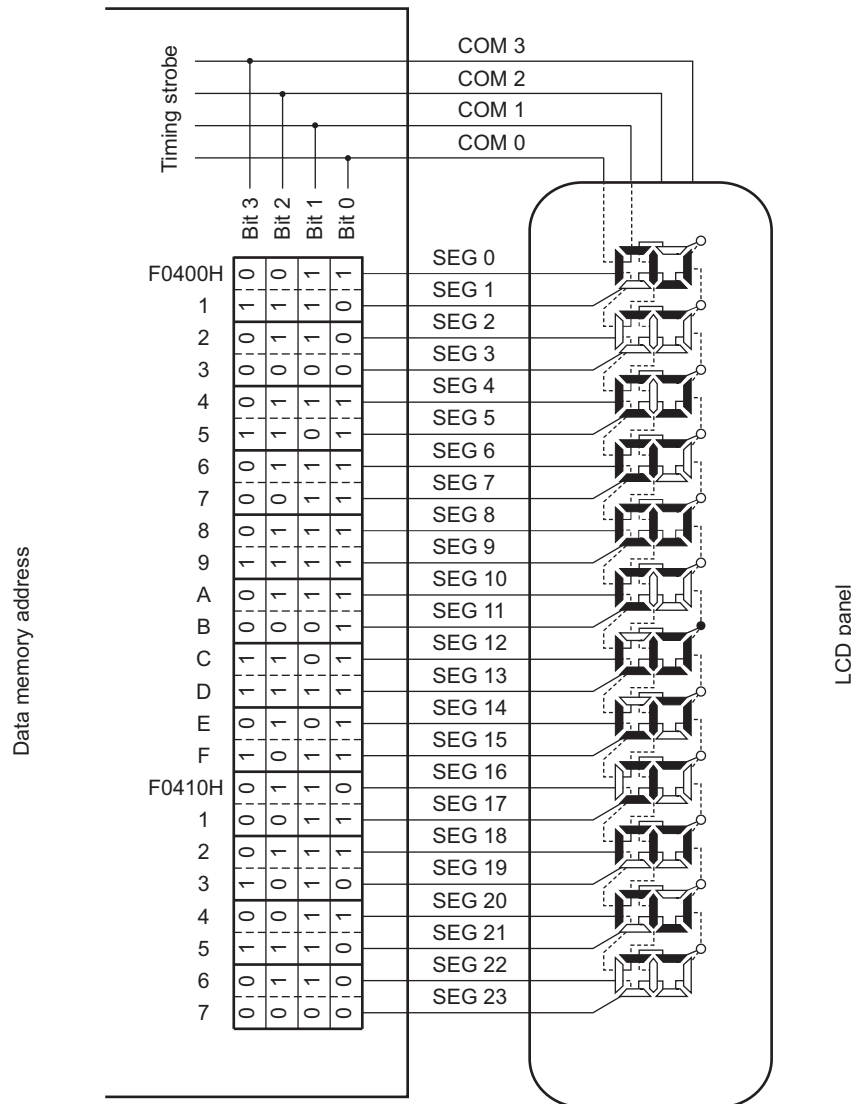
图 14-40 4 个时间片的 LCD 显示屏的连线例子
