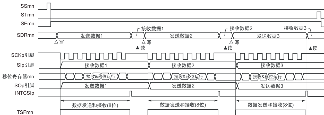
图 12-44 主控发送和接收（单次发送和接收模式）的时序图（类型 1：DAPmn=0、CKPmn=0）
