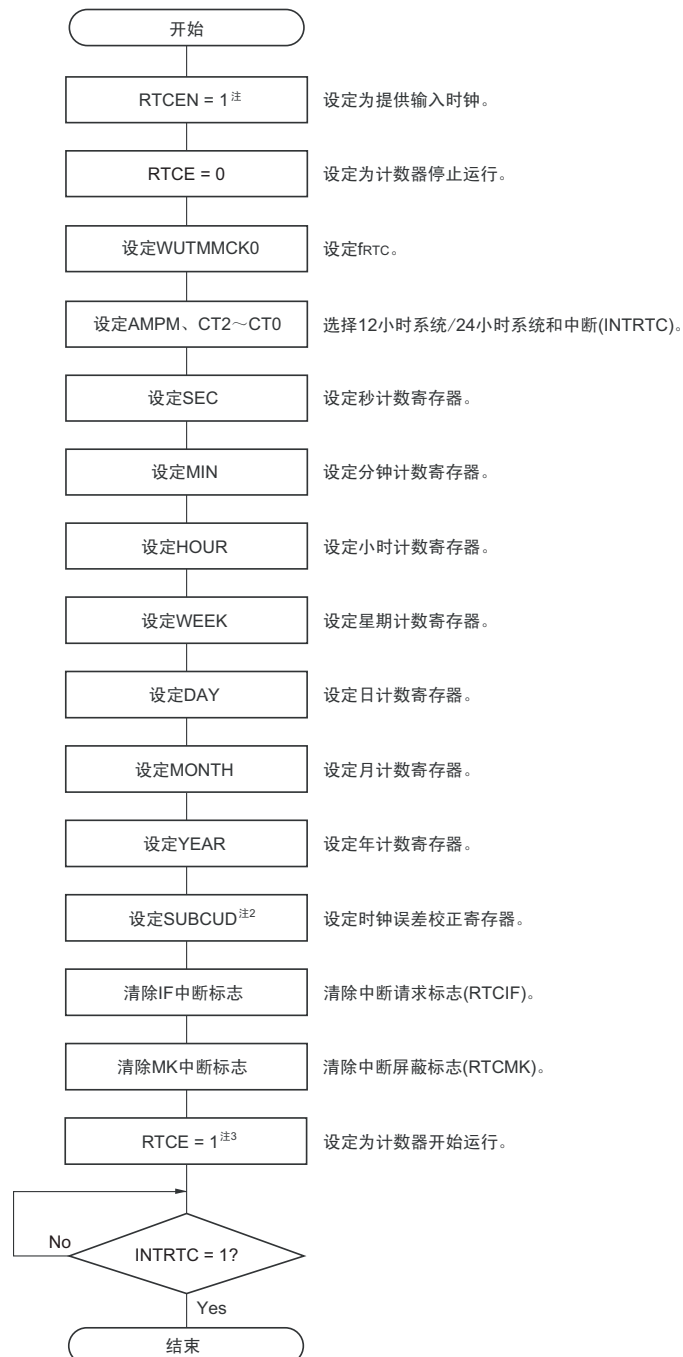
图 7-17 实时时钟的运行开始步骤
