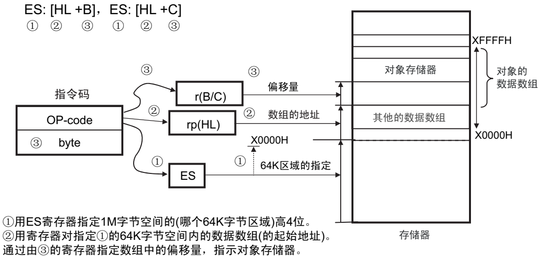
图 3-35 ES:[HL+B]、ES:[HL+C] 的例子
