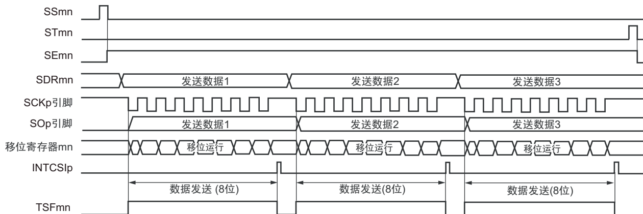
图 12-28 主控发送 (单次发送模式) 的时序图 (类型 1: DAPmn=0、CKPmn=0)
