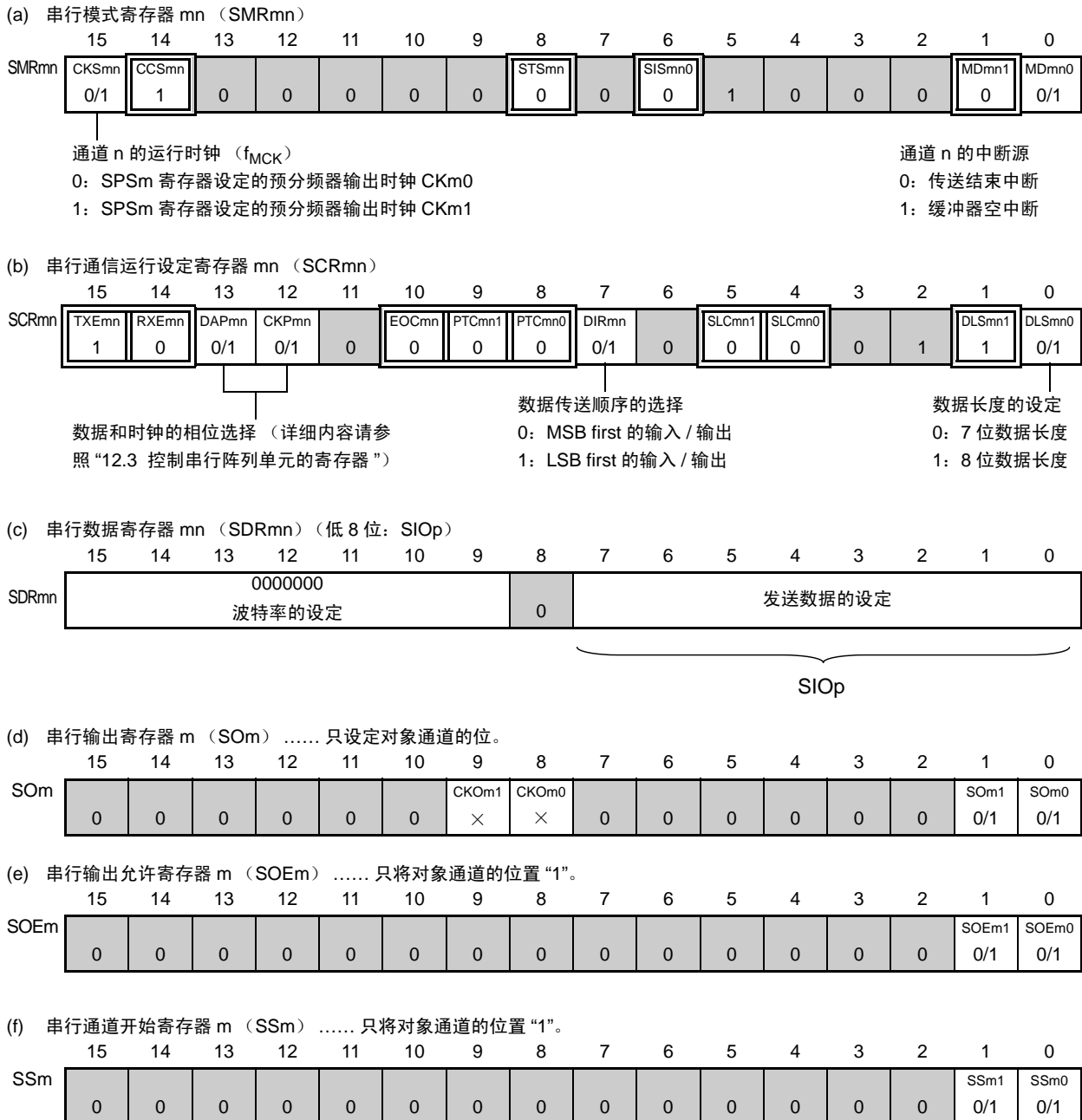
图 12-48 3 线串行 I/O (CSI00、CSI01) 从属发送时的寄存器设定内容例子
