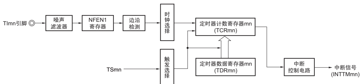
图 6-47 作为外部事件计数器运行的框图
