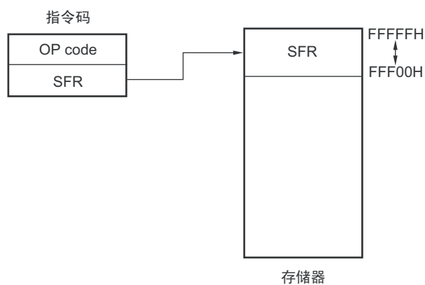
图 3-24 SFR 寻址的概要
