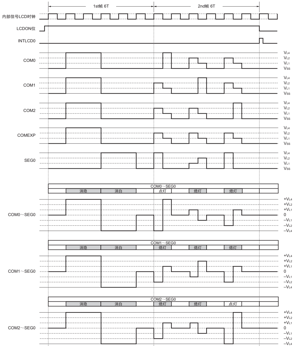
图 14-45 记忆性液晶波形的 LCD 驱动波形例子 (3 个时间片、1/3 偏压法)
