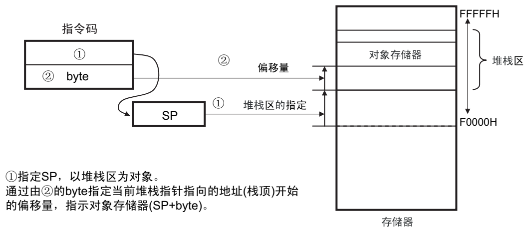
图 3-27 [SP+byte] 的例子
