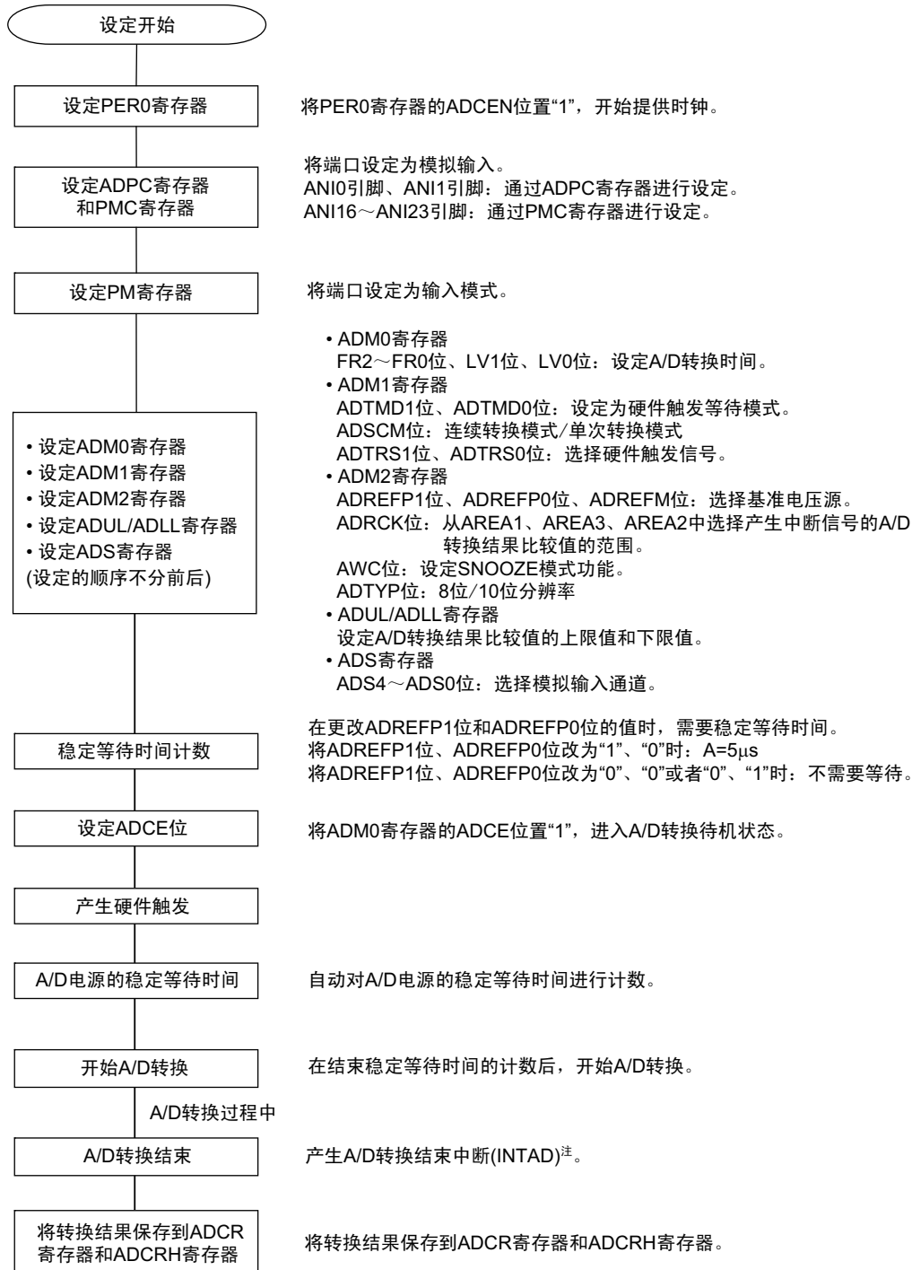
图 11-28 硬件触发等待模式的设定
