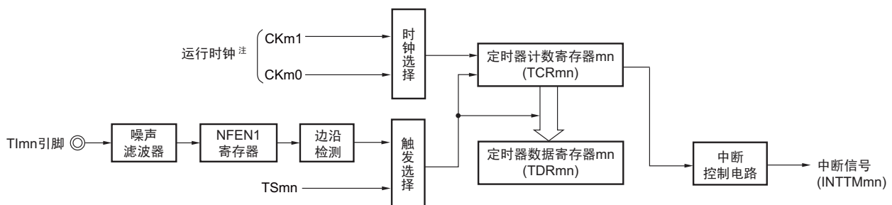
图 6-55 作为输入脉冲间隔测量运行的框图
