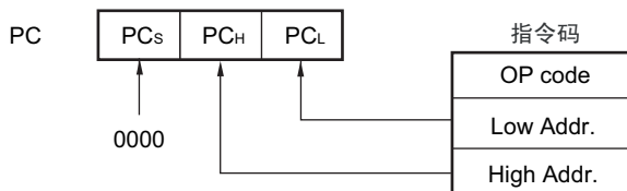
图 3-16 CALL !addr16/BR !addr16 的例子
