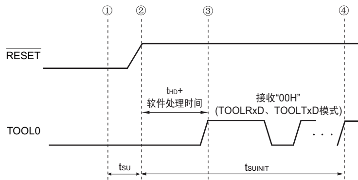
图 26-8 闪存编程模式的进入
