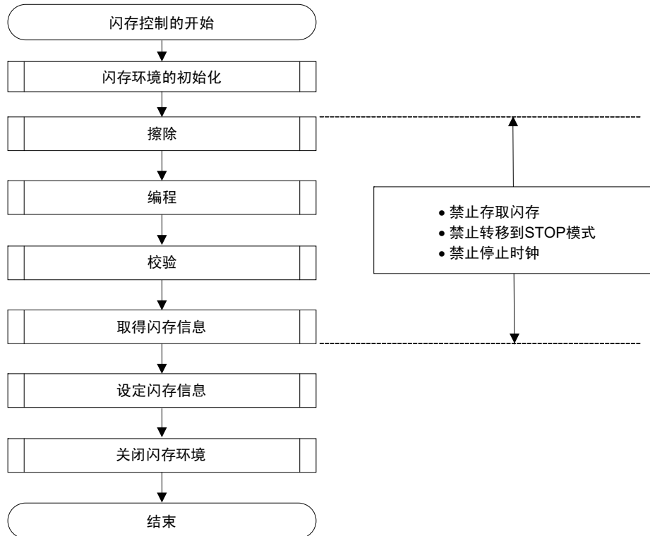
图 26-10 自编程流程（改写闪存）
