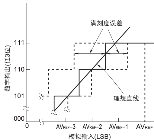
图 11-38 满刻度误差
