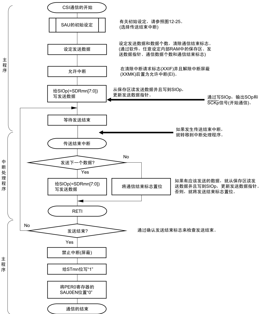
图 12-29 主控发送（单次发送模式）的流程图
