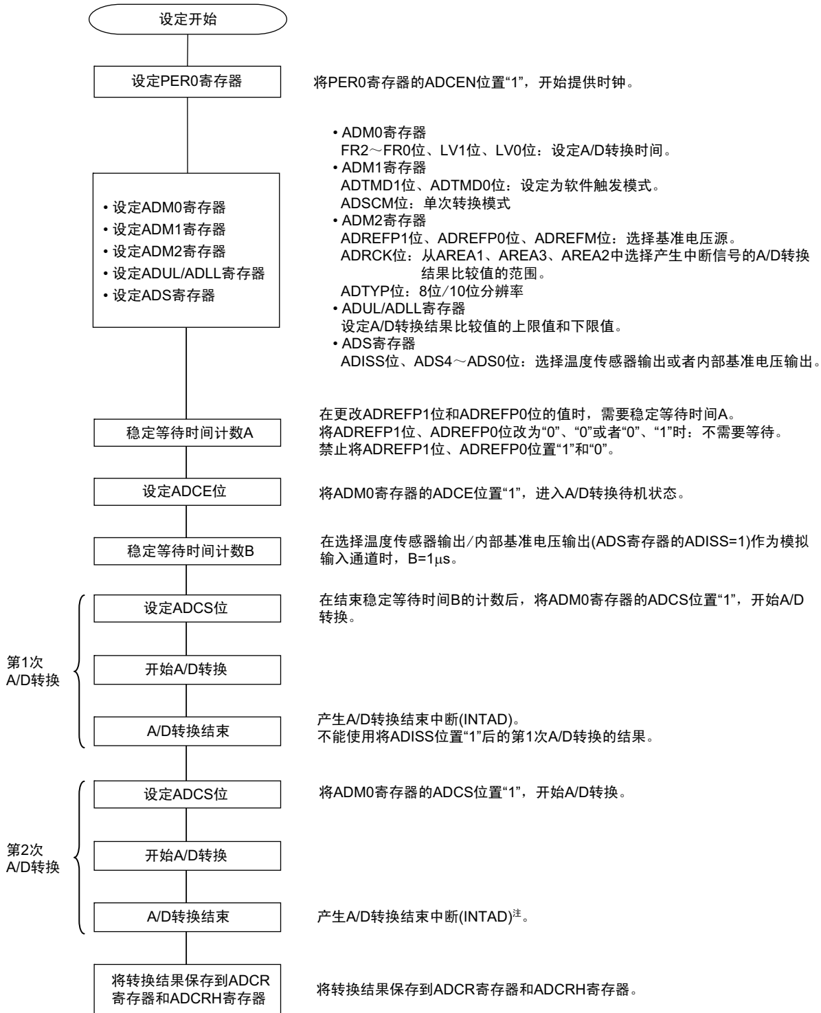
图 11-29 选择温度传感器输出 / 内部基准电压输出时的设定
