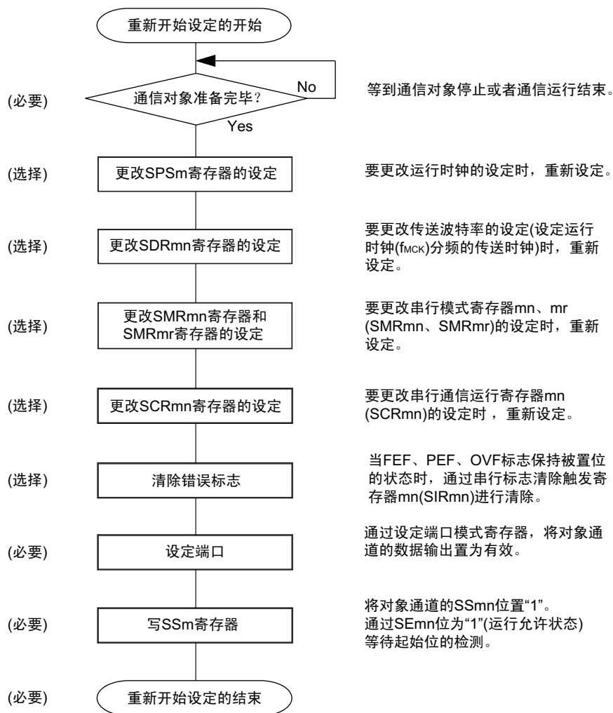
图 12-86 UART 接收的重新开始设定步骤
