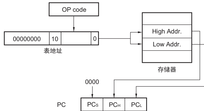
图 3-17 表间接寻址的概要
