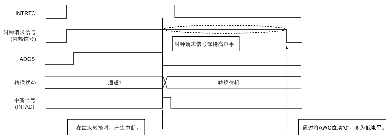
图 11-32 在 A/D 转换结束后发生中断时的运行例子
