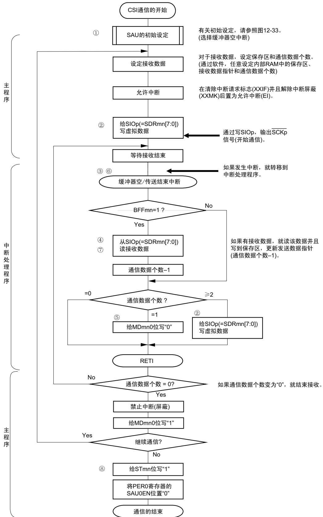
图 12-39 主控接收（连续接收模式）的流程图
