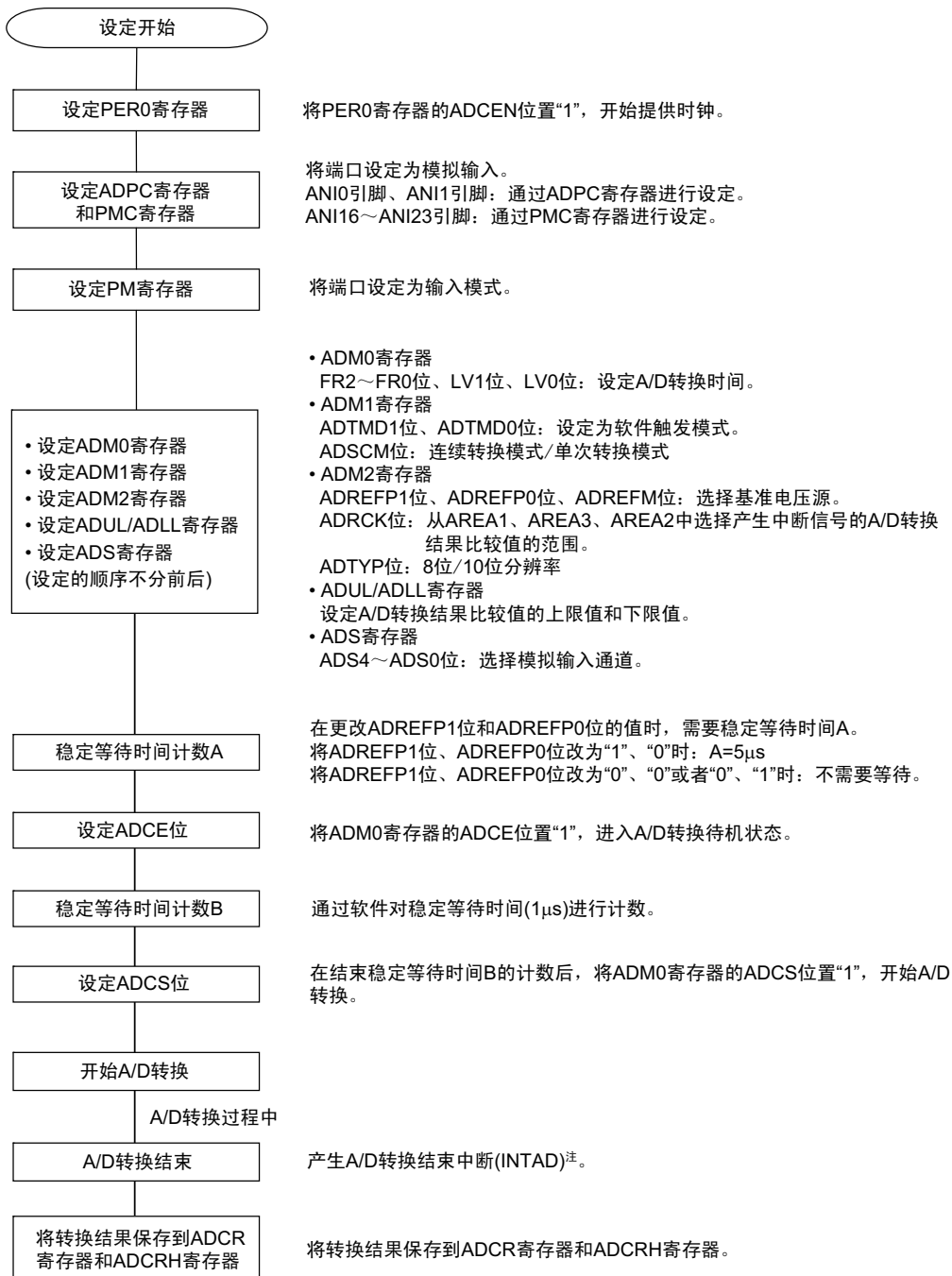
图 11-26 软件触发模式的设定
