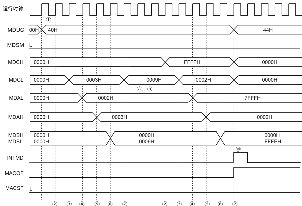
图 15-8 乘加运算（无符号）的时序图 ( 2 \times 3 + 3 = 9 \rightarrow 32767 \times 2 + 4294901762 = 0 (发生上溢))
