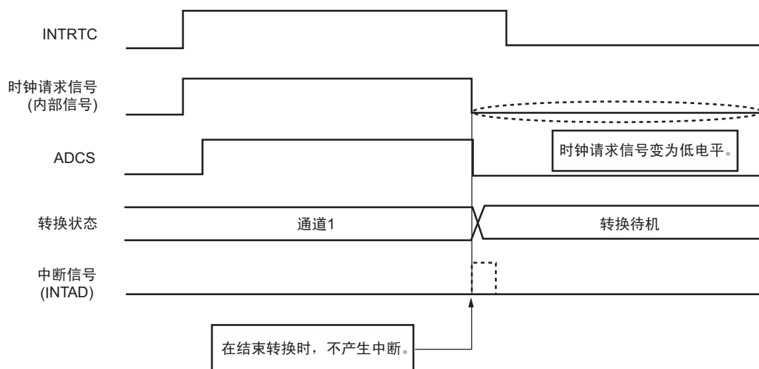
图 11-33 在 A/D 转换结束后不发生中断时的运行例子
