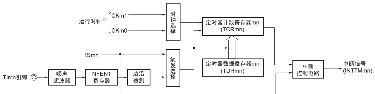
图 6-63 作为延迟计数器运行的框图
