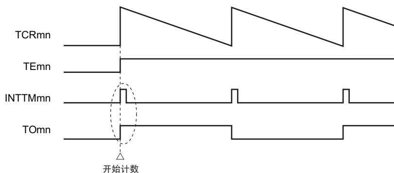
图 6-41 MDmn0 位为“1”的情况
