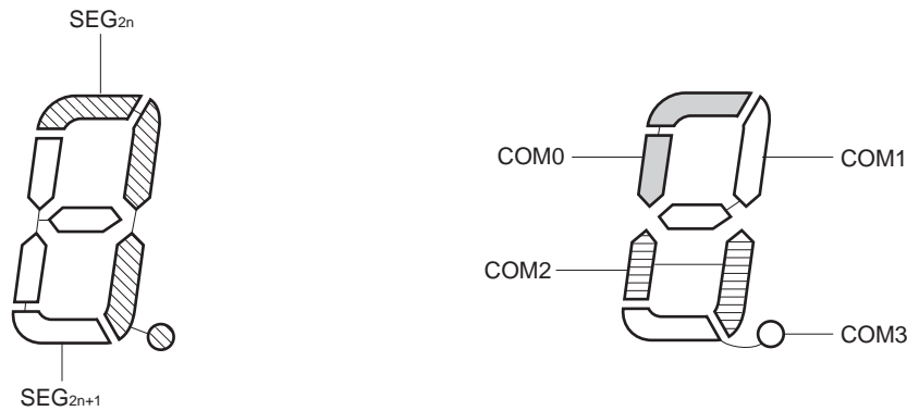
图 14-39 4 个时间片的 LCD 显示图形和电极连线
