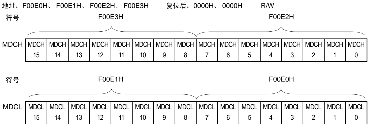
图 15-4 乘法数据寄存器 C (MDCH、MDCL) 的格式
