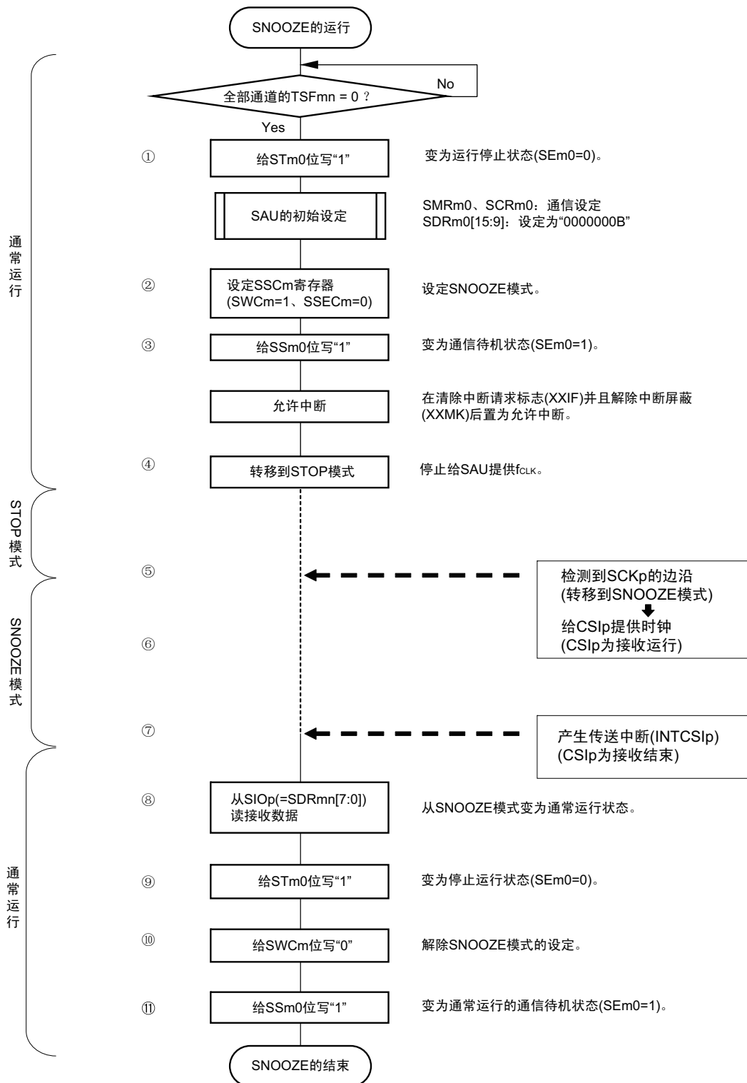
图 12-71 SNOOZE 模式运行（启动一次）的流程图
