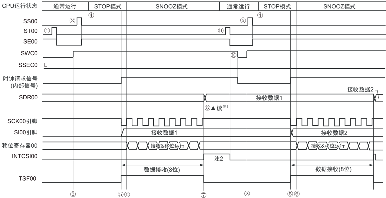
图 12-72 SNOOZE 模式运行（连续启动）的时序图（类型 1：DAPmn=0、CKPmn=0）
