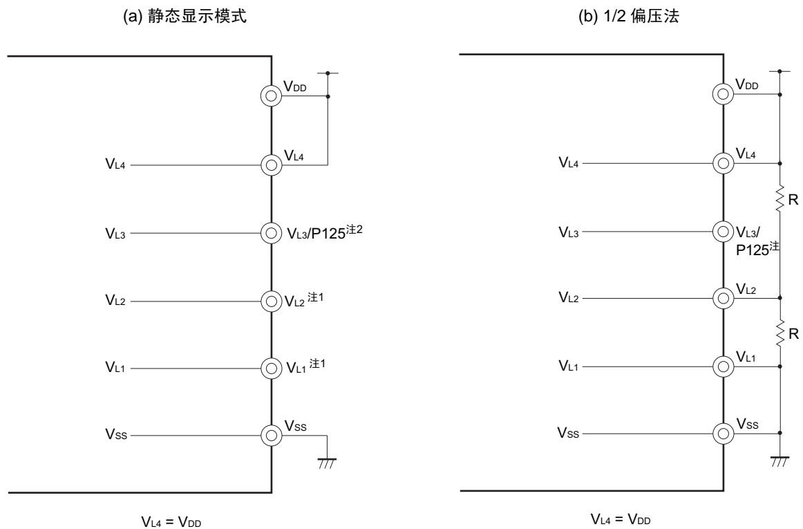
图 14-24 LCD 驱动电源的连接例子（外部电阻分割方式）(1/2)
