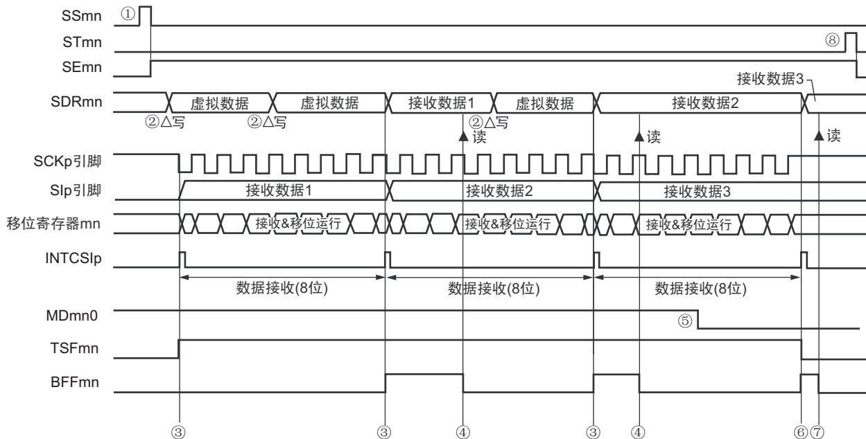
图 12-38 主控接收（连续接收模式）的时序图（类型 1：DAPmn=0、CKPmn=0）
