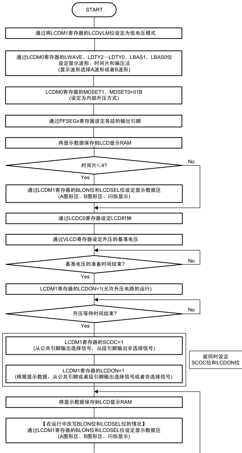
图 14-20 通常液晶波形时的内部升压方式的设定步骤
