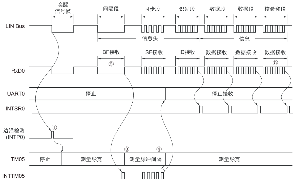
图 12-99 LIN 的接收操作
