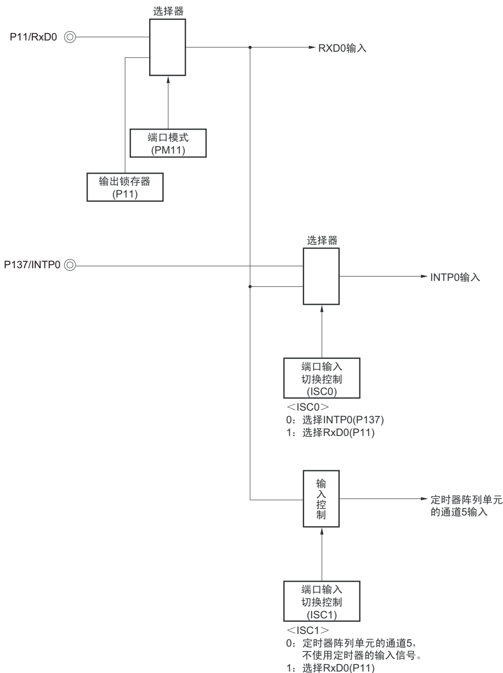
图 12-101 用于 LIN 接收操作的端口结构图（32、44、48 引脚产品的情况）
