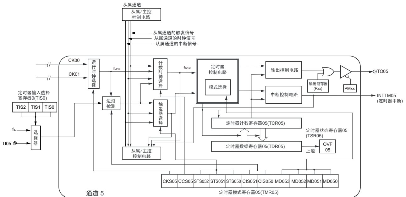
图 6-5 定时器阵列单元 0 的通道 5 的内部框图
