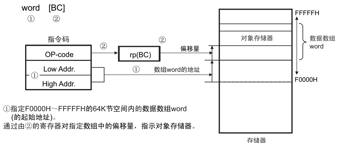
图 3-30 word[BC] 的例子
