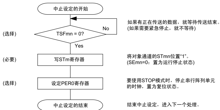
图 12-85 UART 接收的中止步骤
