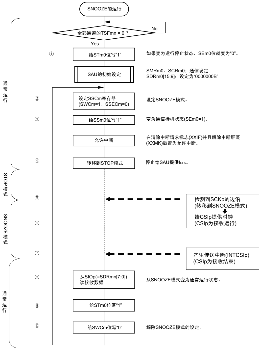
图 12-73 SNOOZE 模式运行（连续启动）的流程图
