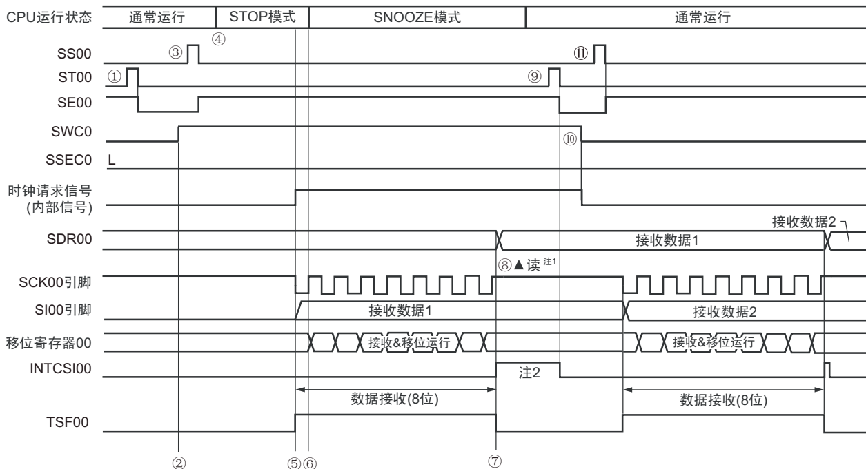
图 12-70 SNOOZE 模式运行（启动一次）的时序图（类型 1：DAPmn=0、CKPmn=0）
