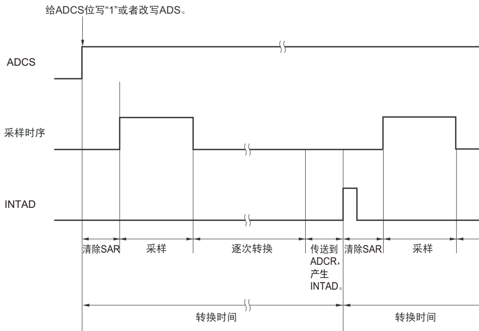
图 11-5 A/D 转换器的采样和 A/D 转换时序（以软件触发模式为例的情况）
