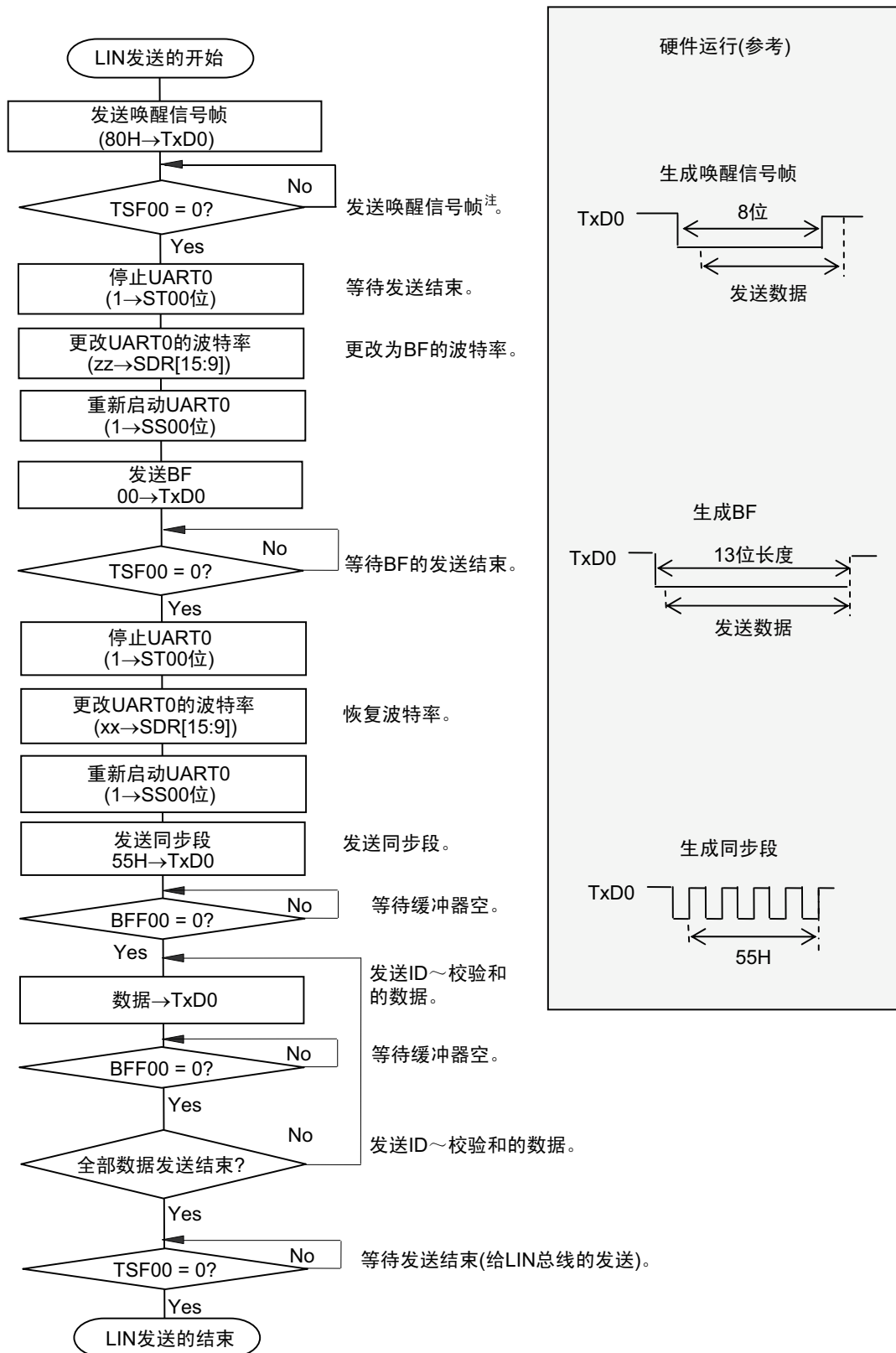
图 12-98 LIN 发送的流程图
