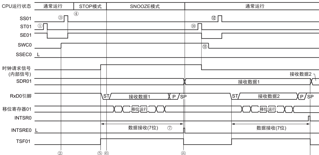
图 12-90 SNOOZE 模式运行（异常运行①）的时序图
