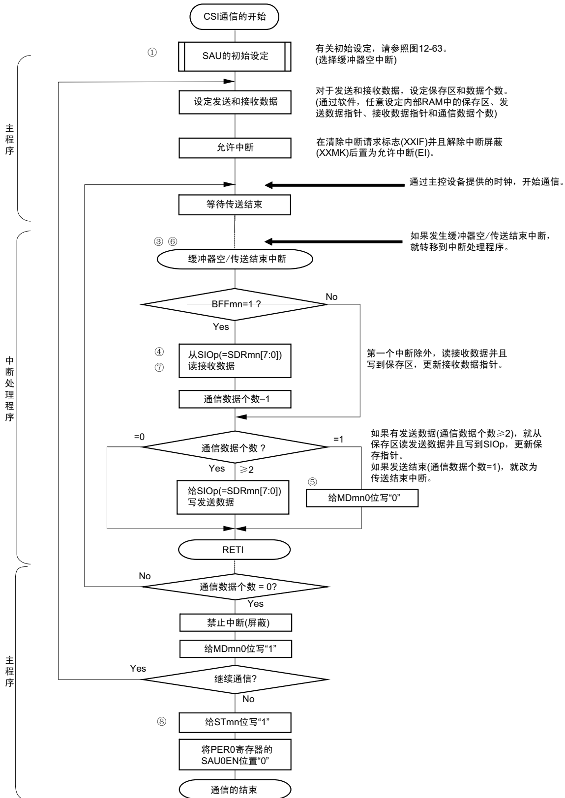
图 12-69 从属发送和接收（连续发送和接收模式）的流程图
