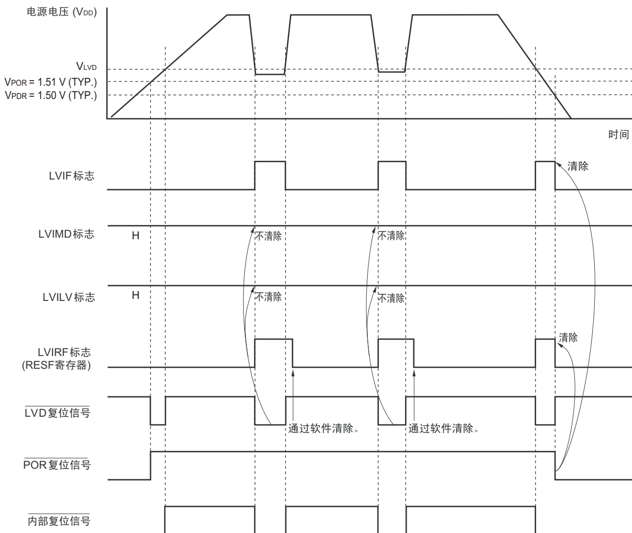
图 22-4 内部复位信号的发生时序（选项字节的 LVIMDS1、LVIMDS0=1、1）
