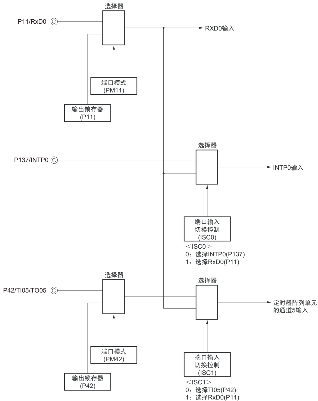
图 12-102 用于 LIN 接收操作的端口结构图（52、64 引脚产品的情况）
