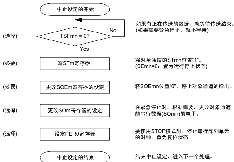
图 12-50 从属发送的中止步骤
