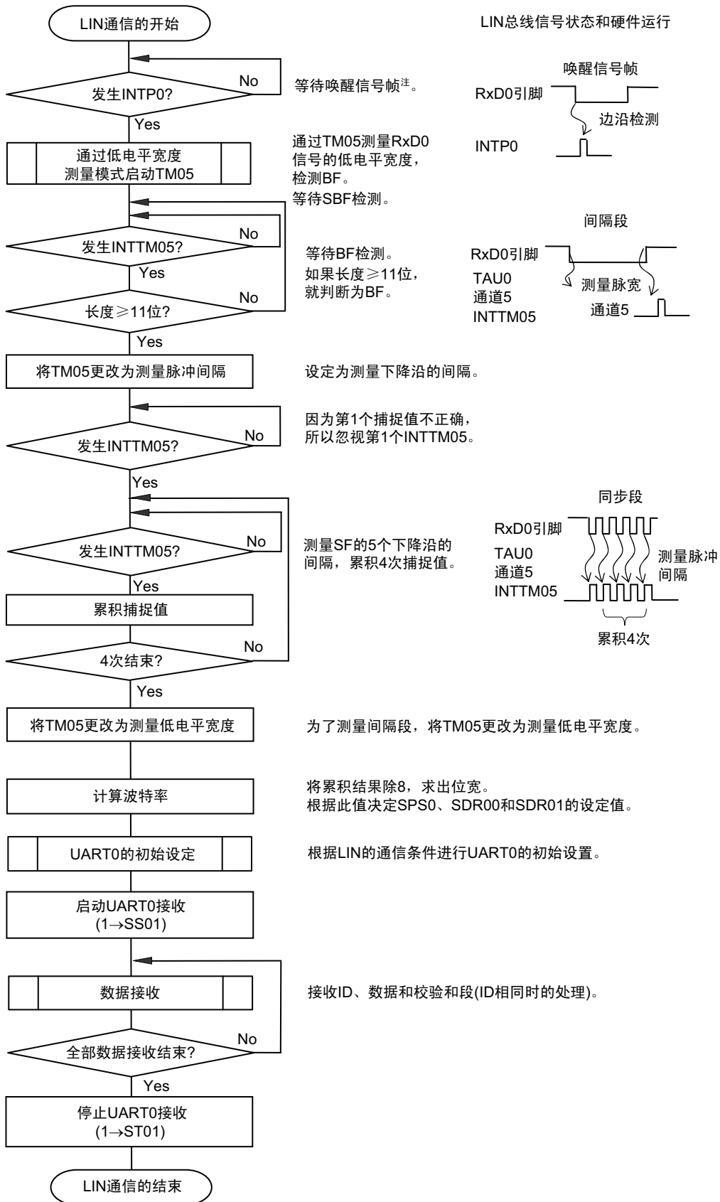
图 12-100 LIN 接收的流程图
