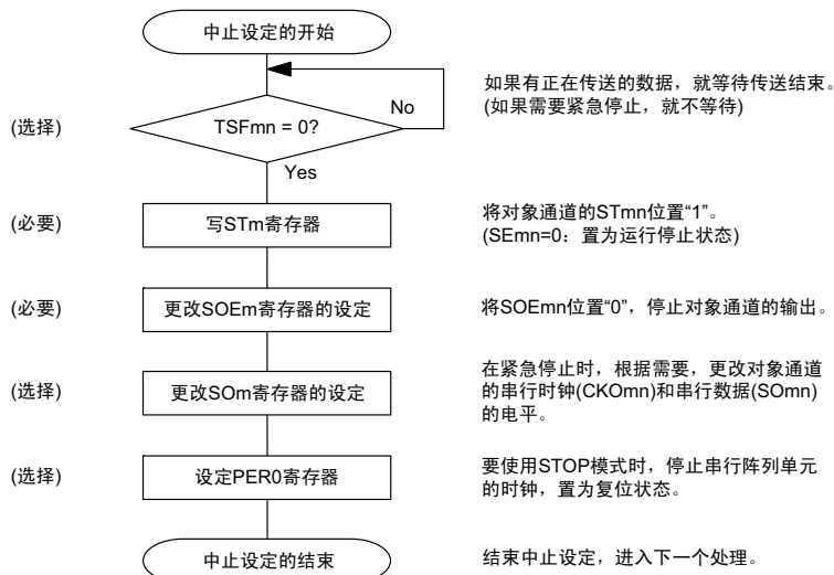
图 12-42 主控发送和接收的中止步骤
