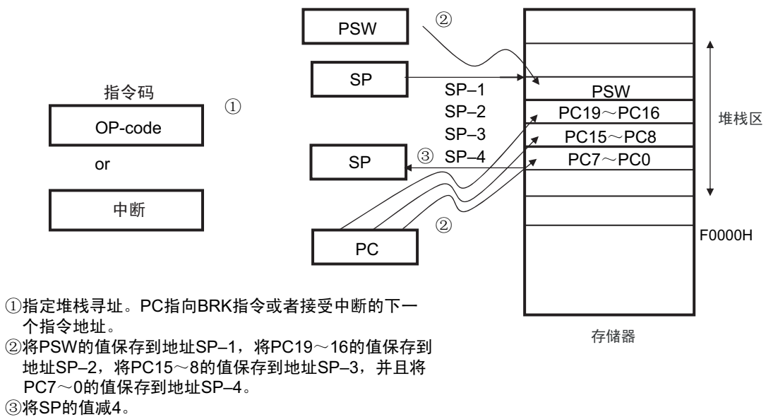
图 3-40 中断、BRK 的例子
