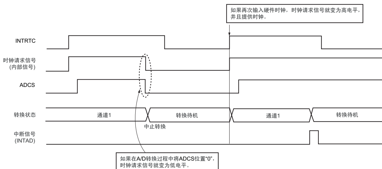
图 11-34 中止 A/D 转换 / 重新开始 A/D 转换时的运行例子
