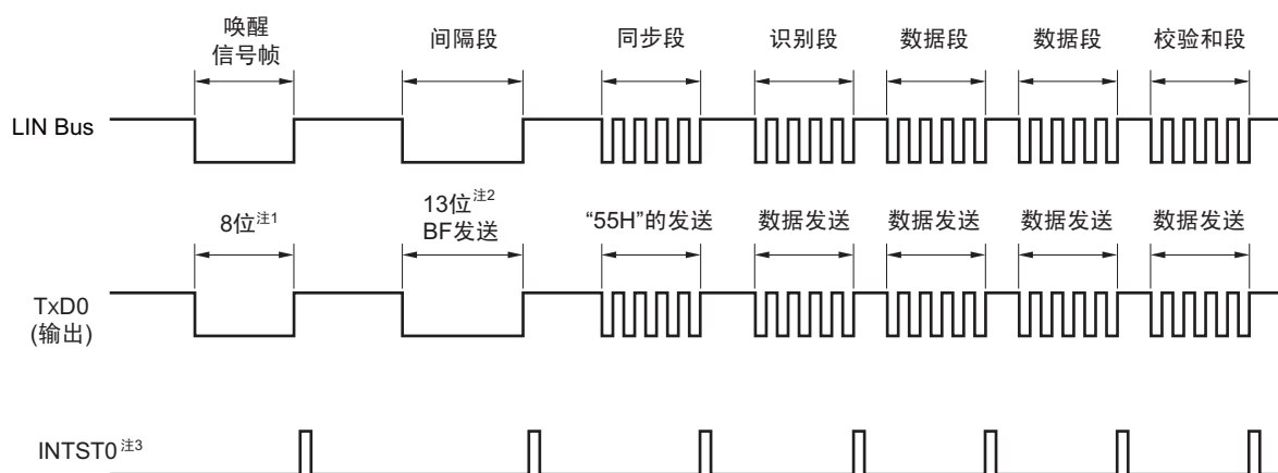
图 12-97 LIN 的主控发送操作
