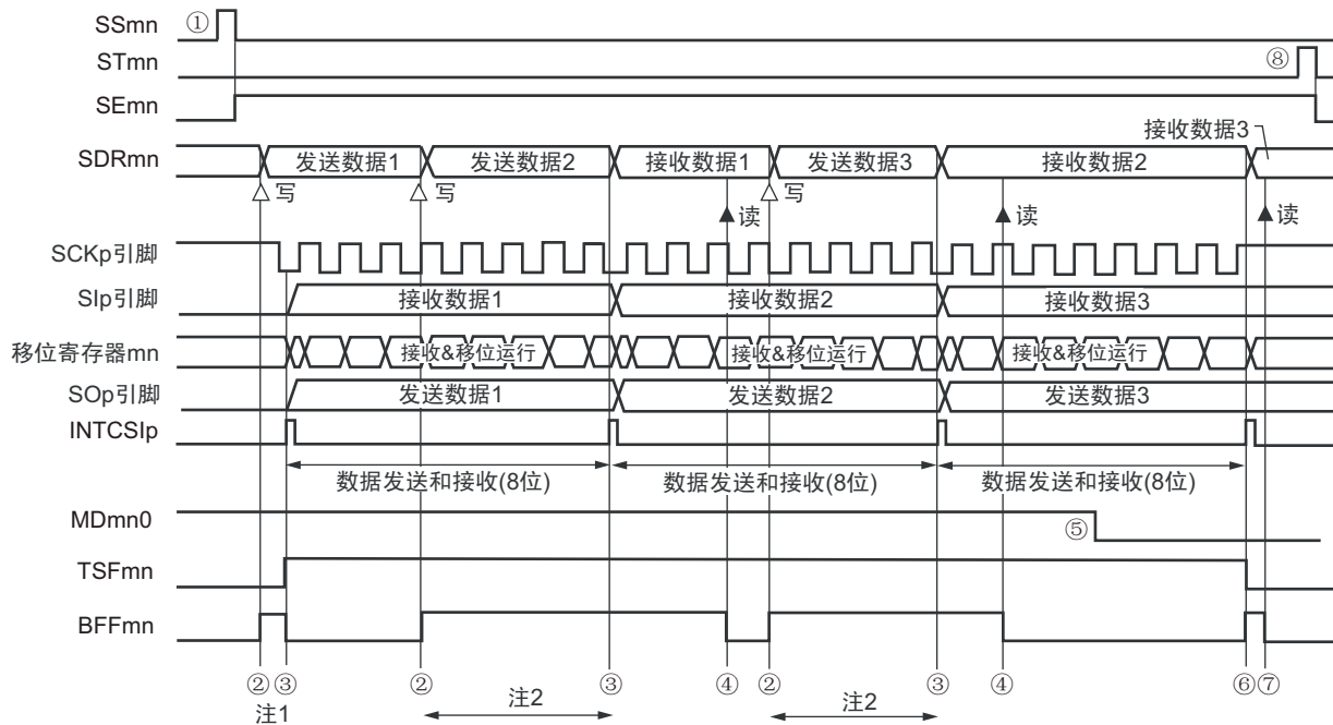
图 12-68 从属发送和接收（连续发送和接收模式）的时序图（类型 1：DAPmn=0、CKPmn=0）
