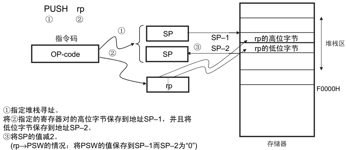
图 3-36 PUSH rp 的例子
