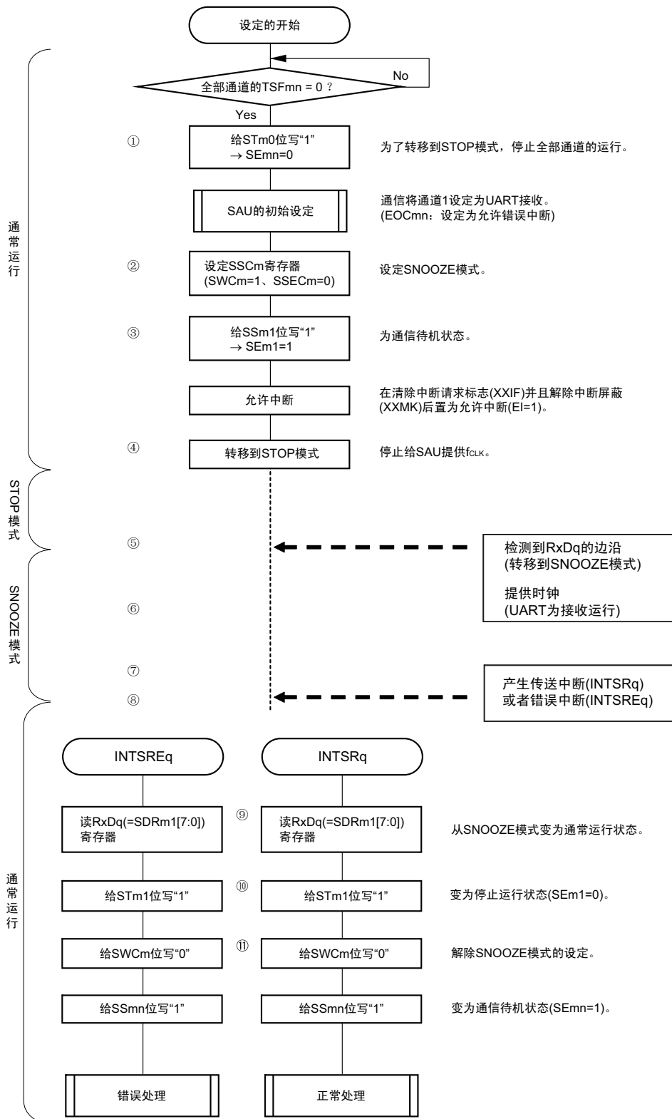
图 12-91 SNOOZE 模式运行（通常运行 / 异常运行①）的流程图
