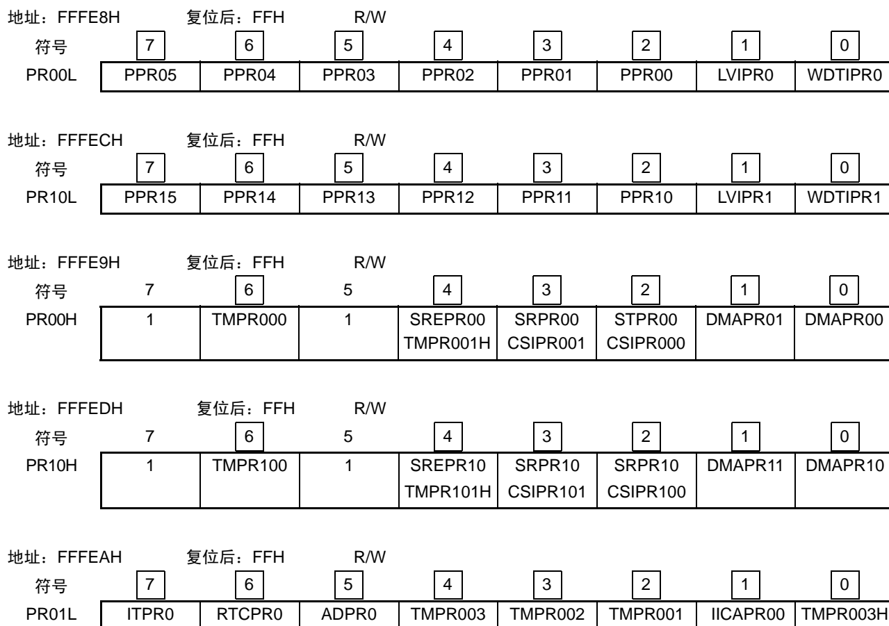
图 17-4 优先级指定标志寄存器 (PR00L、PR00H、PR01L、PR01H、PR02L、PR10L、PR10H、PR11L、PR11H、PR12L) 的格式 (64 引脚产品) (1/2)
