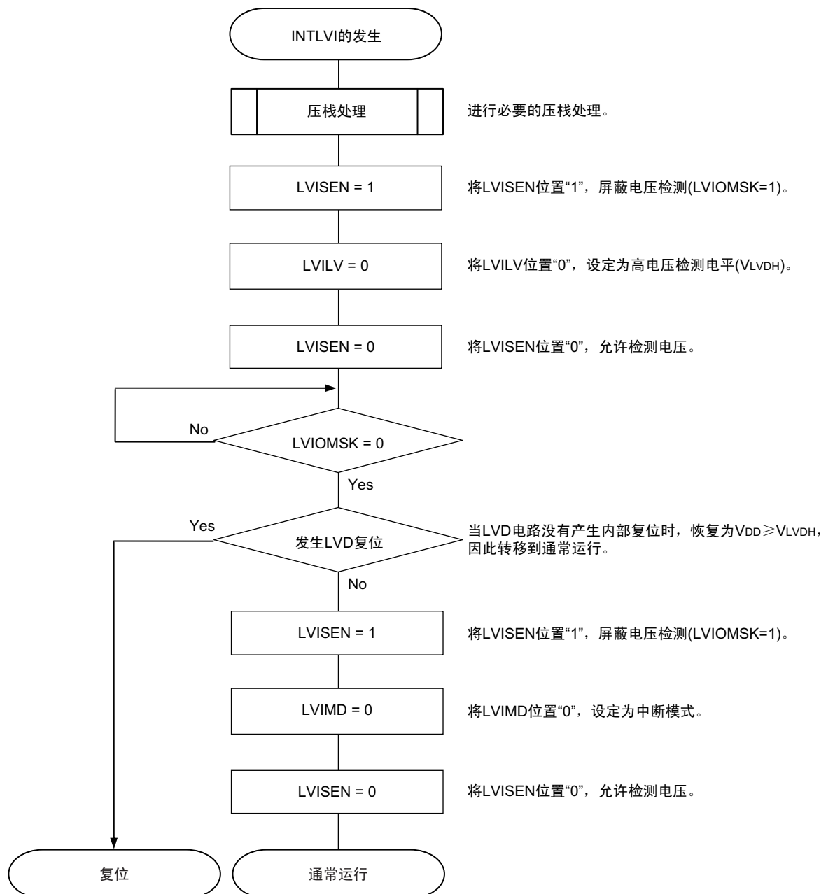
图 22-7 工作电压的确认 / 复位的设定步骤
