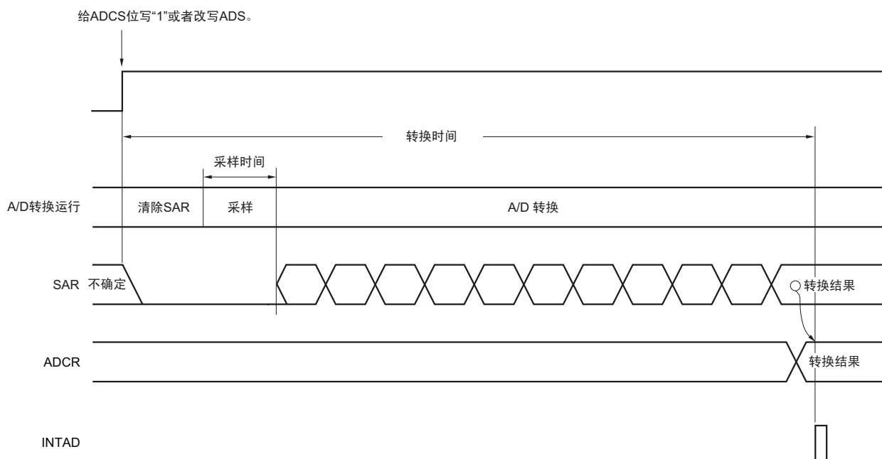
图 11-18 A/D 转换器的转换运行（软件触发模式的情况）
