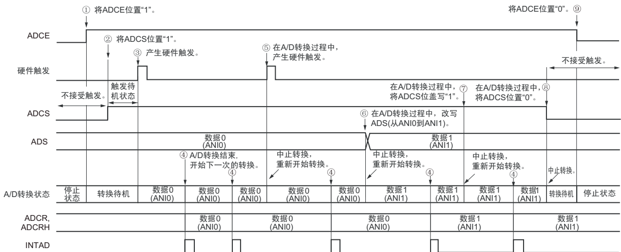
图 11-22 硬件触发无等待模式（连续转换模式）的运行时序例子
