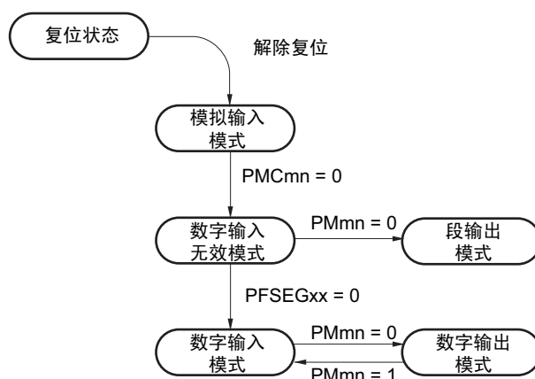
图 14-14 ANIxx/SEGxx/ 端口引脚功能的状态转移图
