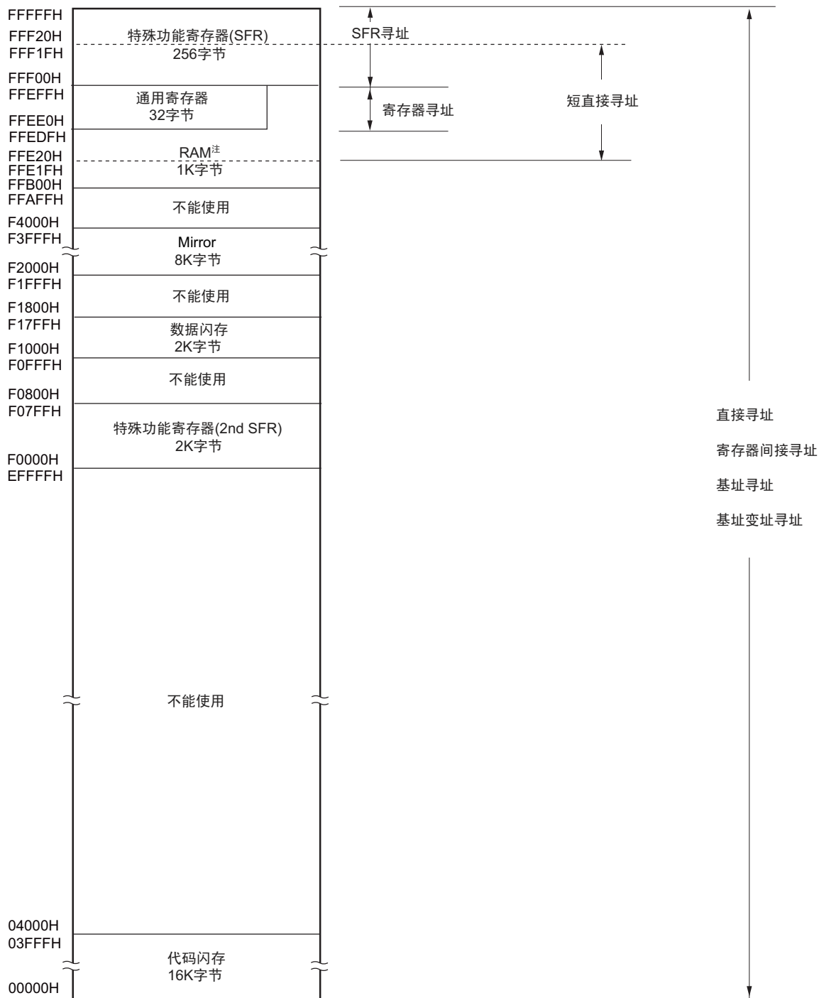
图 3-6 数据存储器和寻址的对应 (R5F10RxA (x=B、F、G、J、L))
