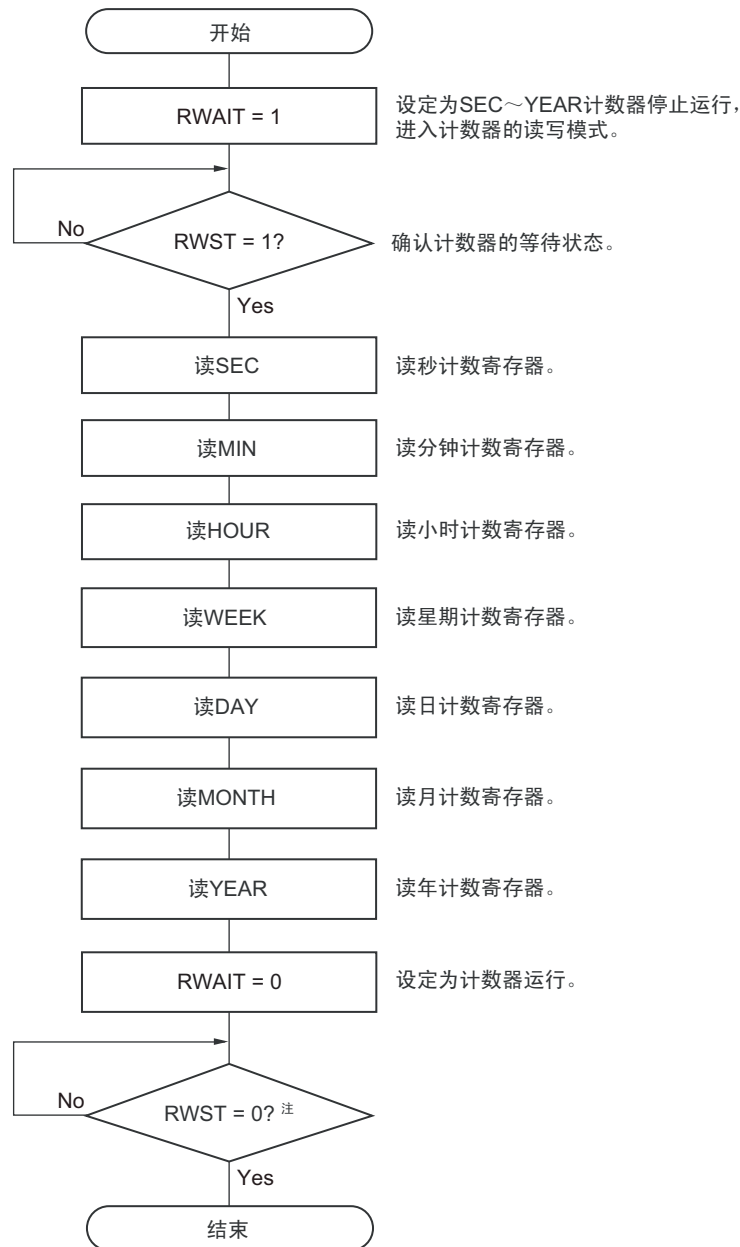
图 7-19 实时时钟计数器的读操作步骤
