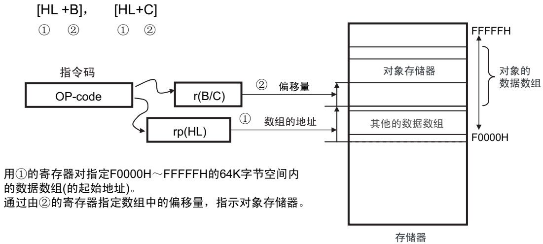
图 3-35 ES:[HL+B]、ES:[HL+C] 的例子
