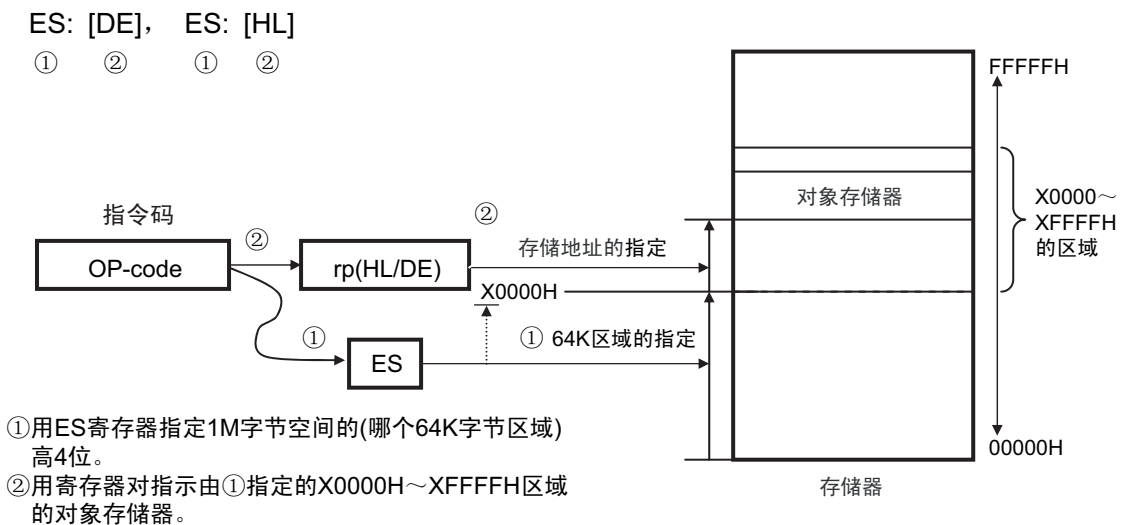
图 3-26 ES:[DE]、ES:[HL] 的例子
