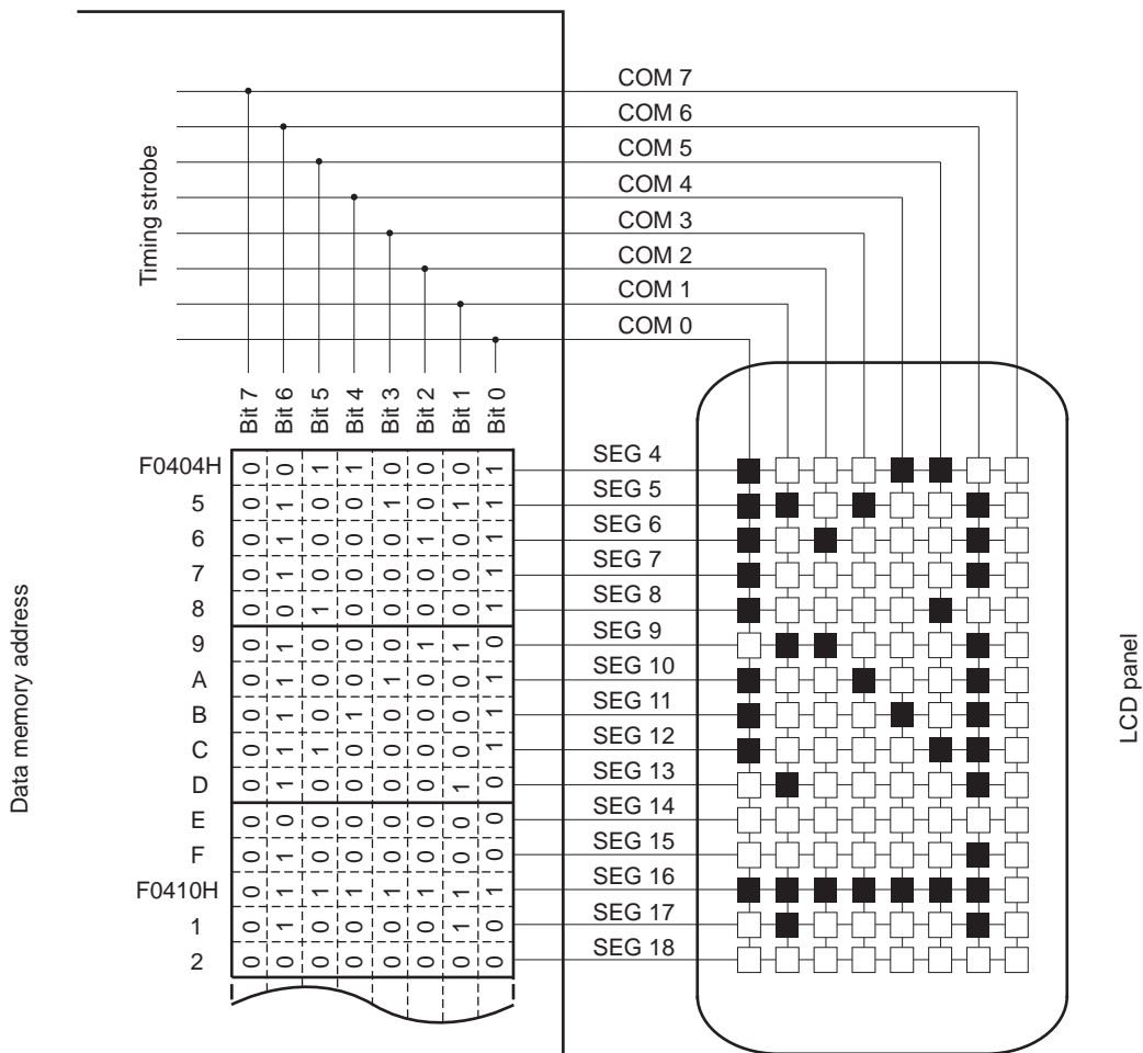
图 14-43 8 个时间片的 LCD 显示屏的连线例子
