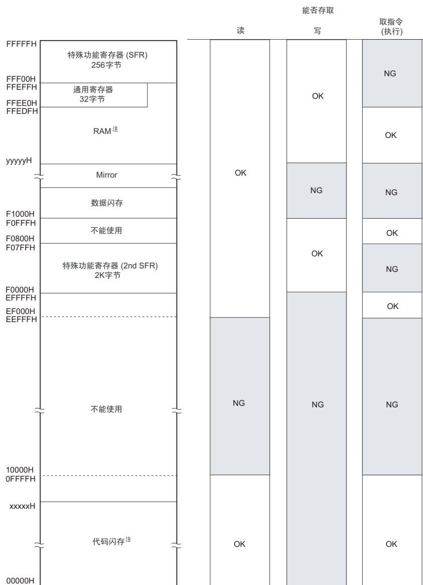
图 23-10 非法存取检测空间
