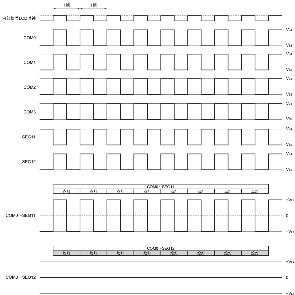
图 14-31 SEG11、SEG12 和 COM0 的静态 LCD 驱动波形例子
