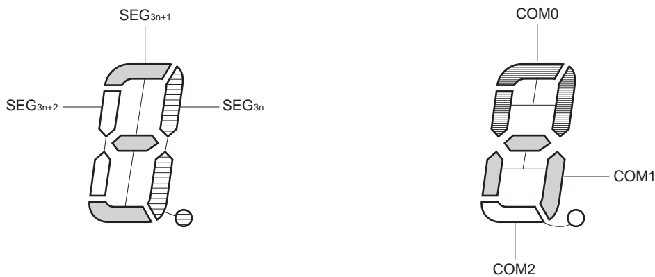
图 14-35 3 个时间片的 LCD 显示图形和电极连线
