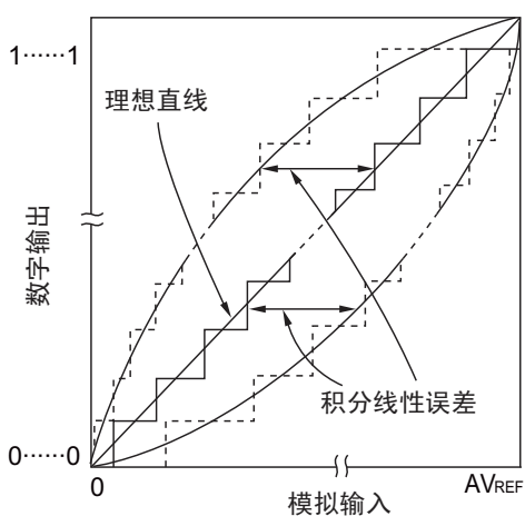
图 11-39 积分线性误差
