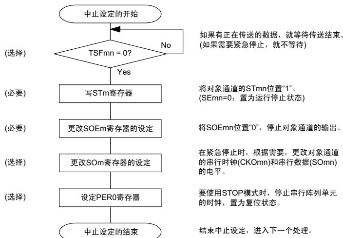
图 12-26 主控发送的中止步骤
