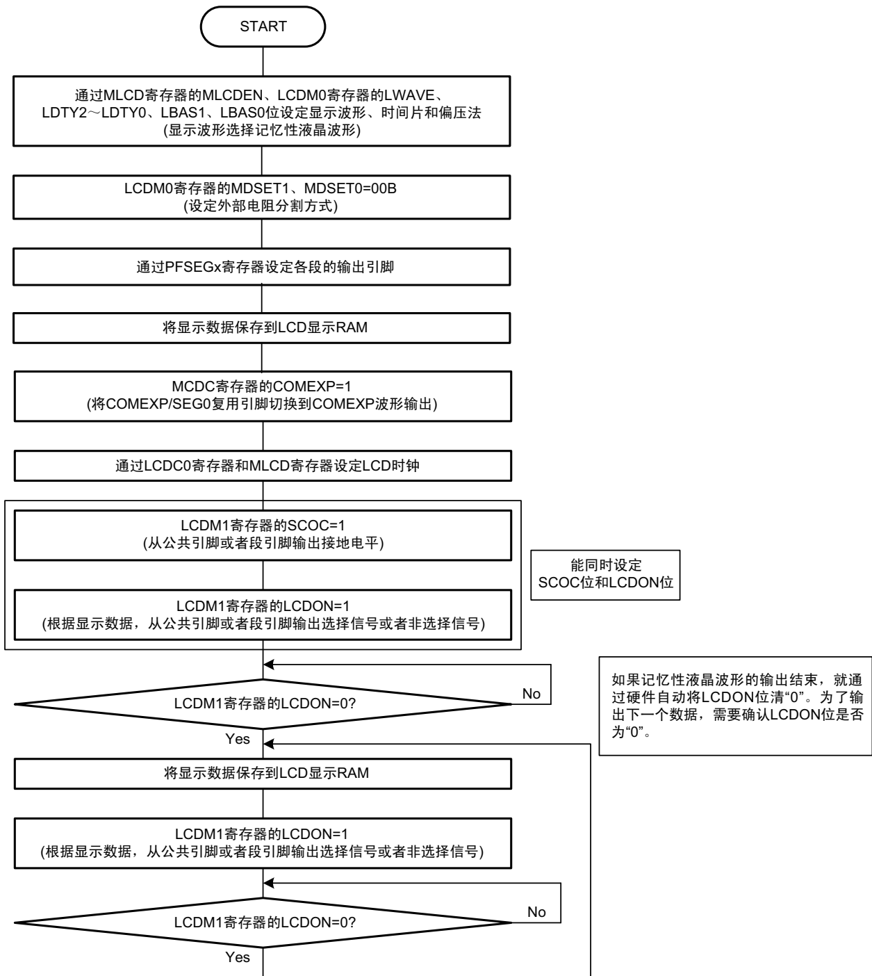
图 14-22 记忆性液晶波形时的外部电阻分割方式的设定步骤
