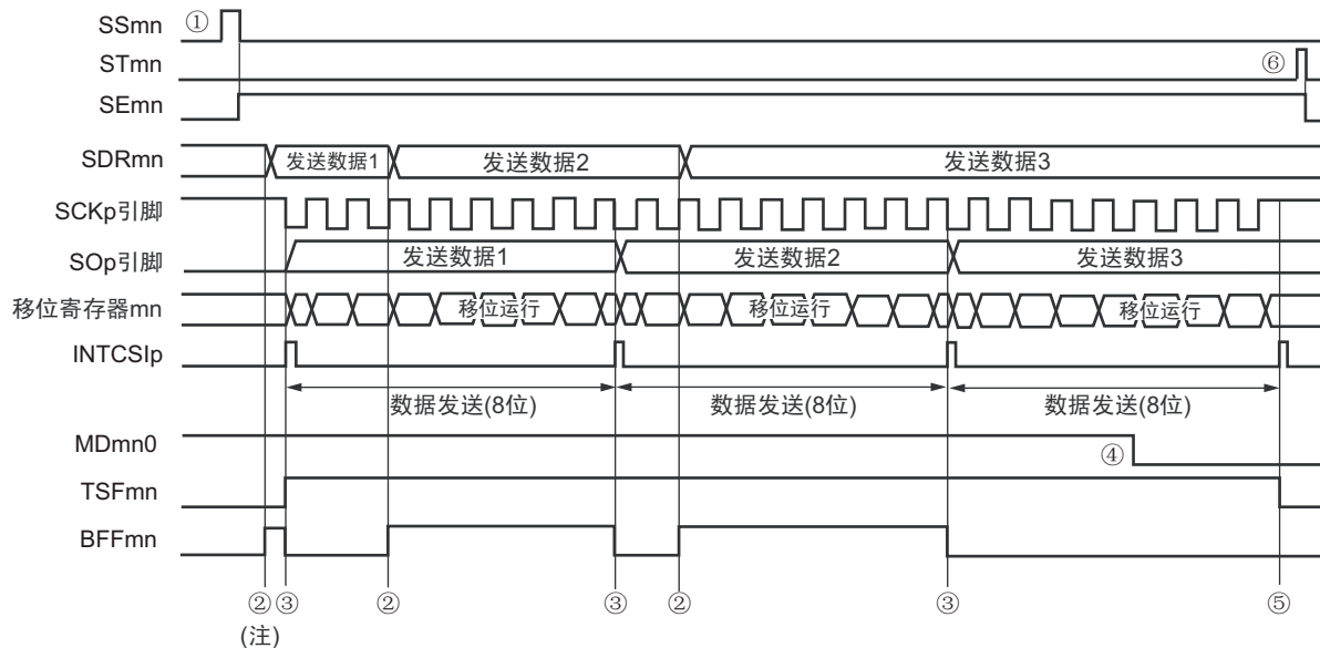
图 12-30 主控发送（连续发送模式）的时序图（类型 1：DAPmn=0、CKPmn=0）
