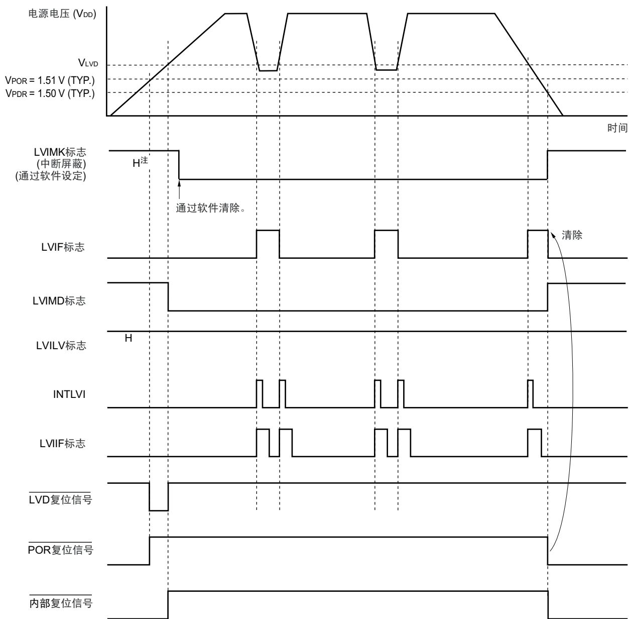
图 22-5 中断信号的发生时序 (选项字节的 LVIMDS1、LVIMDS0=0、1)
