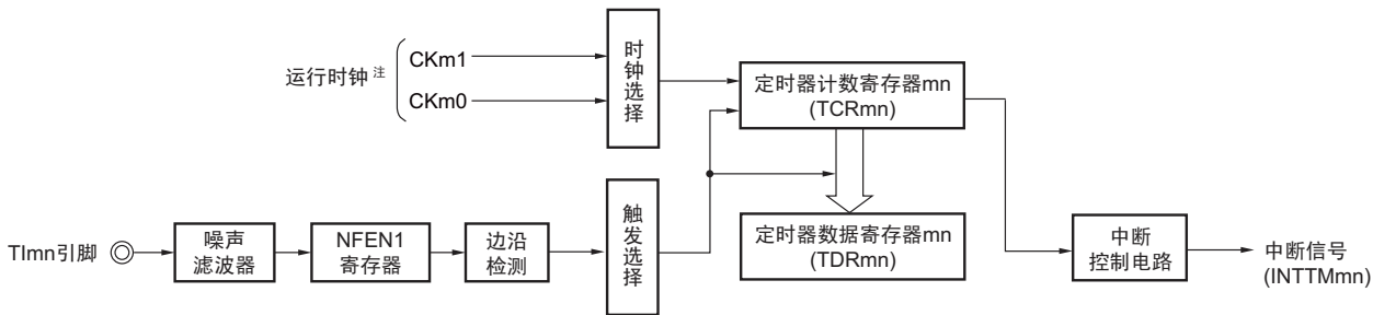
图 6-59 作为输入信号高 / 低电平宽度测量运行的框图
