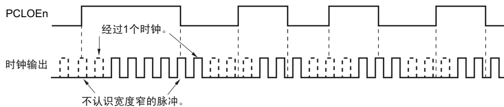
图 9-5 遥控输出的应用例子
