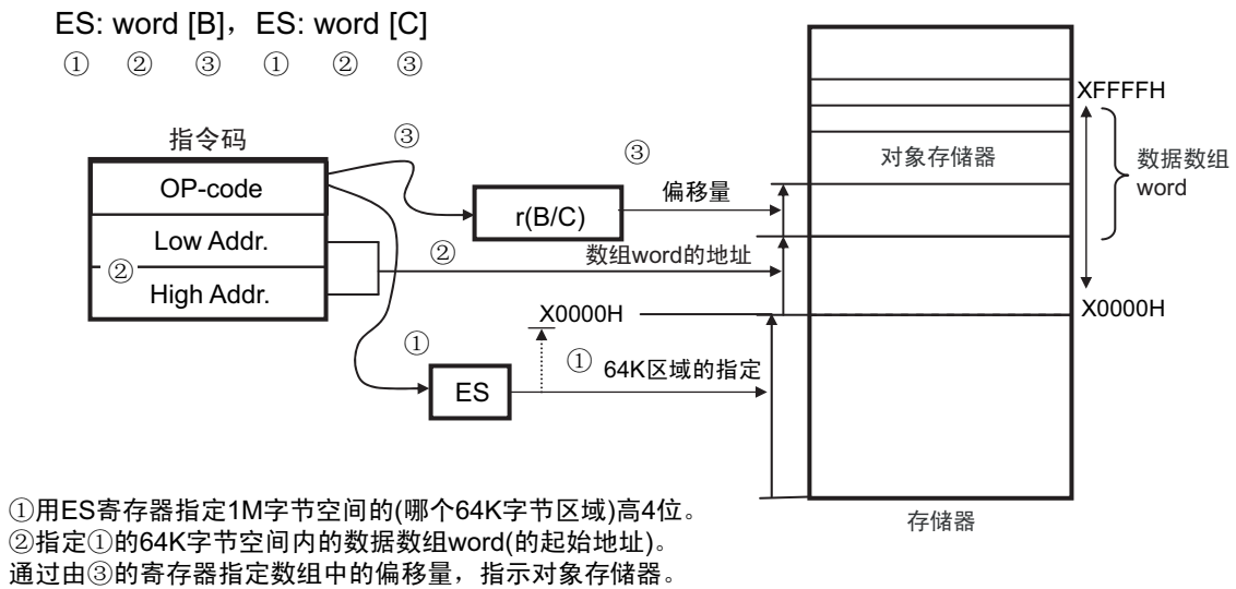
图 3-32 ES:word[B]、ES:word[C] 的例子
