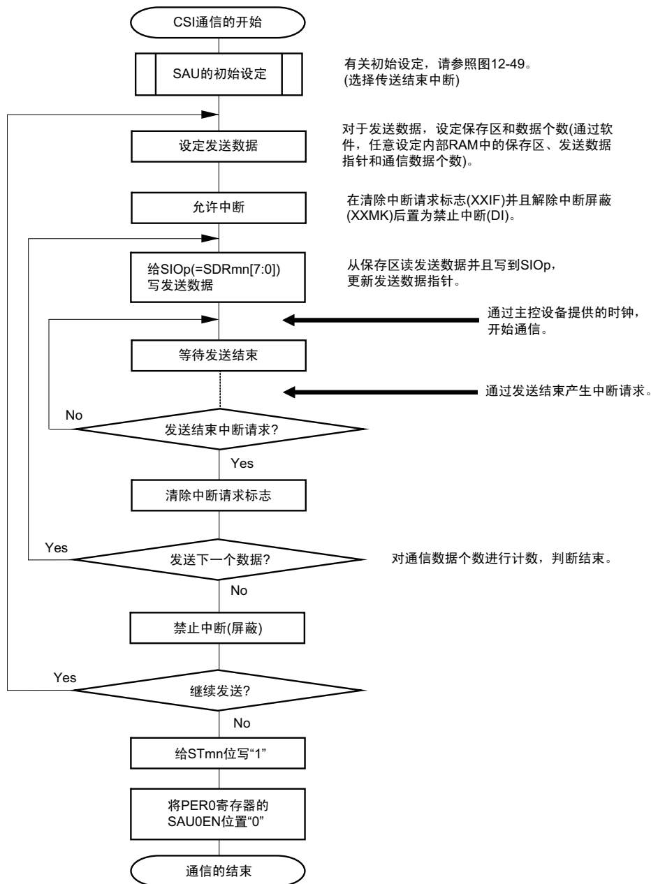
图 12-53 从属发送（单次发送模式）的流程图
