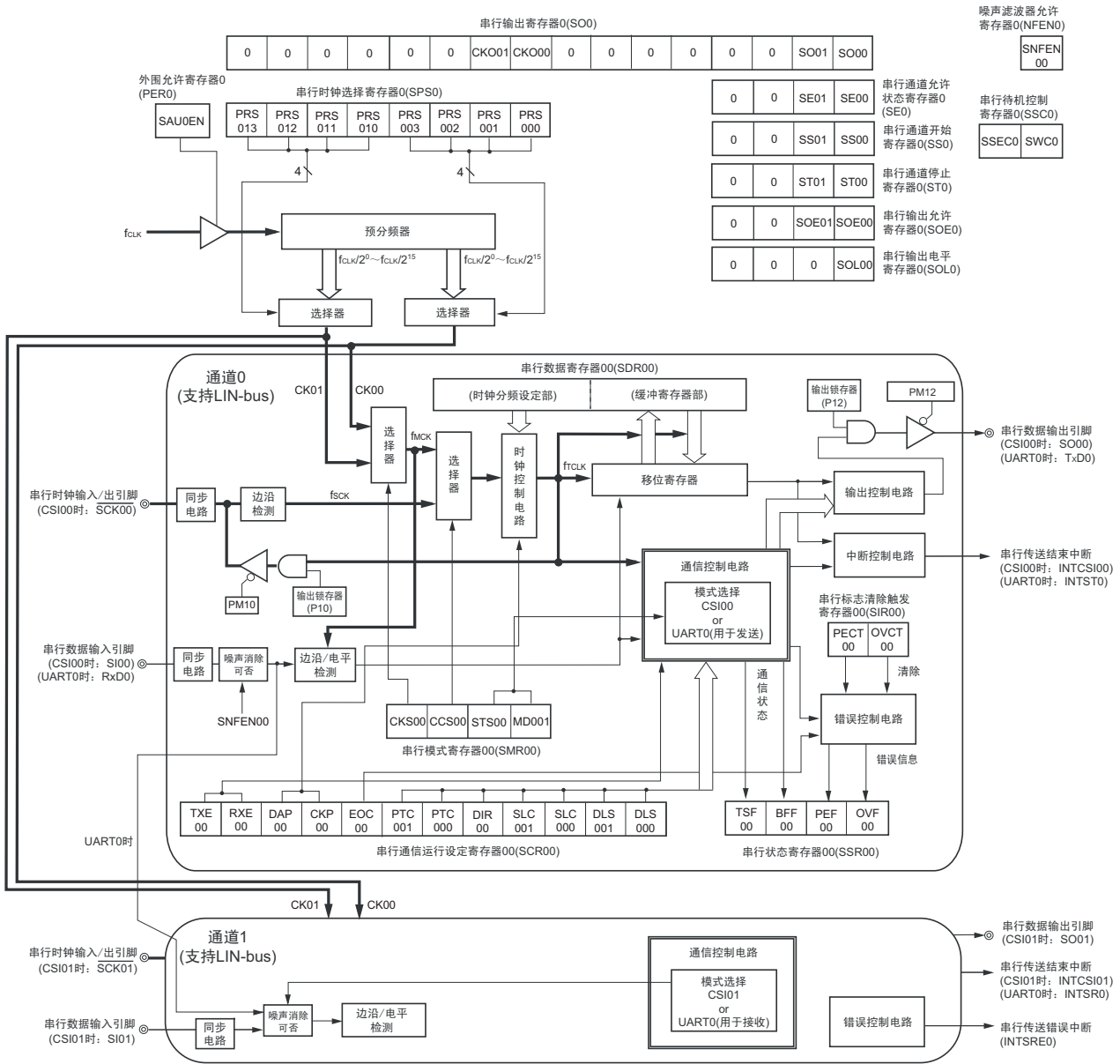
图 12-1 串行阵列单元的框图
