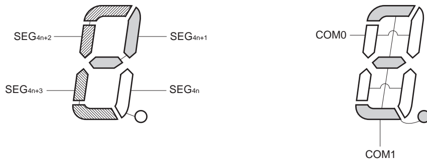
图 14-32 2 个时间片的 LCD 显示图形和电极连线
