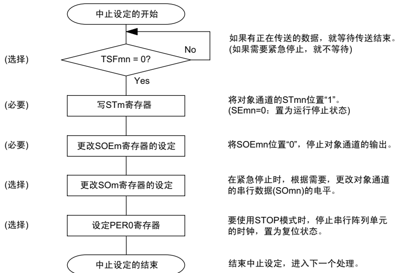
图 12-64 从属发送和接收的中止步骤
