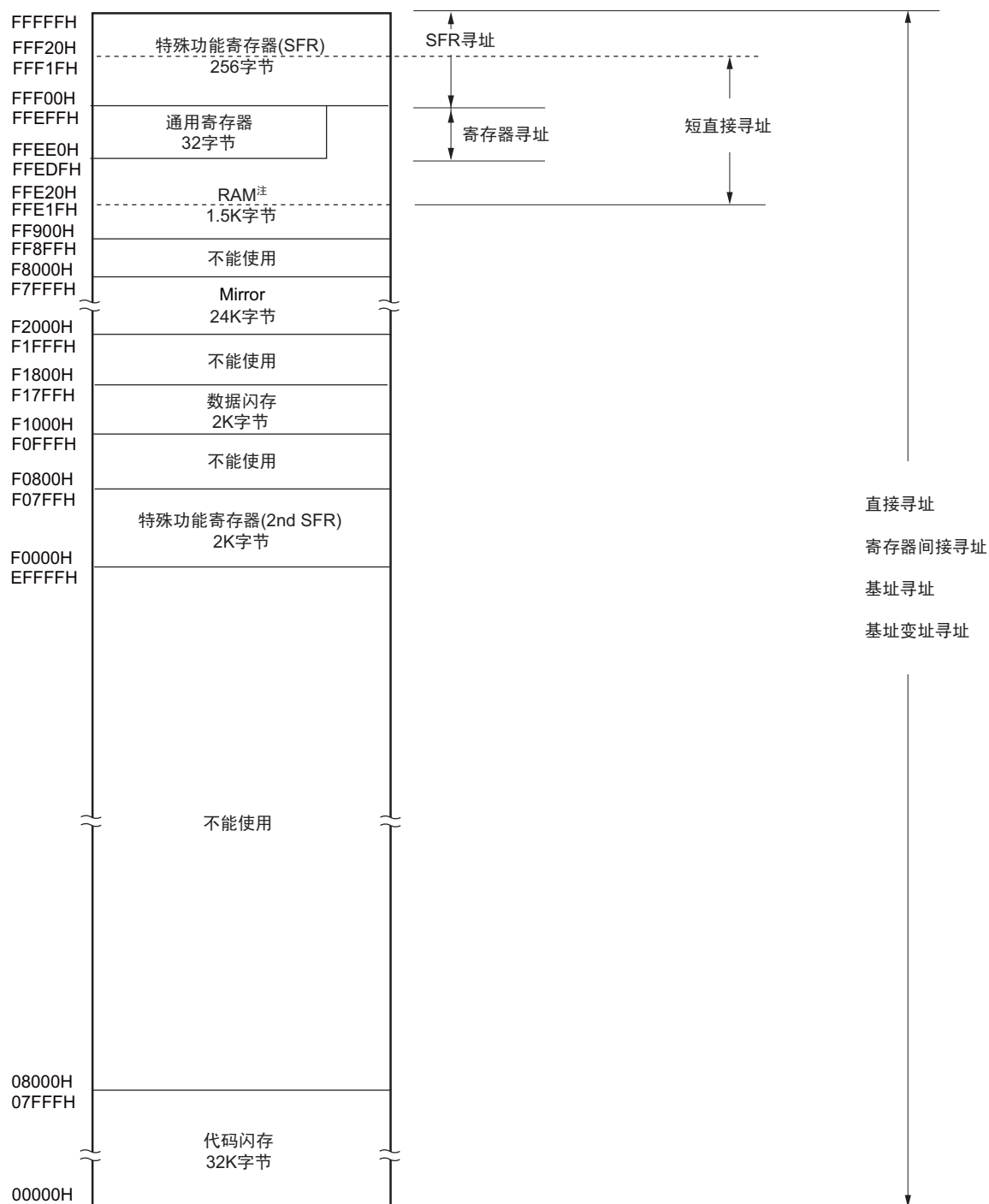
图 3-7 数据存储器和寻址的对应 (R5F10RxC (x=B、F、G、J、L))
