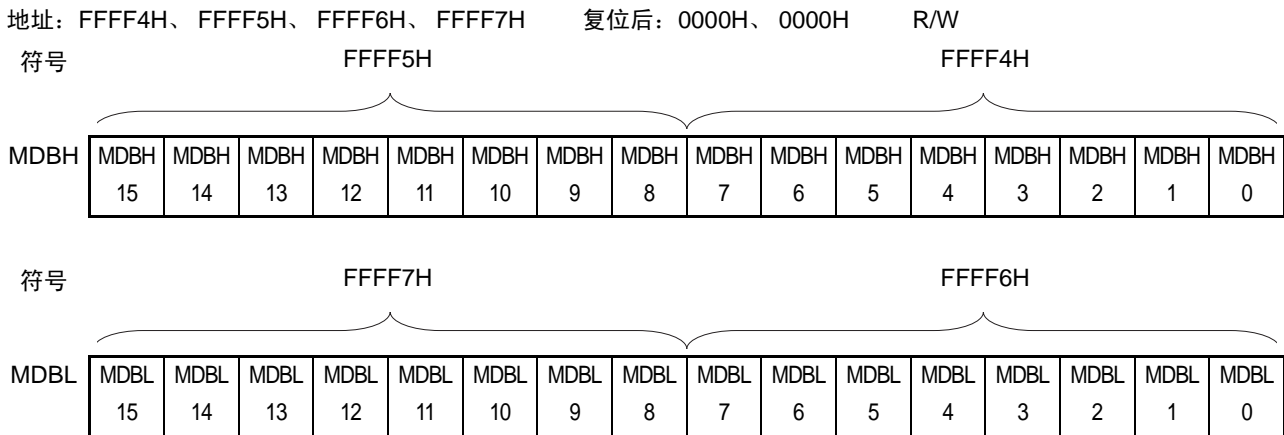
图 15-3 乘除数据寄存器 B (MDBH、MDBL) 的格式
