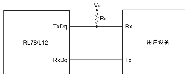
UART 模式的连接图 (不同电位的通信)
