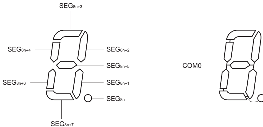
图 14-29 静态 LCD 的显示图形和电极连线
