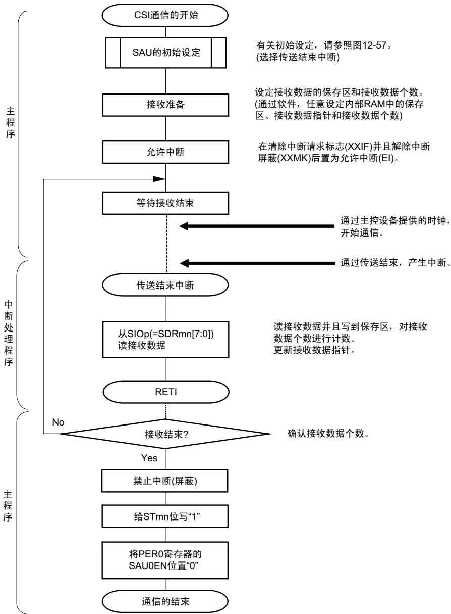
图 12-61 从属接收（单次接收模式）的流程图
