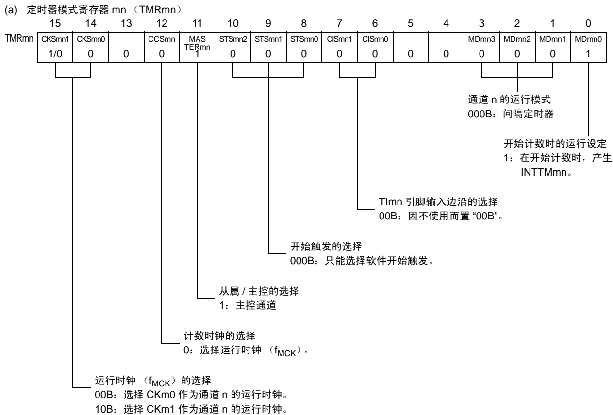
图 6-74 PWM 功能时（主控通道）的寄存器设定内容例子
