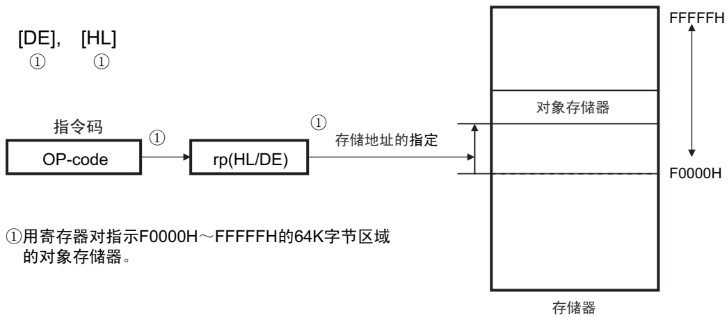
图 3-26 ES:[DE]、ES:[HL] 的例子
