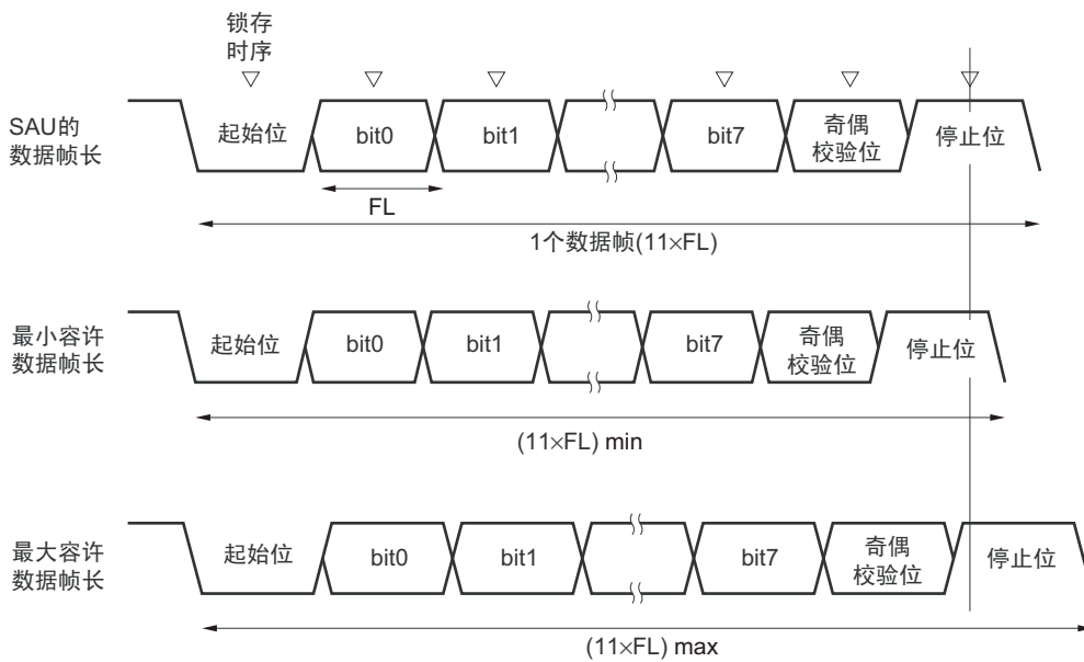
图 12-94 接收时的波特率容许范围 (1 个数据帧的帧长 =11 位的情况)
