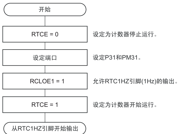
图 7-22 1Hz 输出的设定步骤
