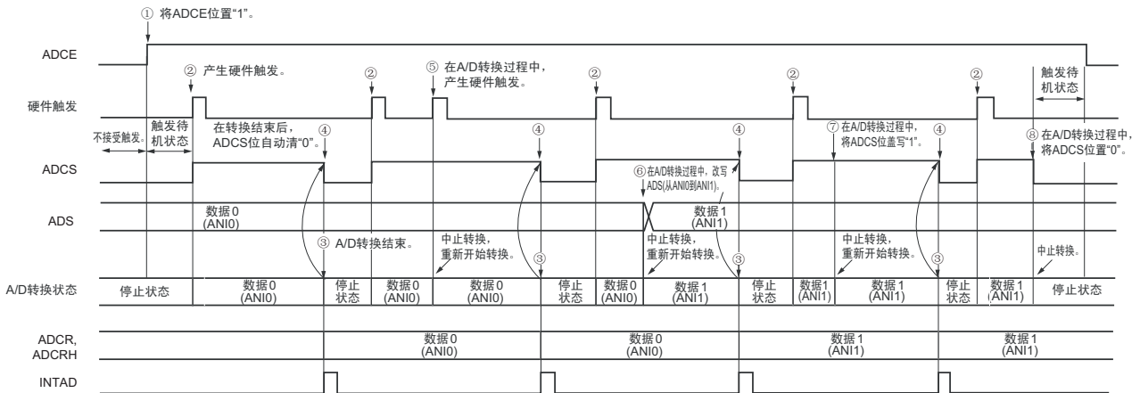
图 11-25 硬件触发等待模式（单次转换模式）的运行时序例子
