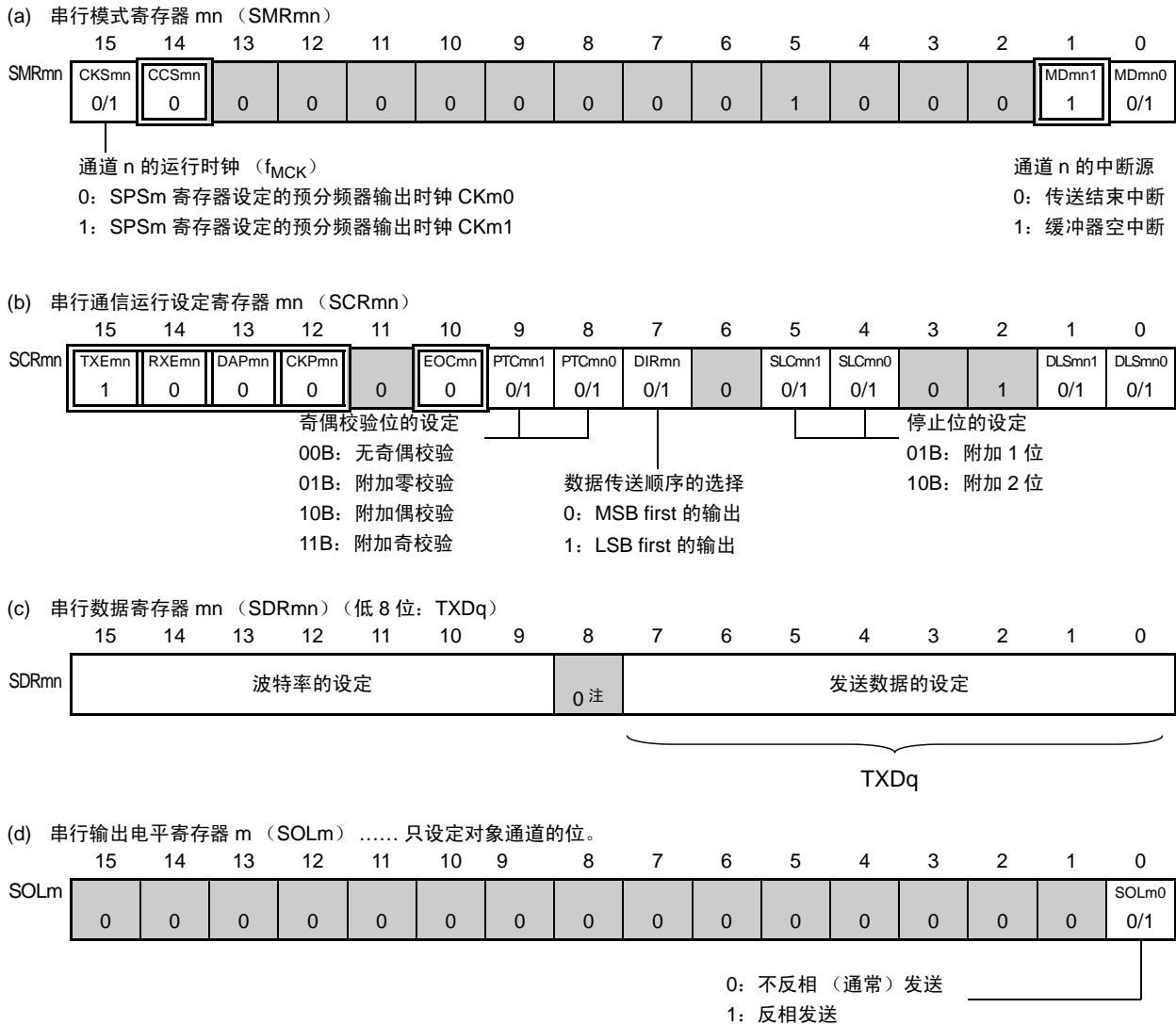
图 12-75 UART (UART0) 的 UART 发送时的寄存器设定内容例子 (1/2)
