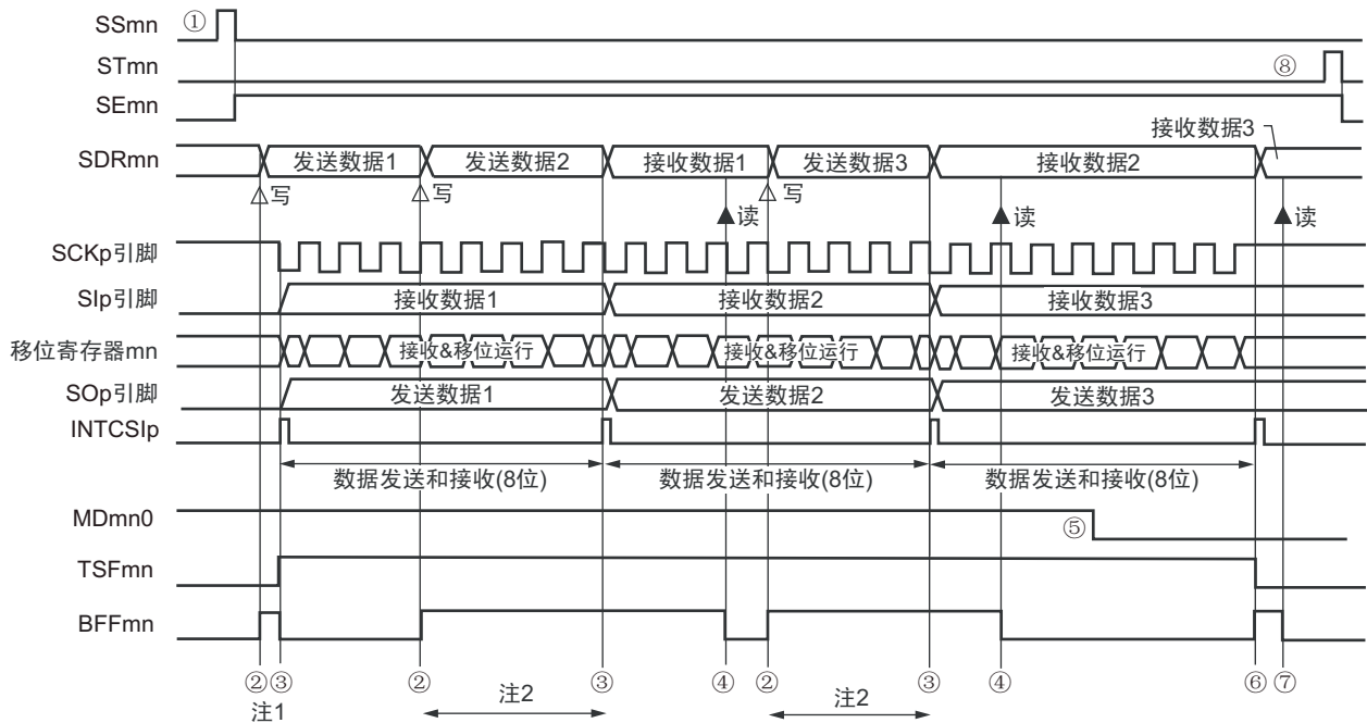
图 12-46 主控发送和接收（连续发送和接收模式）的时序图（类型 1：DAPmn=0、CKPmn=0）
