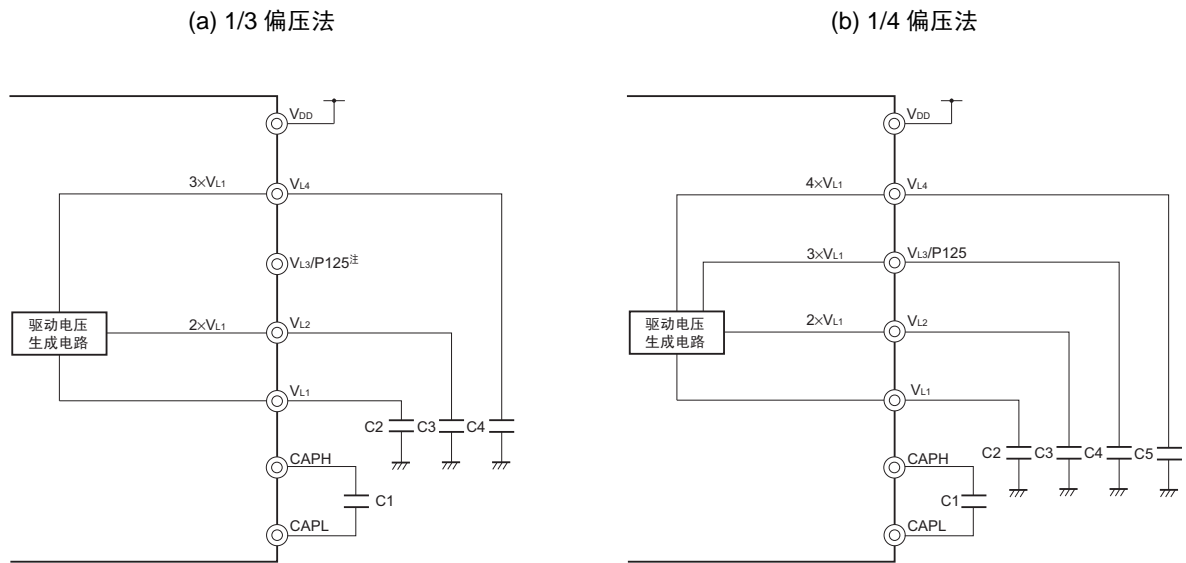
图 14-25 LCD 驱动电源的连接例子 (内部升压方式)
