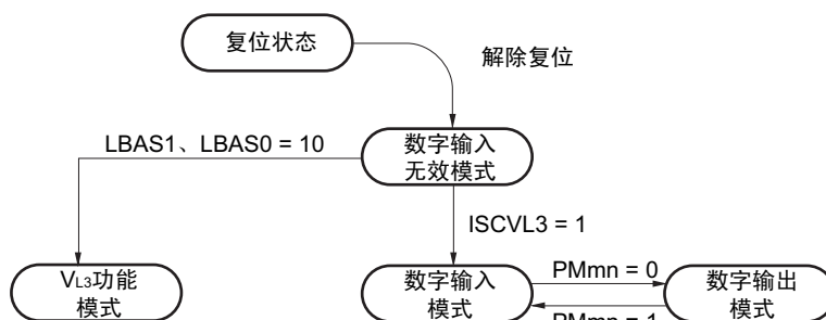
图 4-13 V_{L3}/P125 引脚功能的状态转移图
