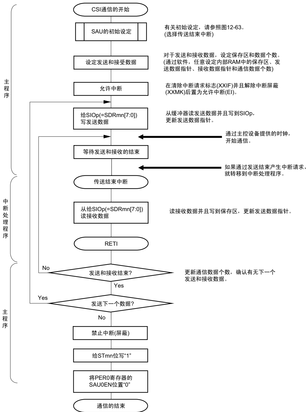
图 12-67 从属发送和接收（单次发送和接收模式）的流程图
