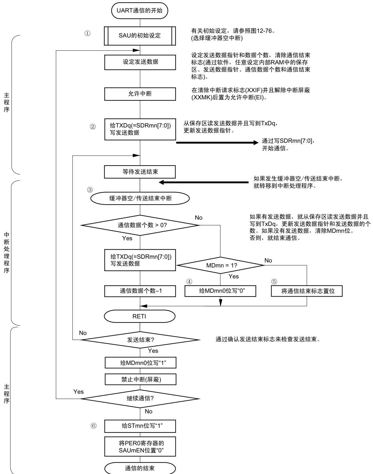
图 12-82 UART 发送（连续发送模式）的流程图
