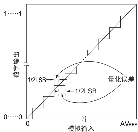
图 11-36 量化误差
