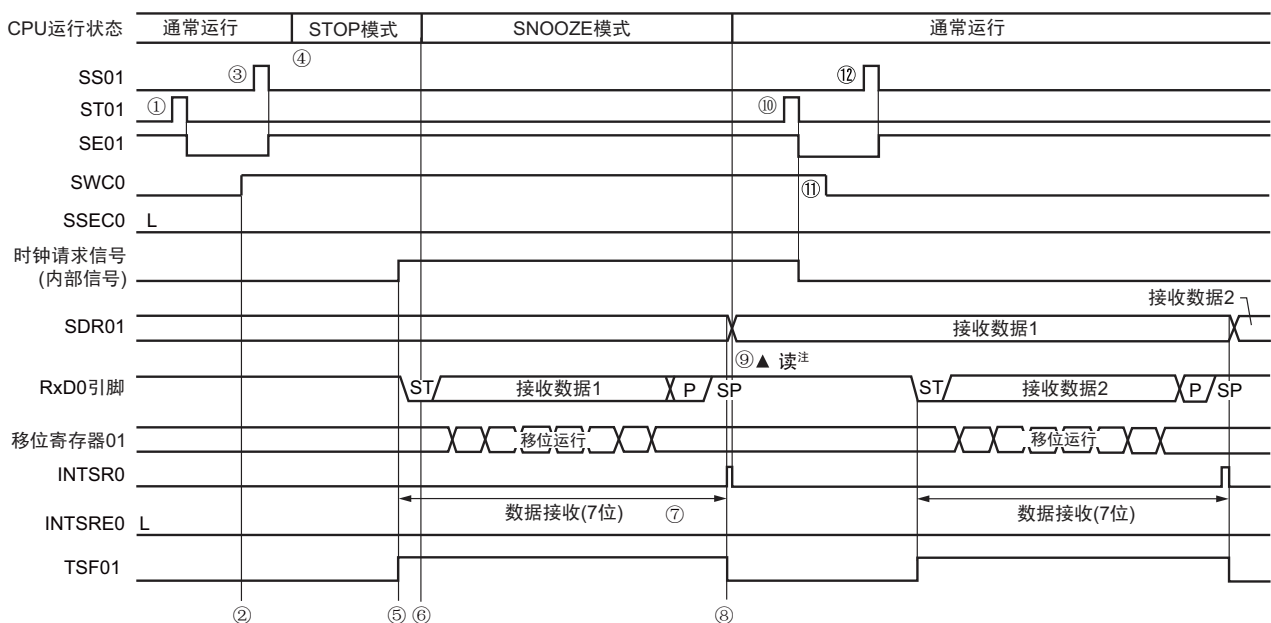
图 12-89 SNOOZE 模式运行（通常运行）的时序图
