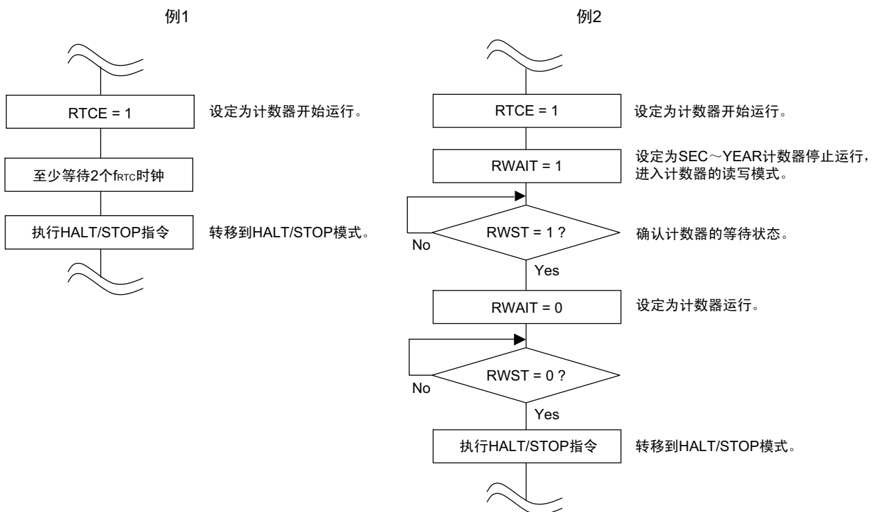
图 7-18 将 RTCE 位置“1”后的 HALT/STOP 模式的转移步骤
