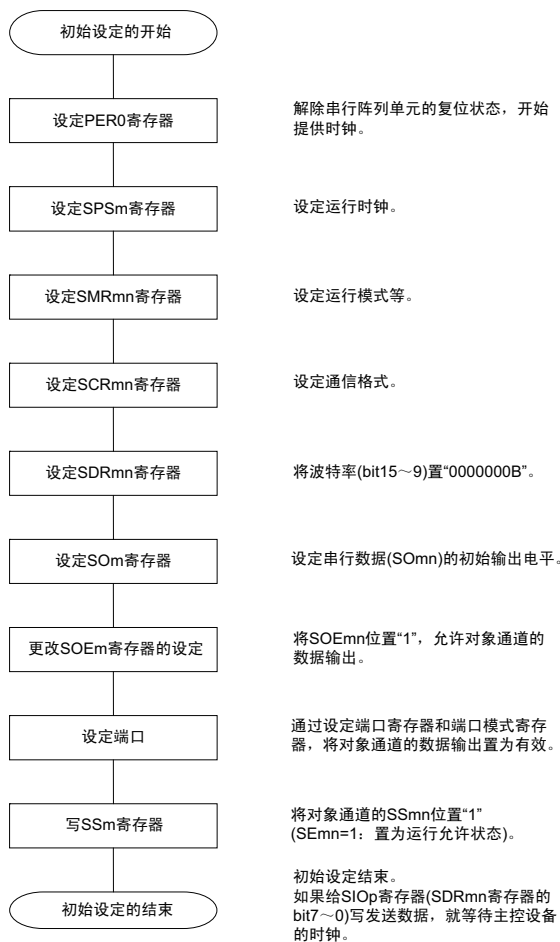
图 12-63 从属发送和接收的初始设定步骤
