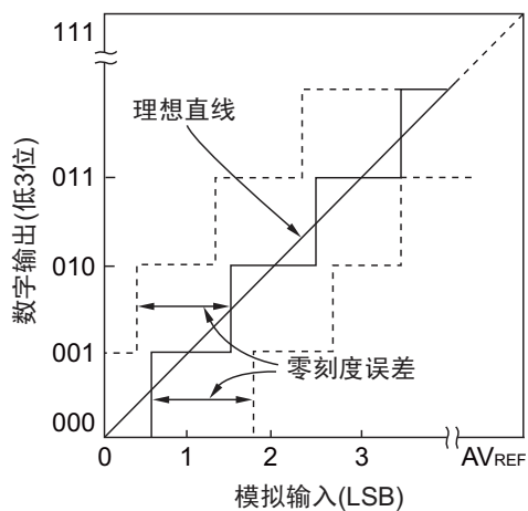
图 11-37 零刻度误差
