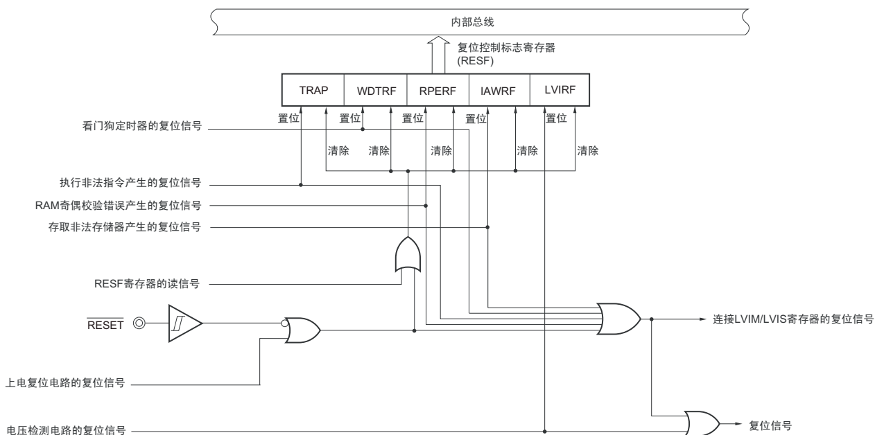
图 20-1 复位功能的框图
