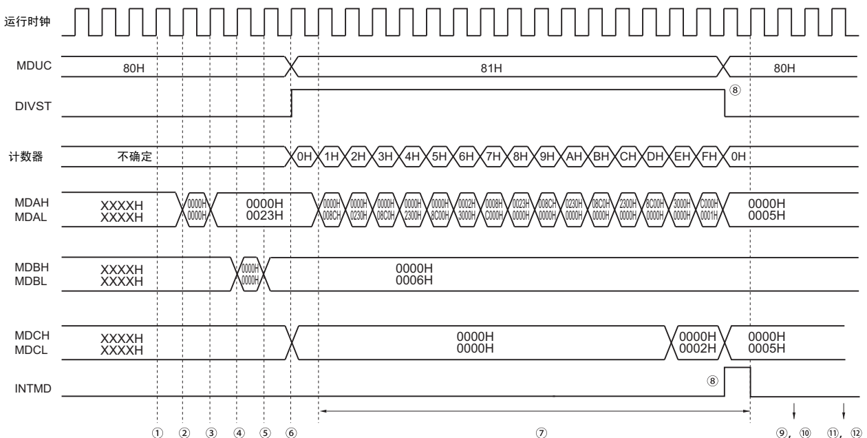
图 15-10 除法运算 (带符号) 的时序图 (35÷6=5 余数 5)
