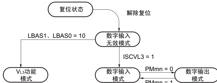
图 14-10 V_{L3} /P125 引脚功能的状态转移图
