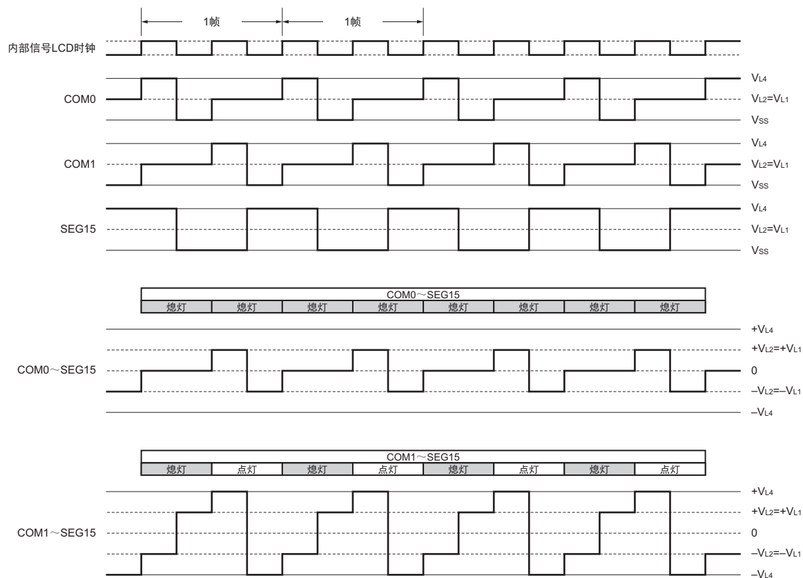
图 14-34 SEG15 和各公共信号之间的 2 个时间片的 LCD 驱动波形例子（1/2 偏压法）
