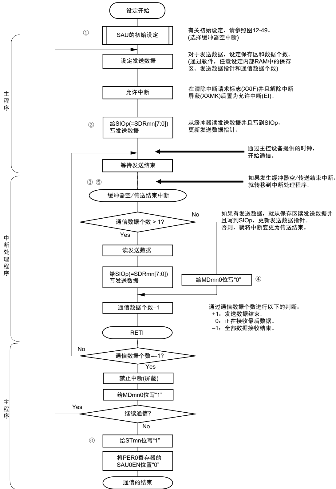
图 12-55 从属发送（连续发送模式）的流程图
