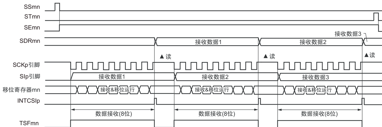
图 12-60 从属接收（单次接收模式）的时序图（类型 1：DAPmn=0、CKPmn=0）
