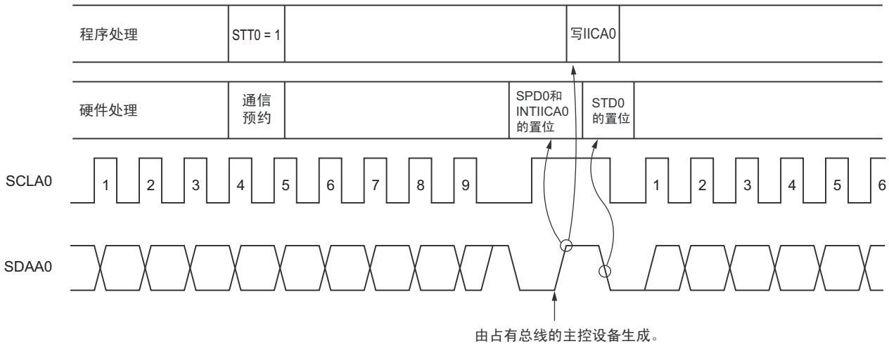
图 13-25 通信预约时序
