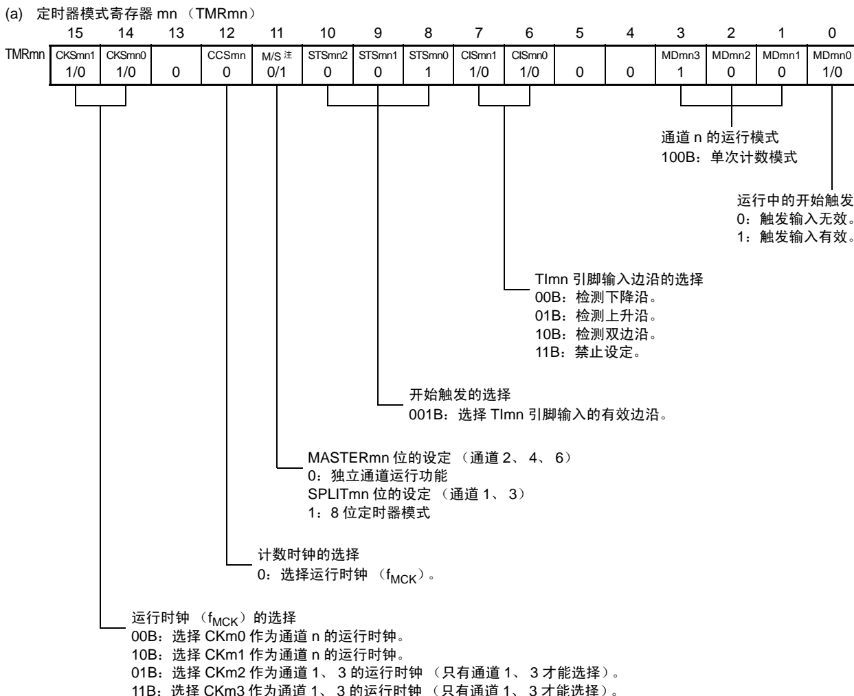
图 6-65 延迟计数器功能时的寄存器设定内容例子
