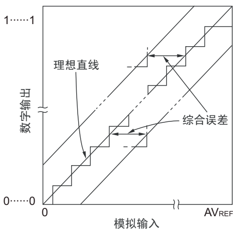
图 11-35 综合误差
