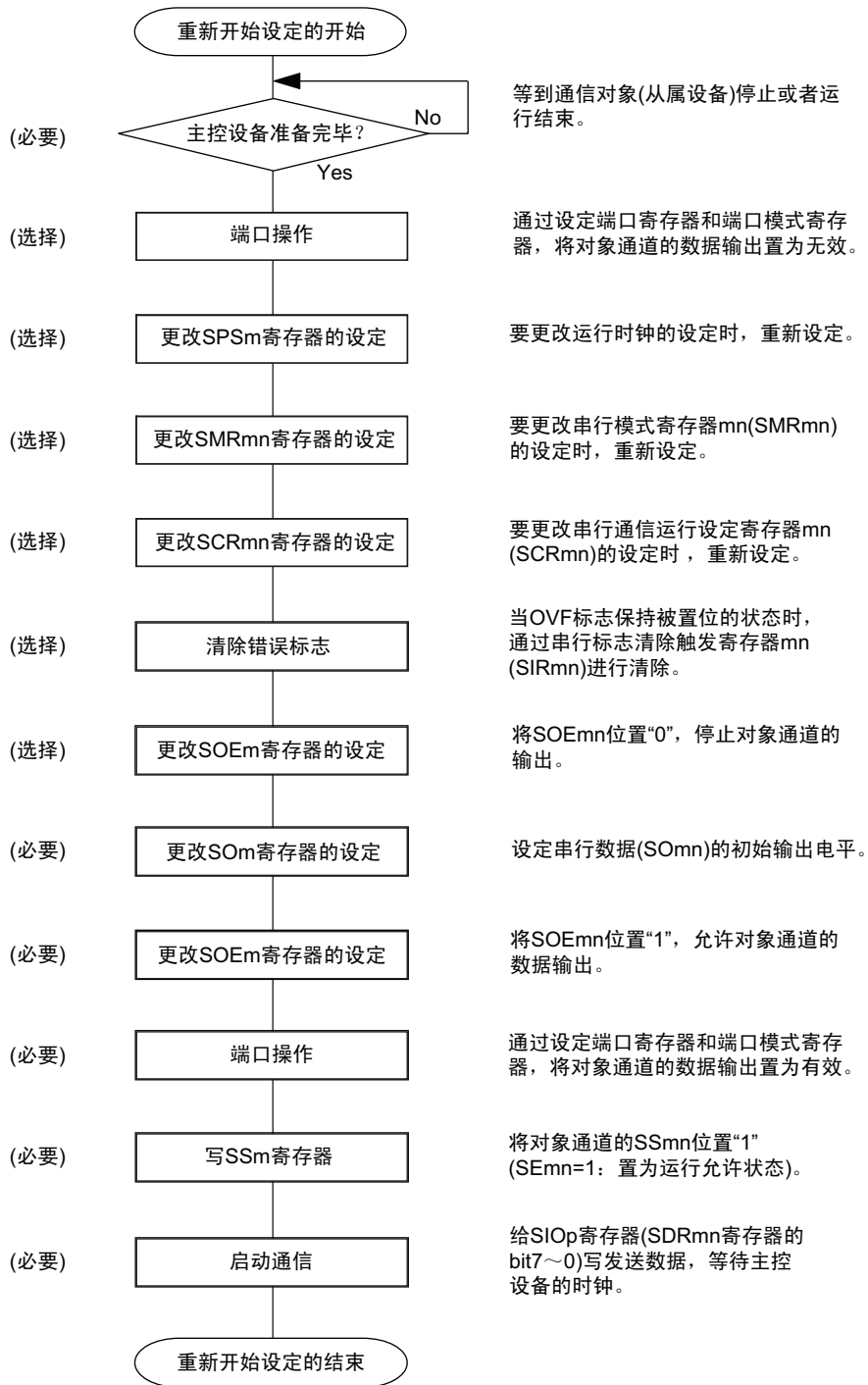
图 12-51 从属发送的重新开始设定步骤
