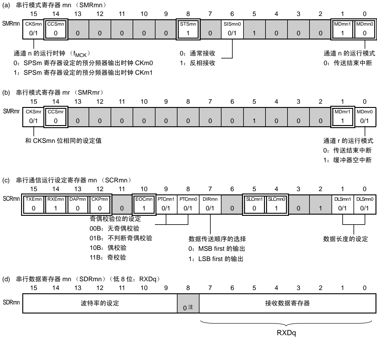
图 12-83 UART (UART0) 的 UART 接收时的寄存器设定内容例子 (1/2)
