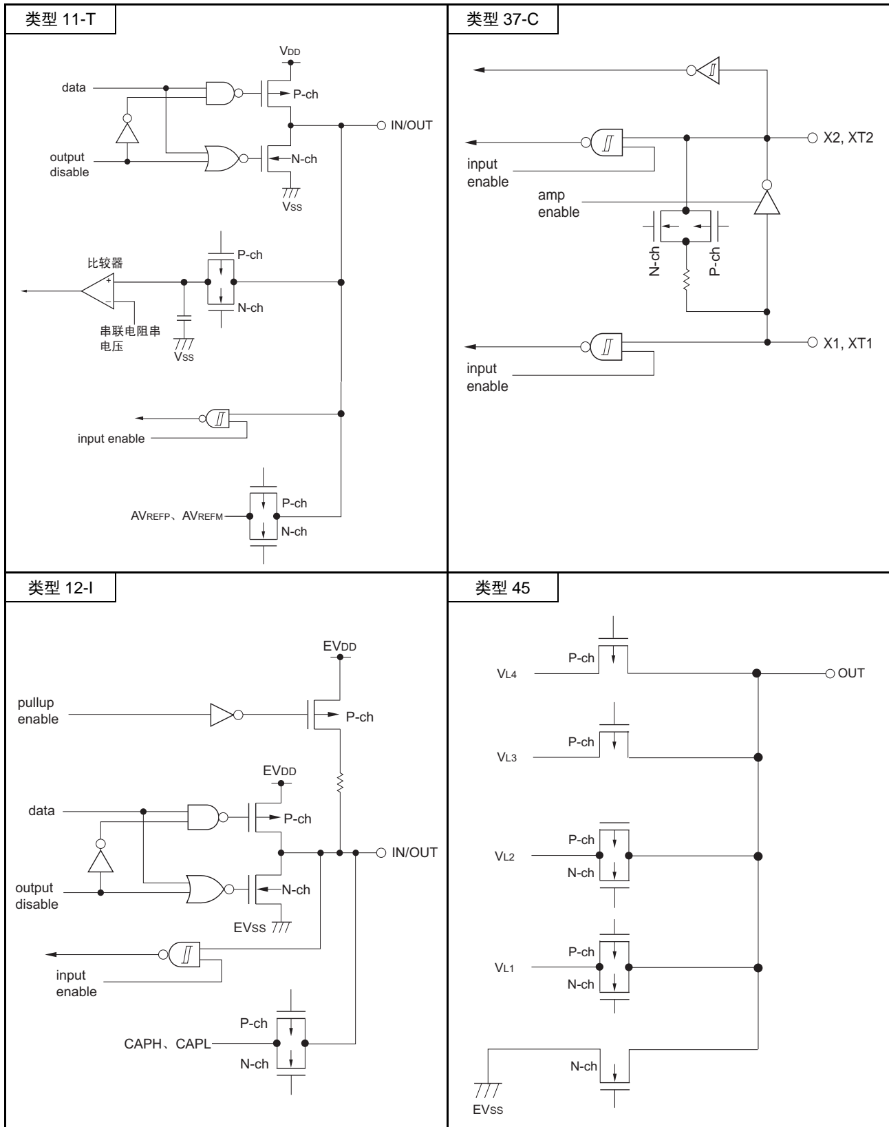
图 2-1 引脚的输入 / 输出电路一览表 (2/4)
