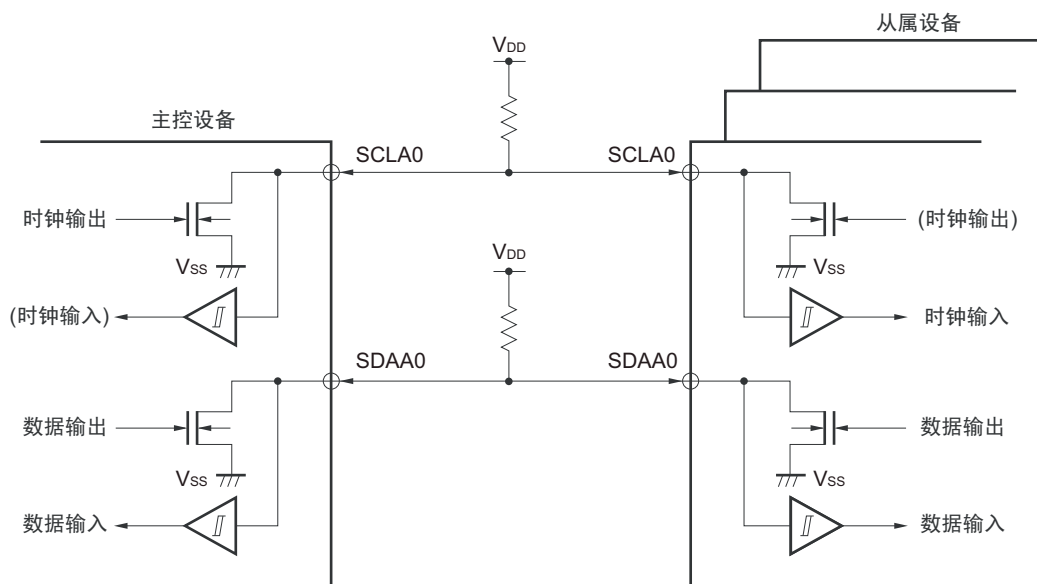
图 13-13 引脚结构图
