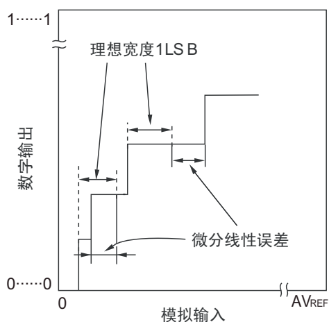
图 11-40 微分线性误差
