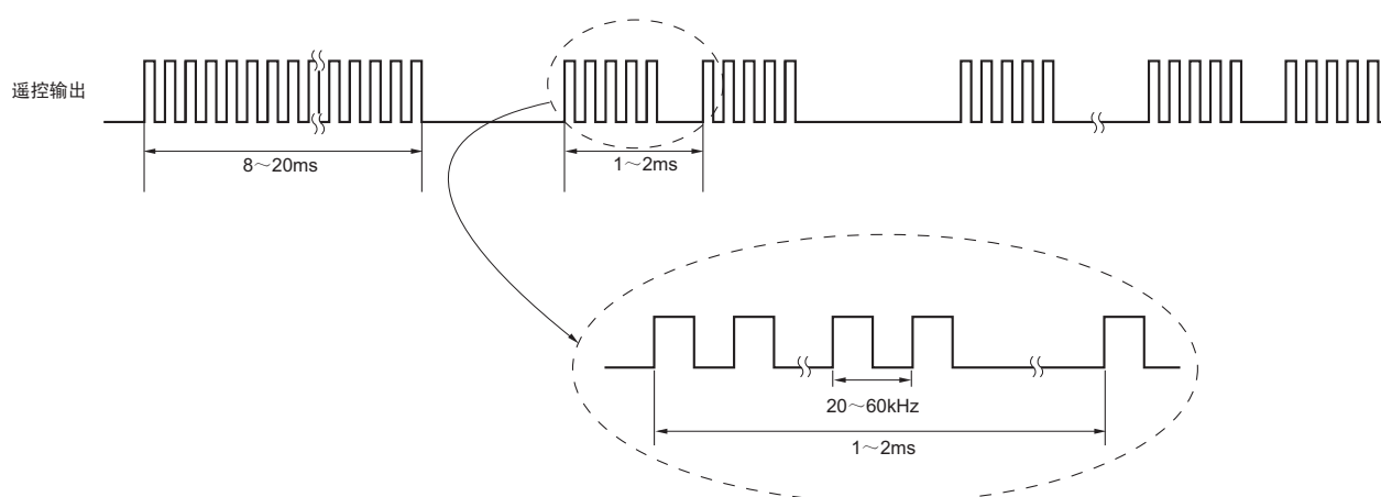
图 6-82 遥控输出
