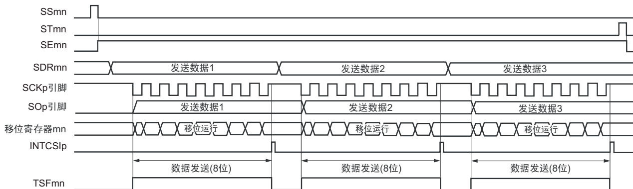
图 12-52 从属发送 (单次发送模式) 的时序图 (类型 1: DAPmn=0、CKPmn=0)
