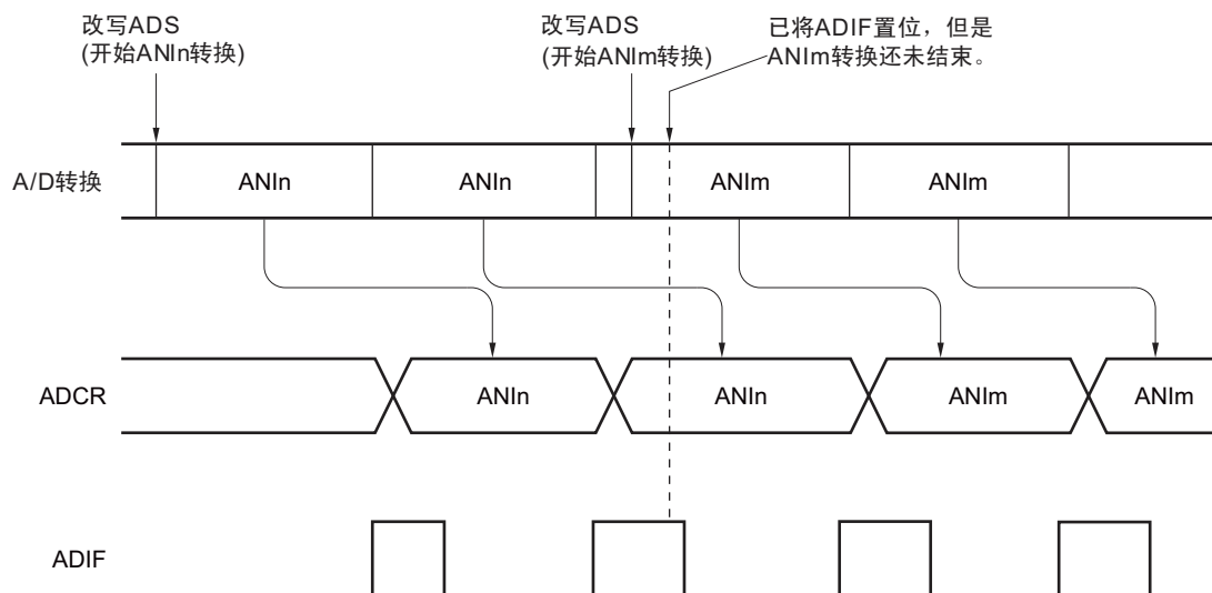
图 11-42 A/D 转换结束中断请求的产生时序
