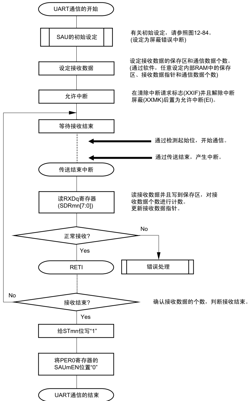
图 12-88 UART 接收的流程图
