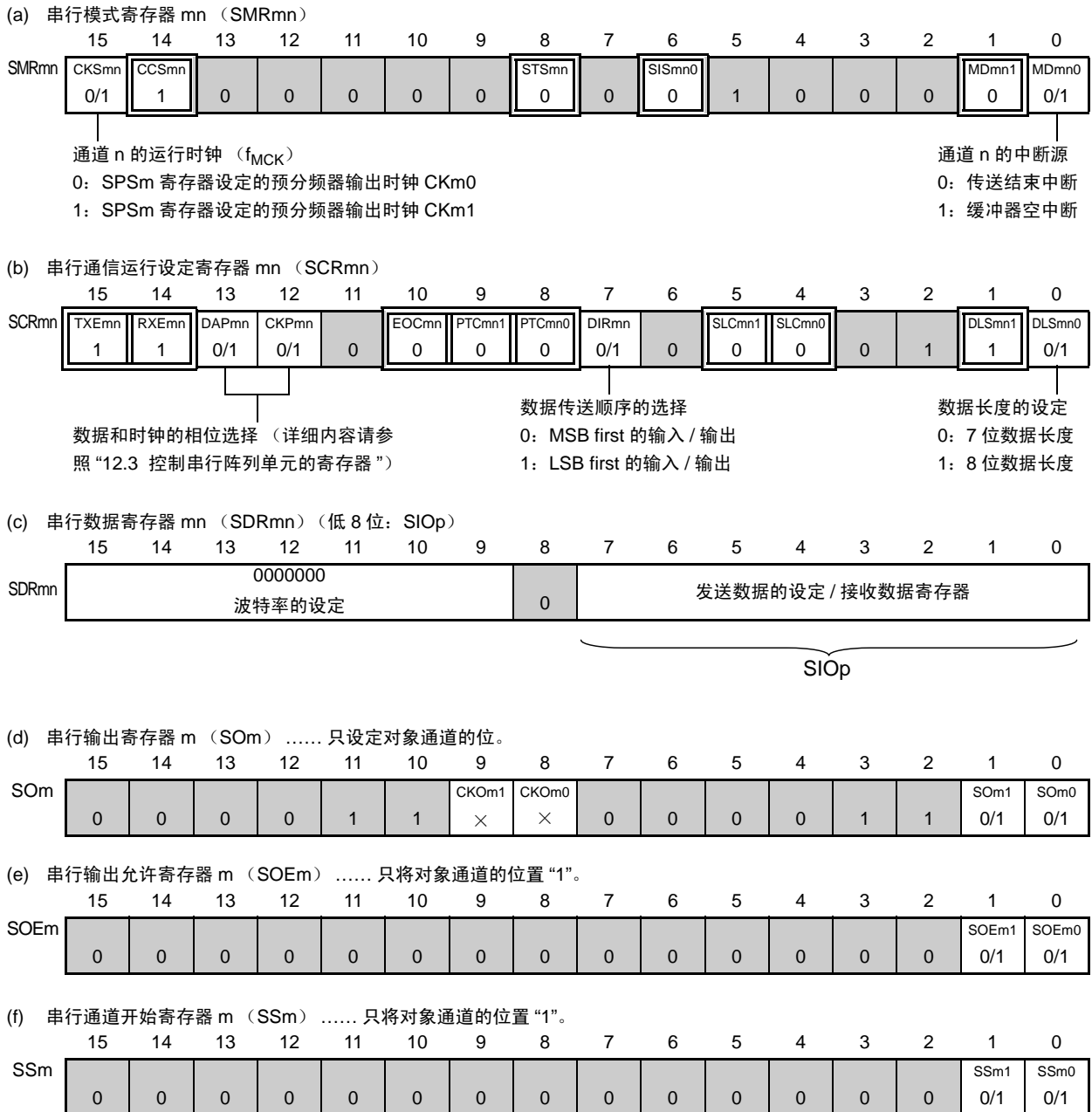
图 12-62 3 线串行 I/O (CSI00、CSI01) 从属发送和接收时的寄存器设定内容例子
